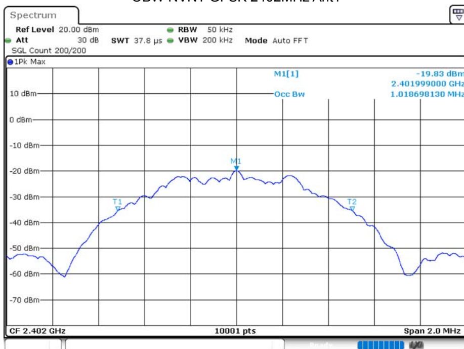
OBW NVNT GFSK 2402MHz Ant1
