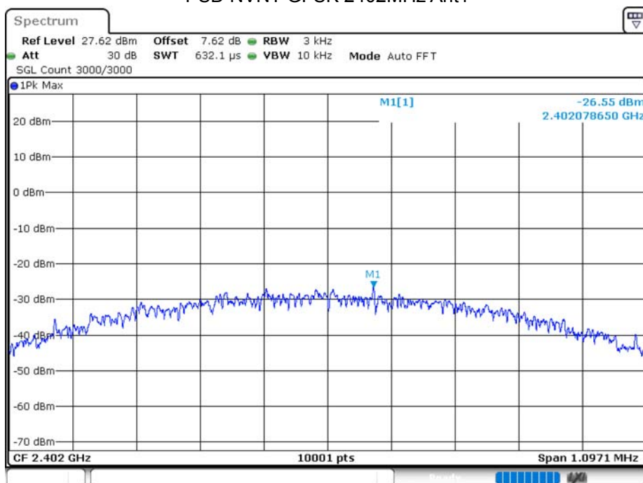
PSD NVNT GFSK 2402MHz Ant1
