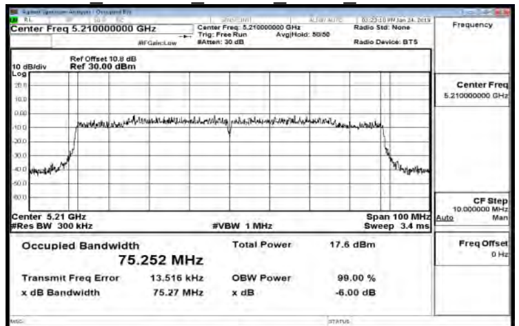
IC 802.11ac 80MHz AUX1 5210MHz
