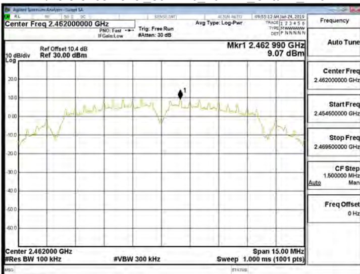
WLAN\Reference Level_802.11b_20MHz_Chain1_2462MHz
