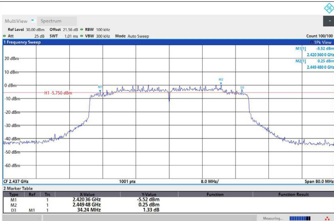
11AX40MIMO-Ant1-2437-PASS
