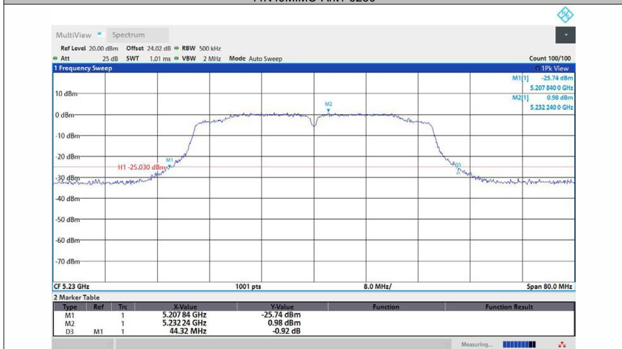
11N40MIMO-Ant2-5230
