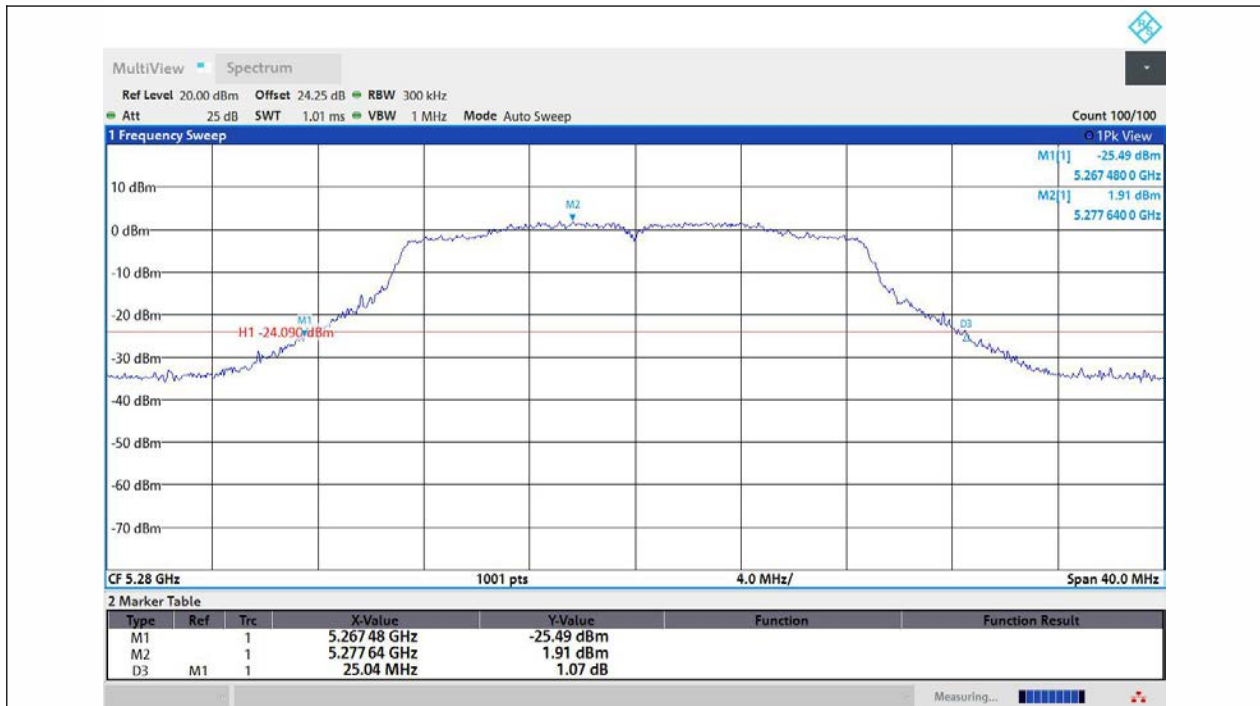
11AC20MIMO-Ant1-5280
