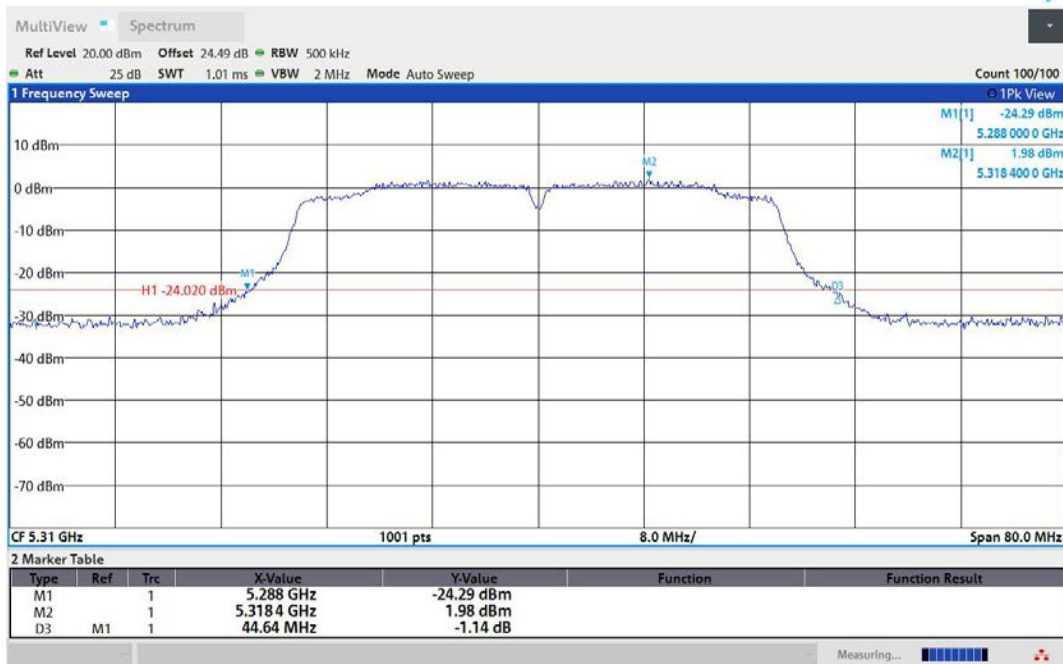
11N40MIMO-Ant1-5310
