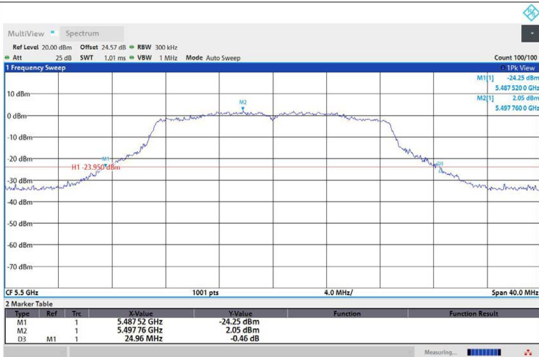
11N20MIMO-Ant1-5500
