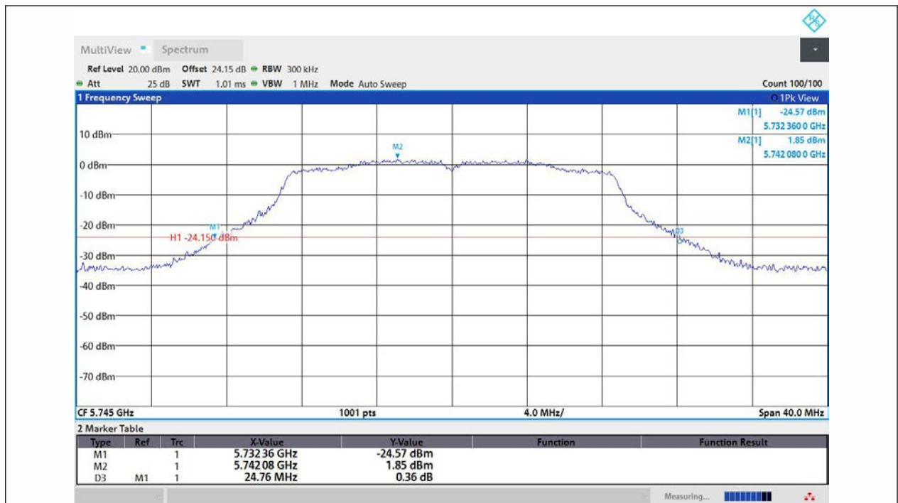
11N20MIMO-Ant1-5745
