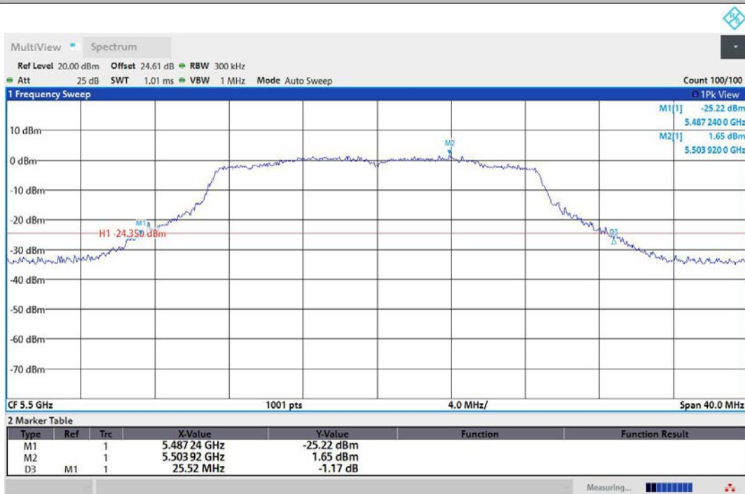
11N20MIMO-Ant2-5500
