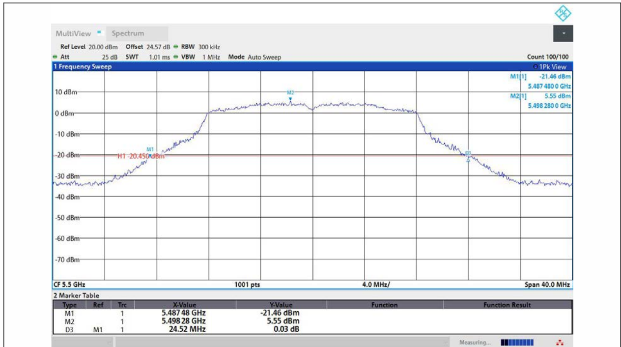
11A-Ant1-5500
