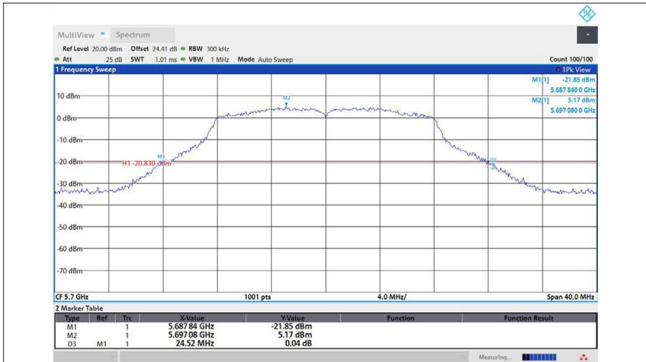
11A-Ant1-5700
