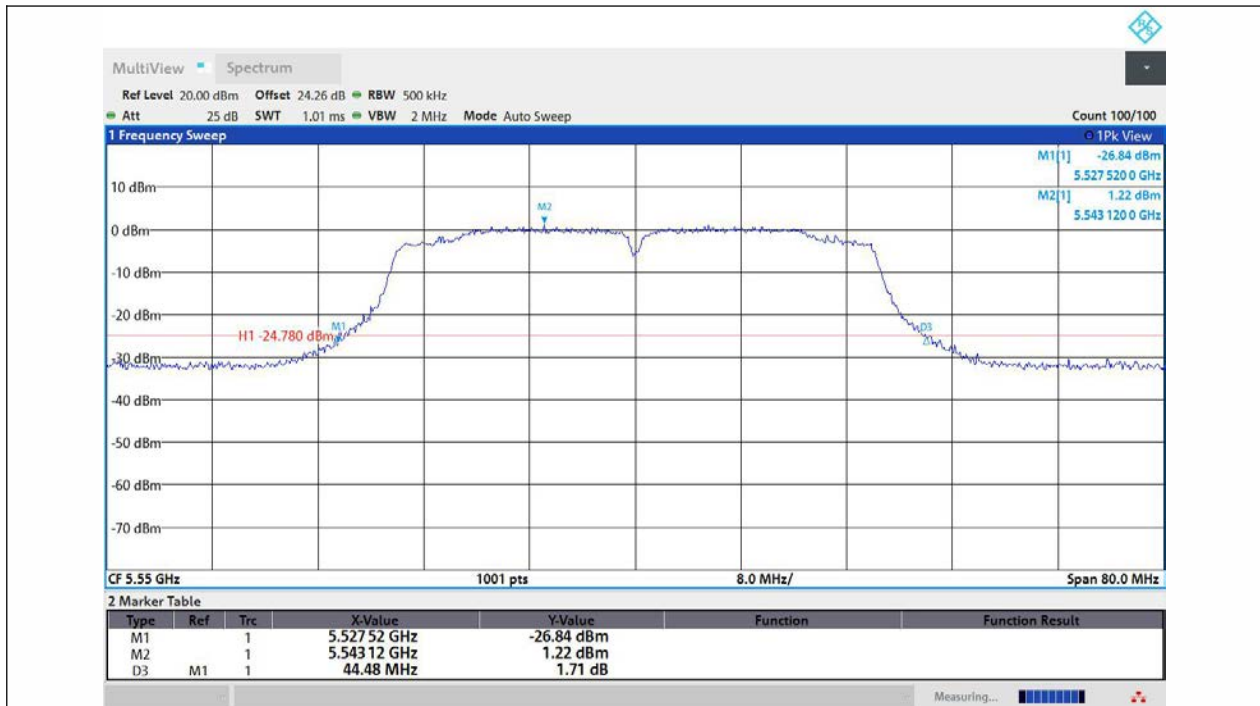
11N40MIMO-Ant1-5550
