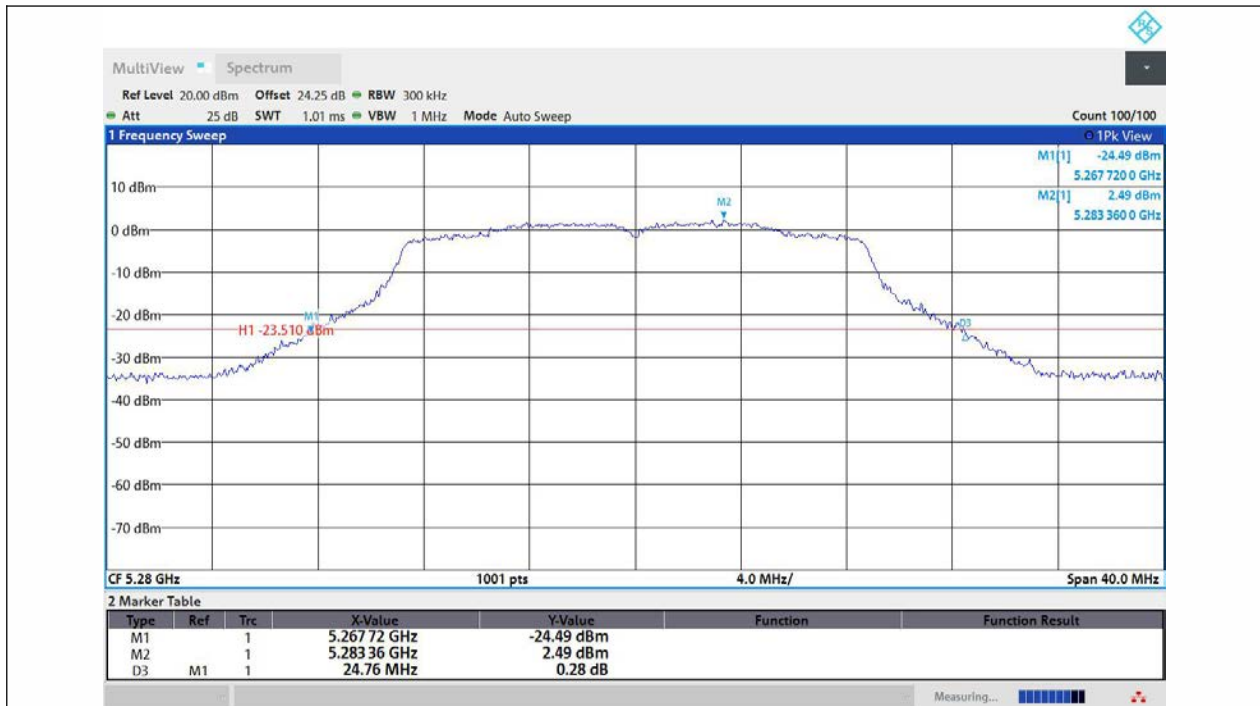
11N20MIMO-Ant1-5280
