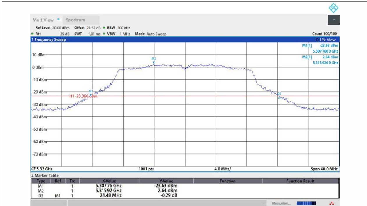
11N20MIMO-Ant1-5320
