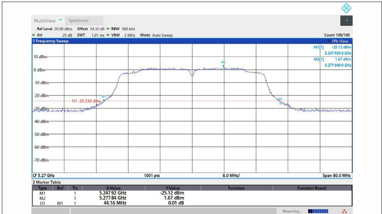
11N40MIMO-Ant1-5270
