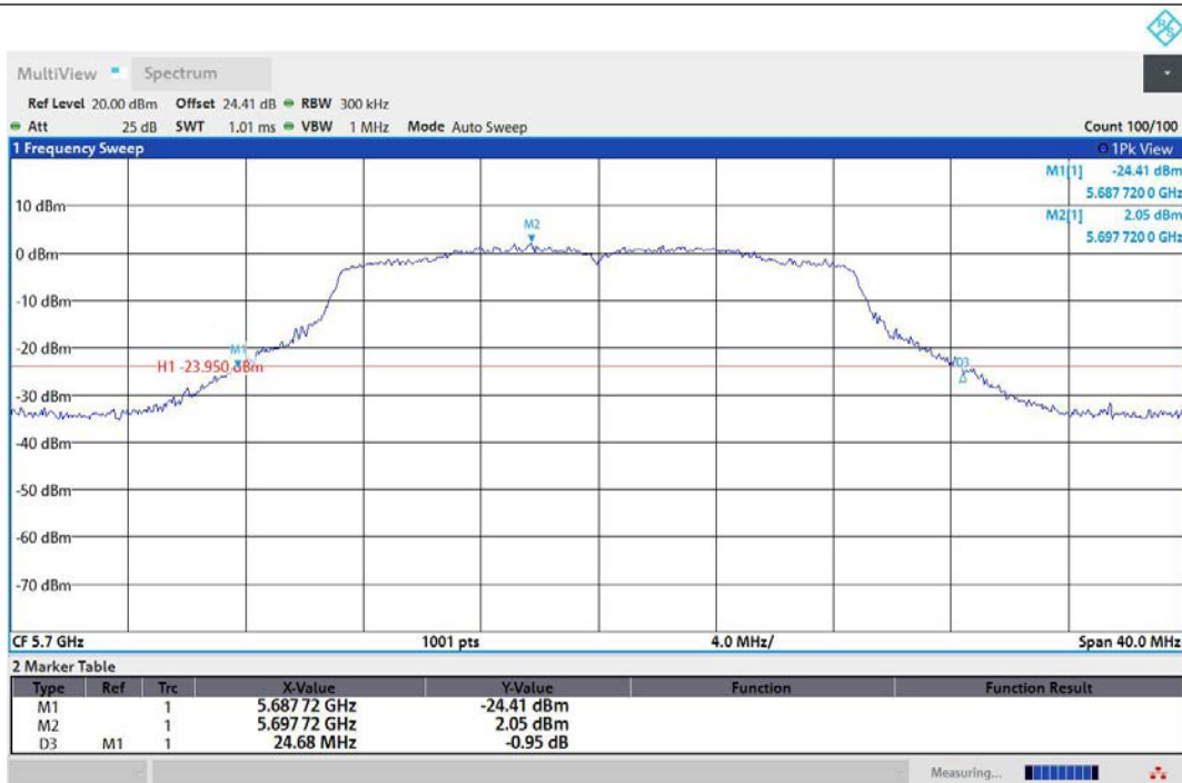
11N20MIMO-Ant1-5700
