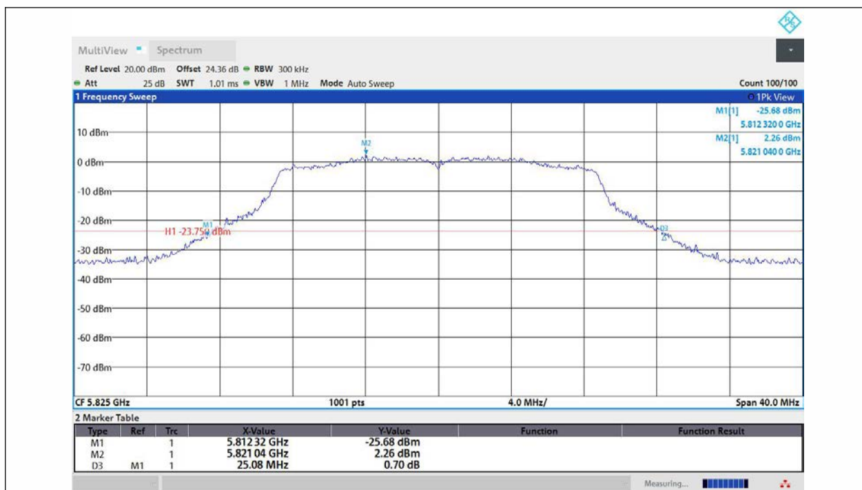
11N20MIMO-Ant1-5825
