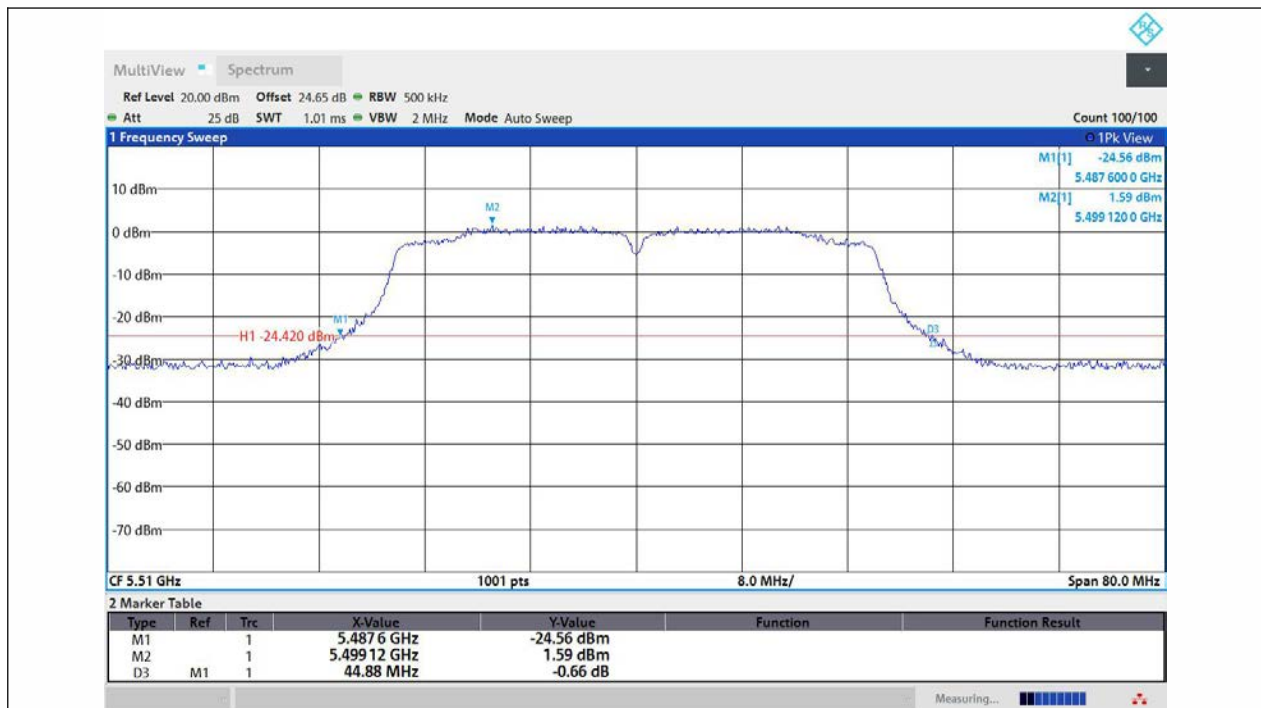
11N40MIMO-Ant1-5510
