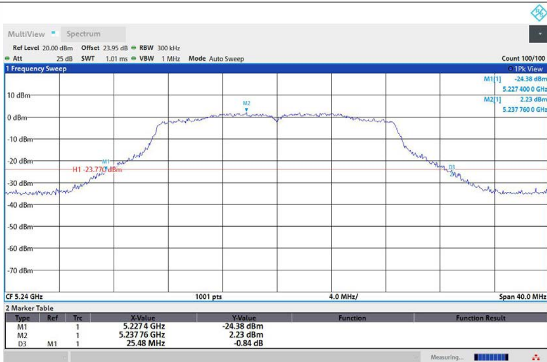
11N20MIMO-Ant1-5240
