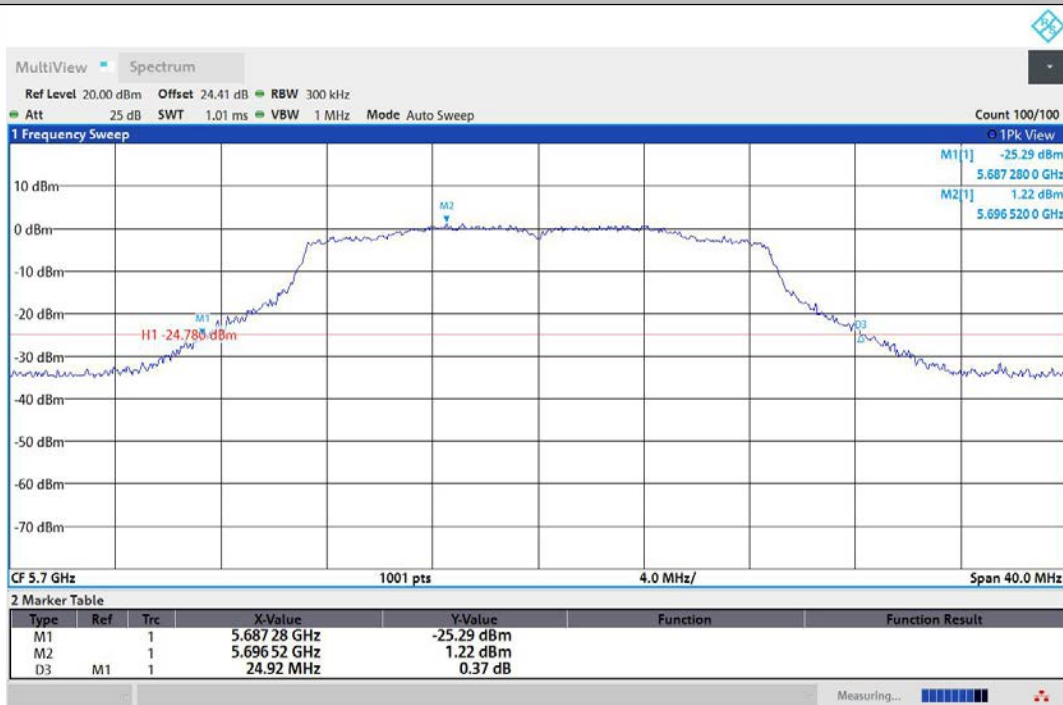
11N20MIMO-Ant2-5700
