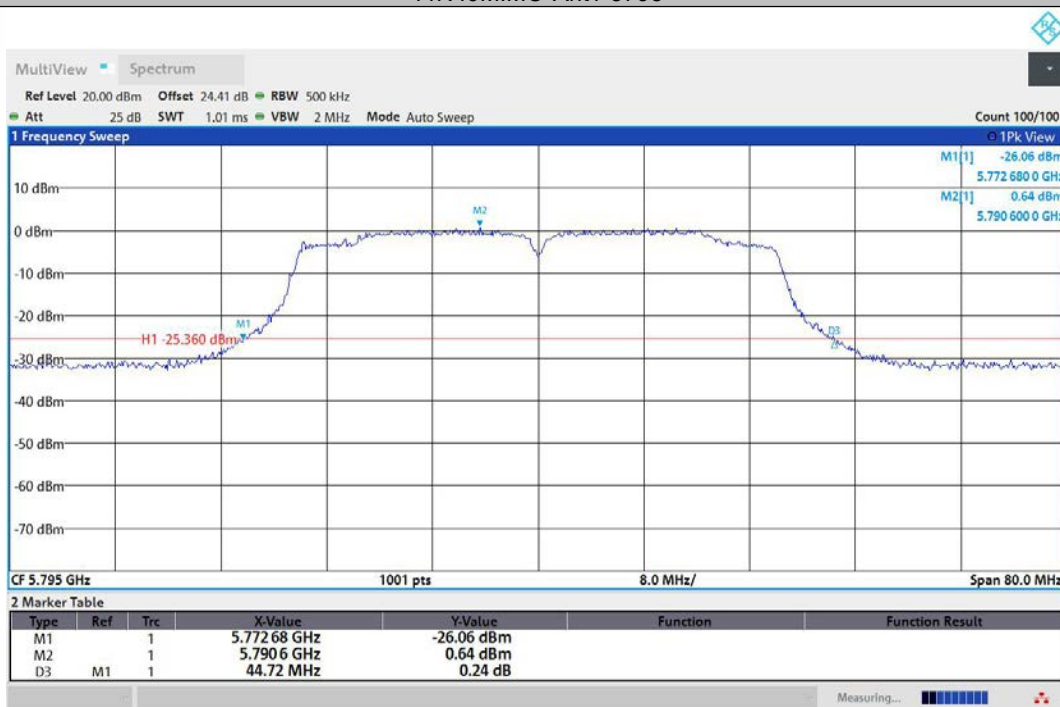
11N40MIMO-Ant2-5795
