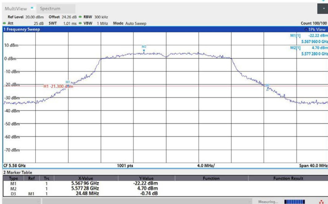
11A-Ant1-5580
