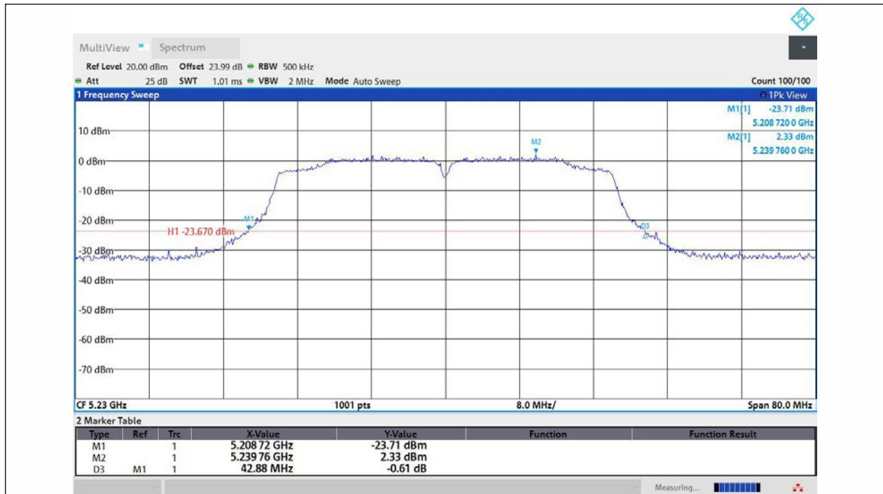
11N40MIMO-Ant1-5230
