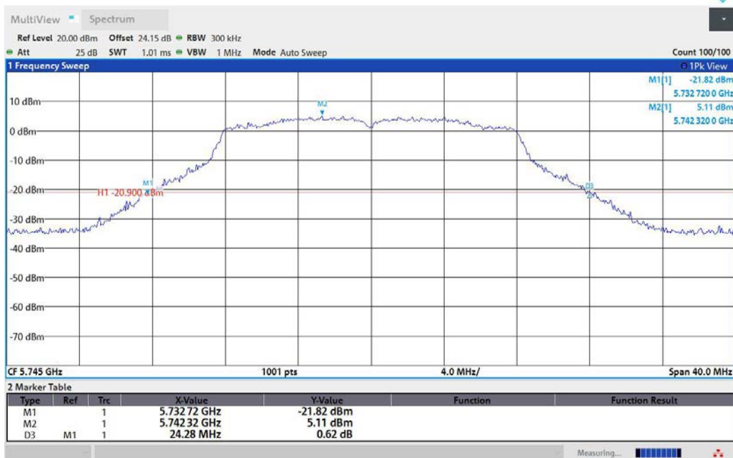
11A-Ant1-5745
