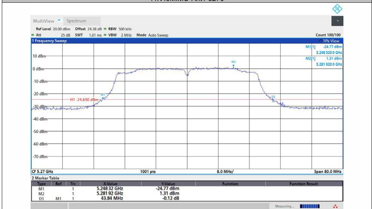
11N40MIMO-Ant2-5270
