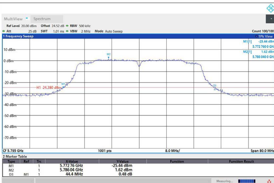
11N40MIMO-Ant1-5795
