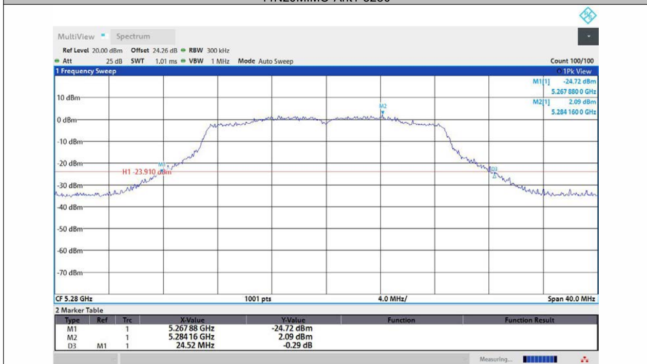
11N20MIMO-Ant2-5280
