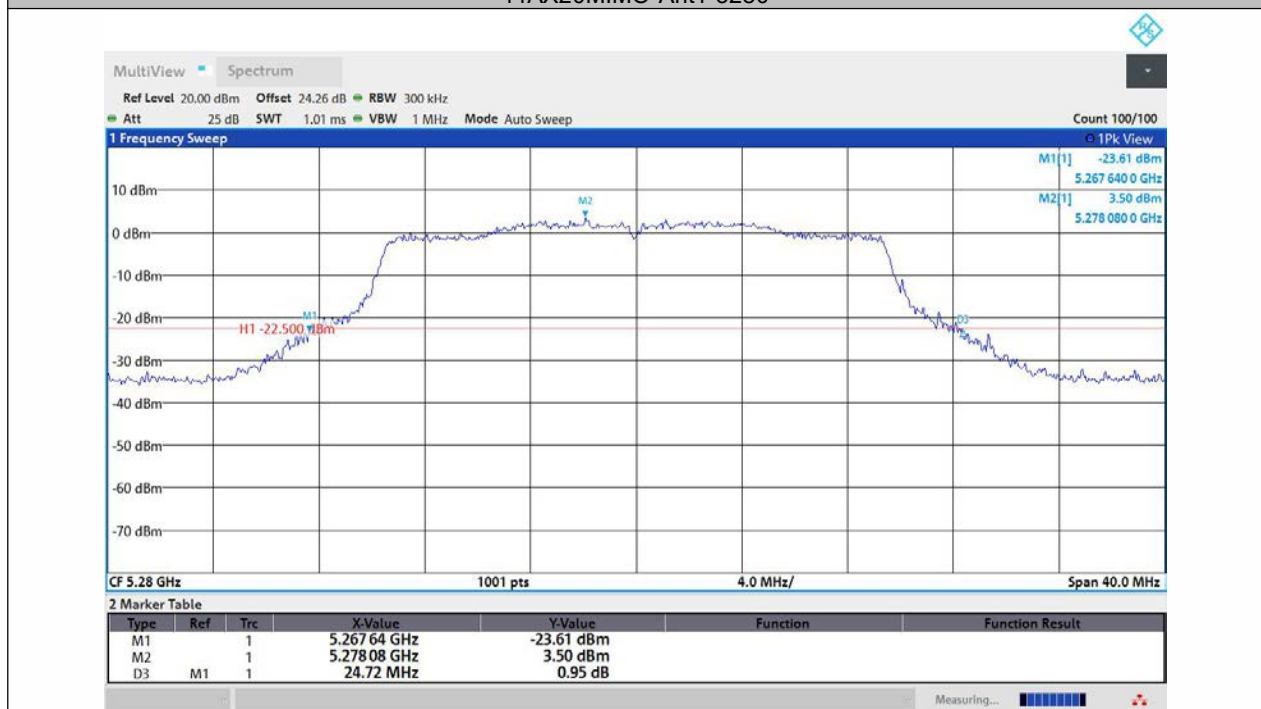
11AX20MIMO-Ant2-5280
