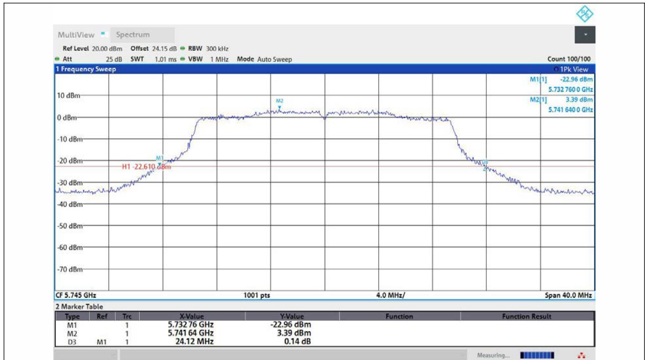
11AX20MIMO-Ant1-5745
