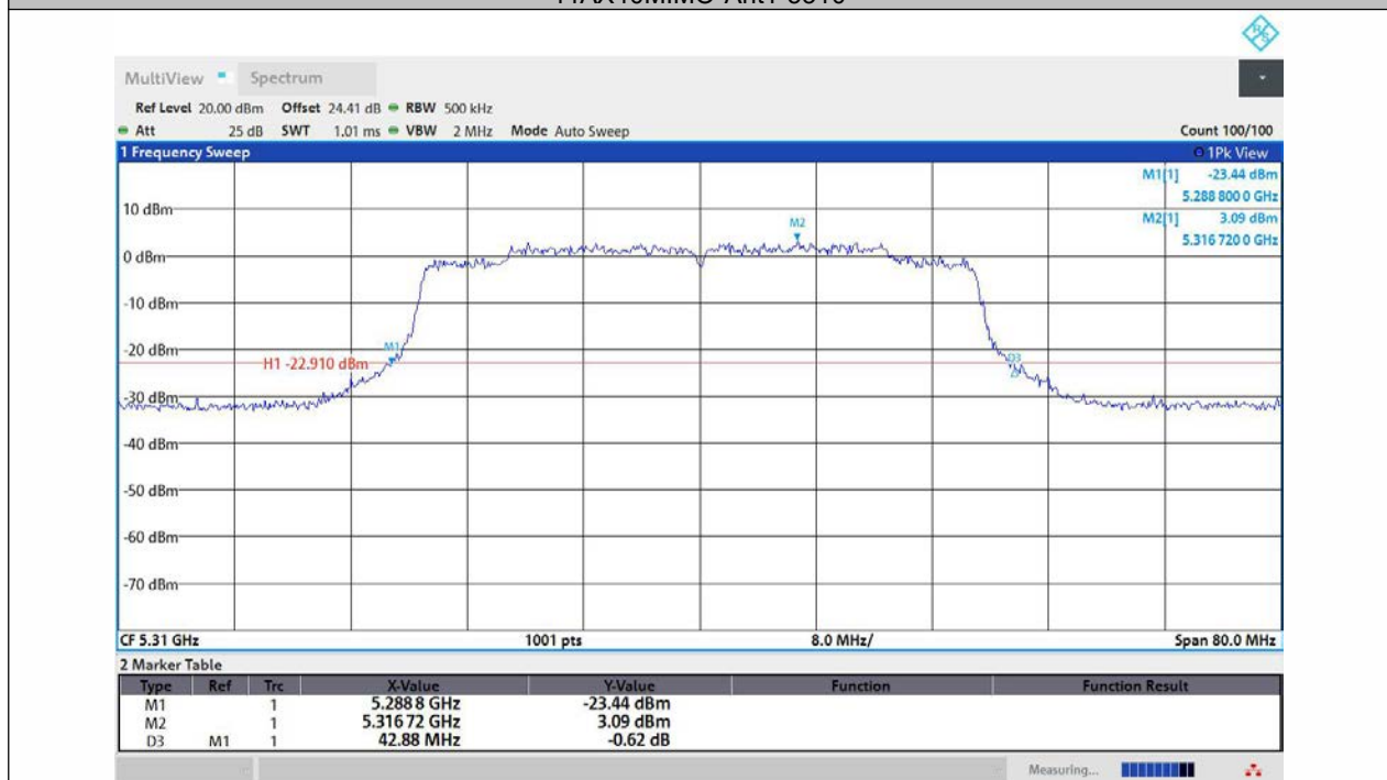
11AX40MIMO-Ant2-5310
