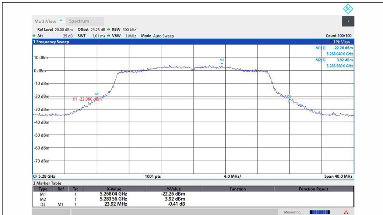
11AX20MIMO-Ant1-5280
