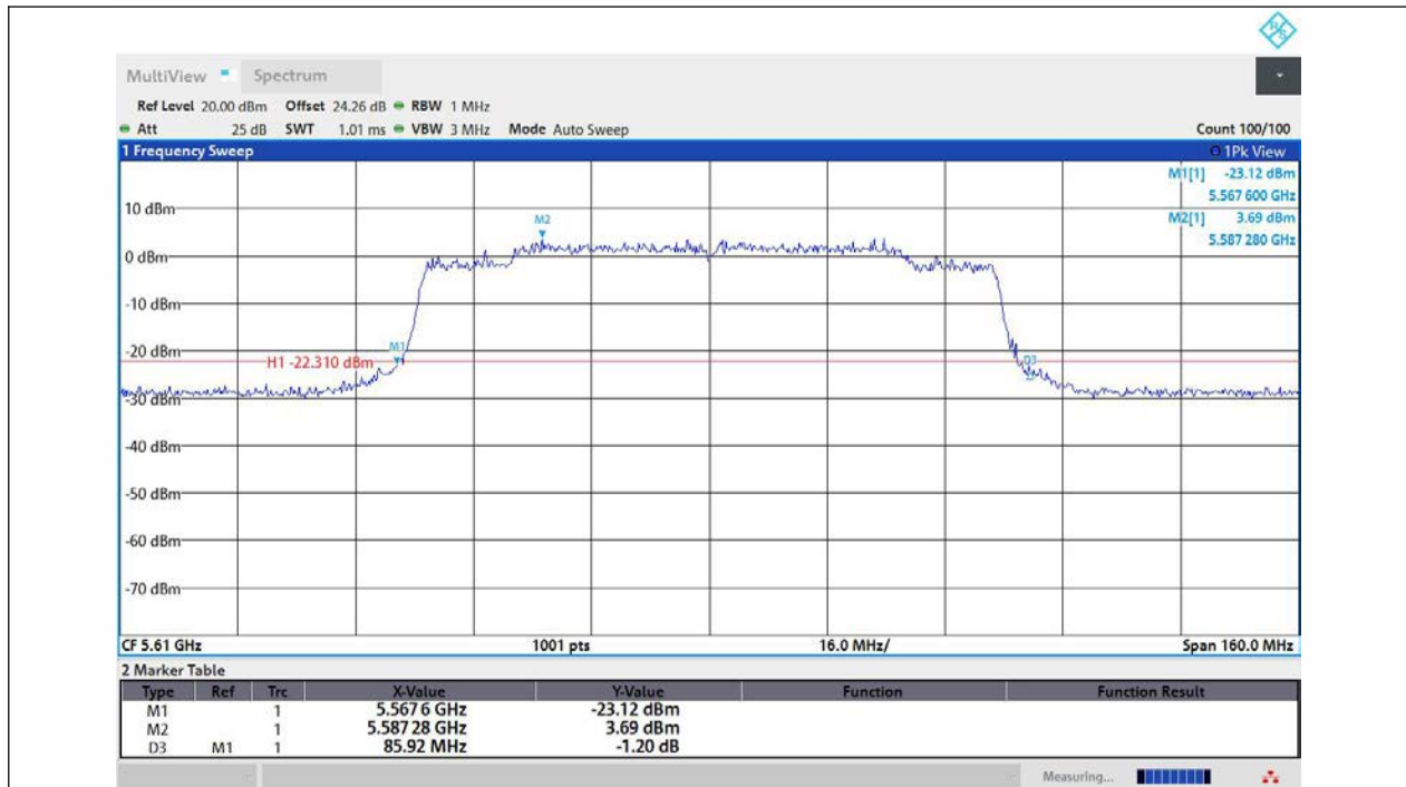
11AX80MIMO-Ant1-5610
