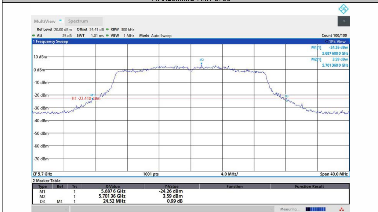
11AX20MIMO-Ant2-5700
