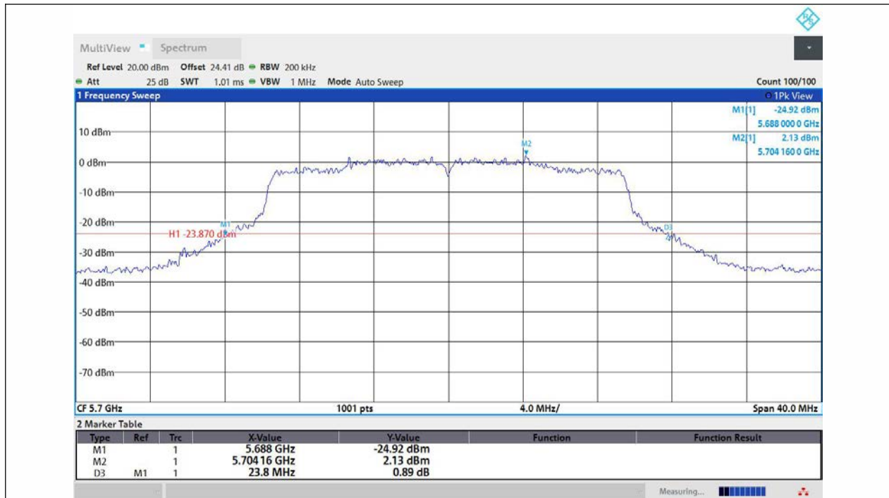
11AX20MIMO-Ant1-5700
