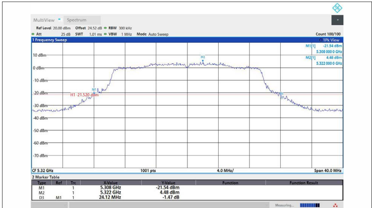
11AX20MIMO-Ant1-5320
