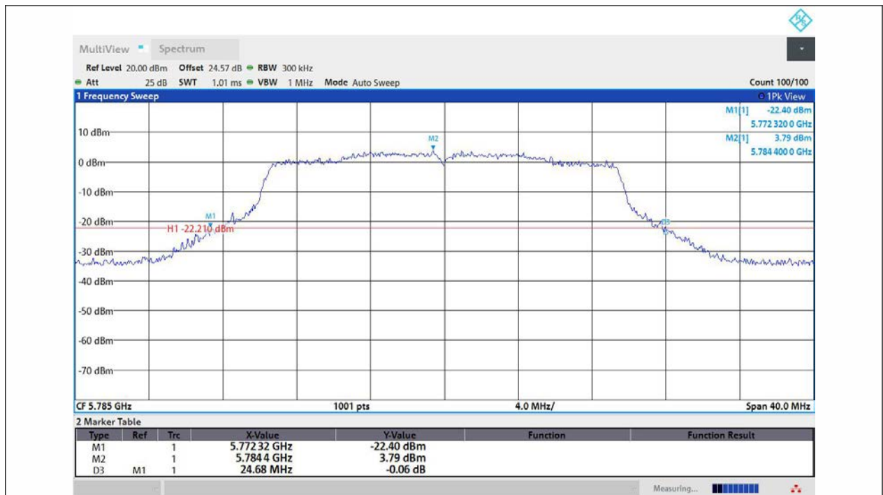
11AX20MIMO-Ant1-5785
