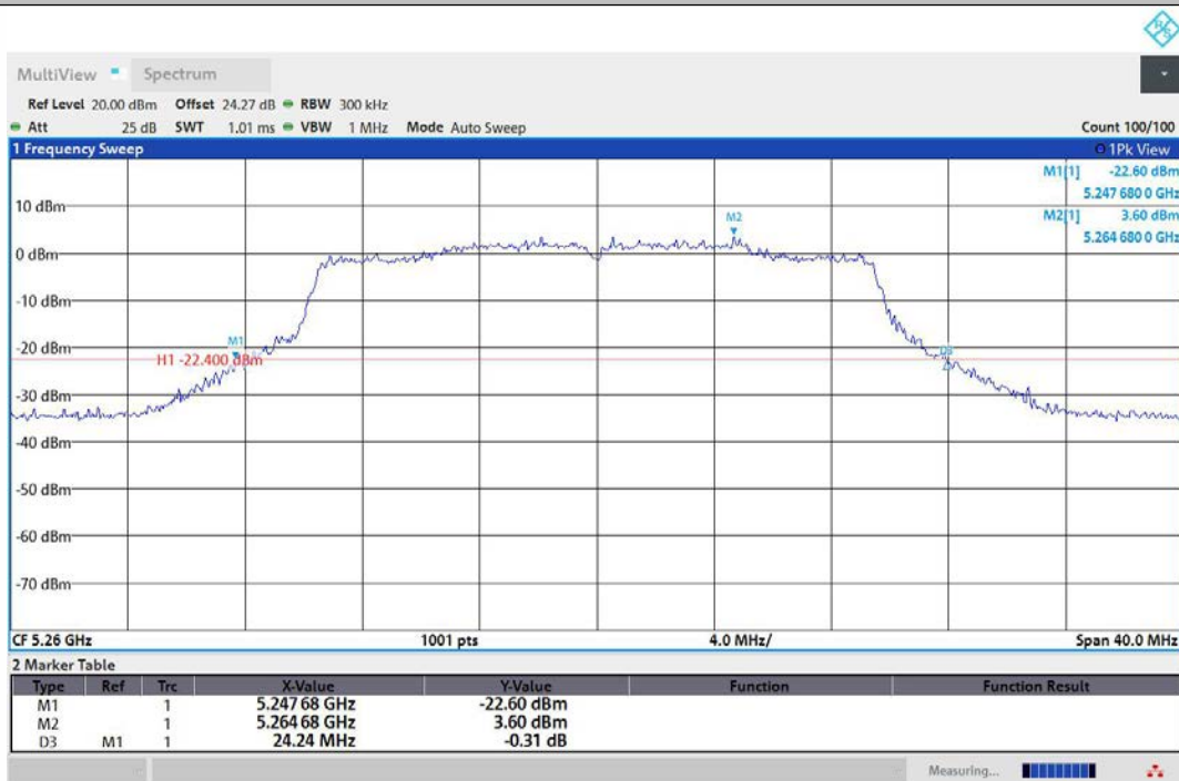
11AX20MIMO-Ant2-5260
