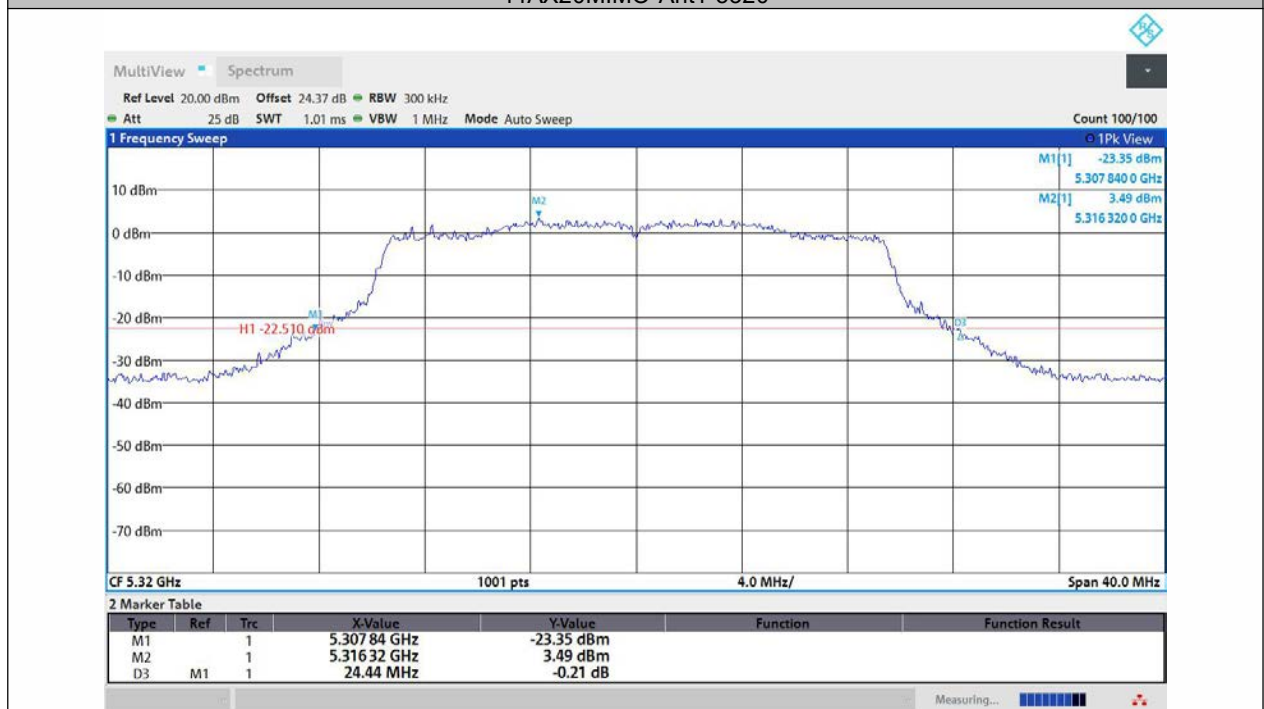
11AX20MIMO-Ant2-5320
