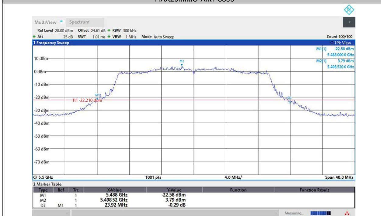
11AX20MIMO-Ant2-5500
