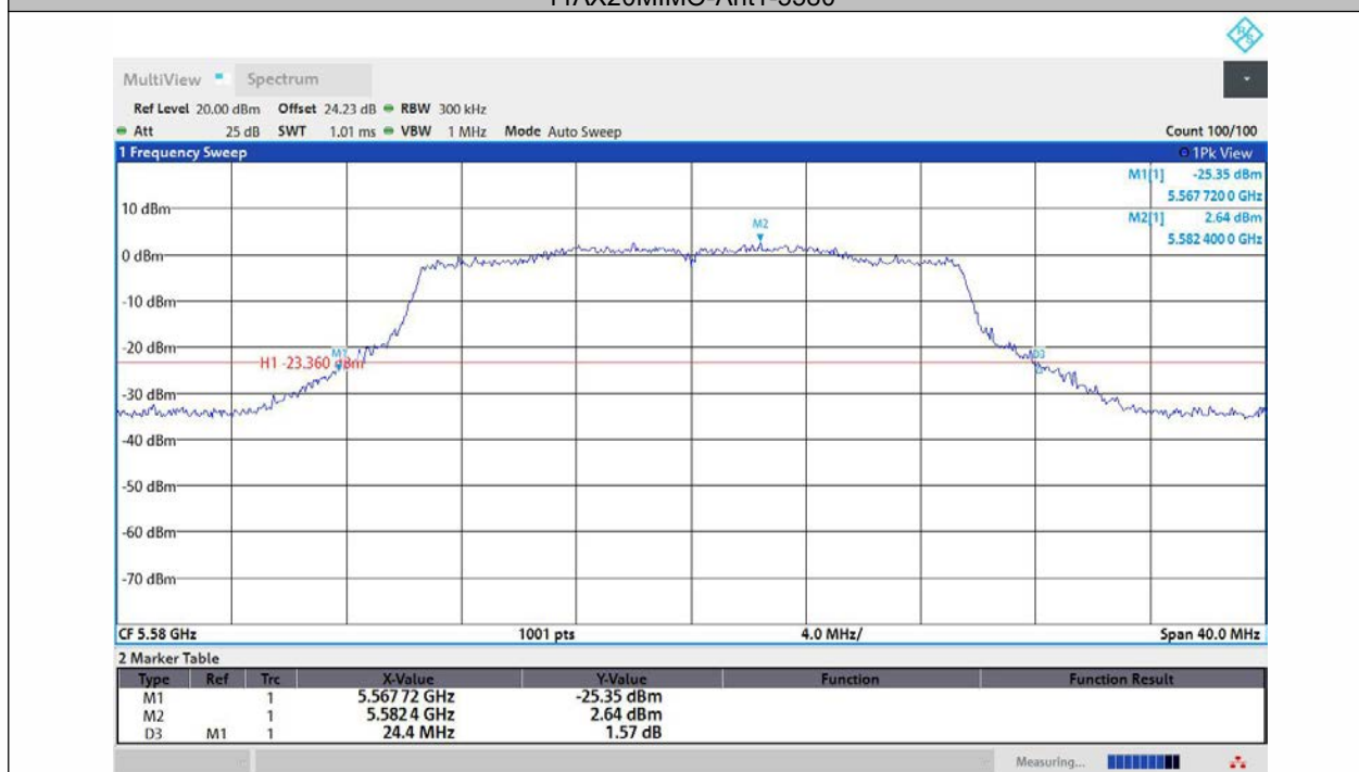
11AX20MIMO-Ant2-5580
