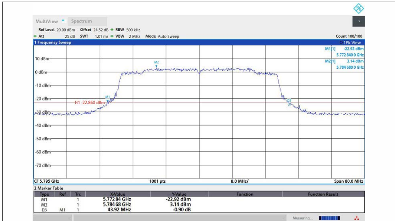
11AX40MIMO-Ant1-5795
