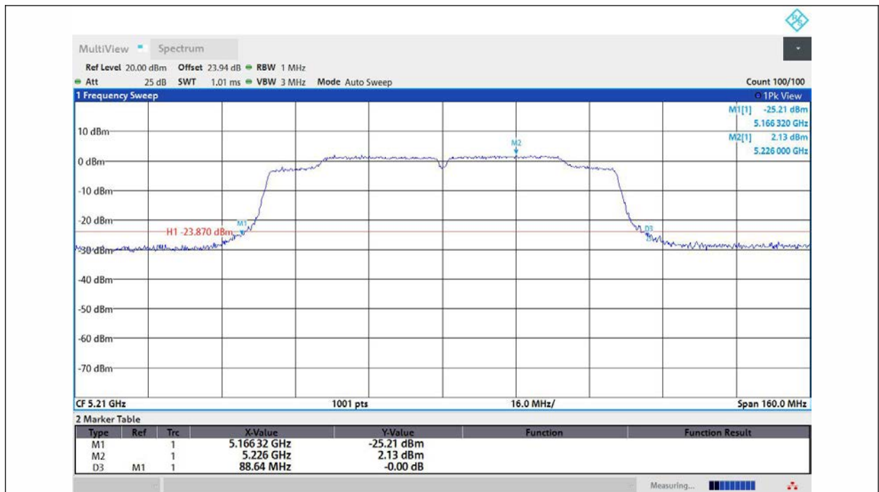
11AC80MIMO-Ant1-5210
