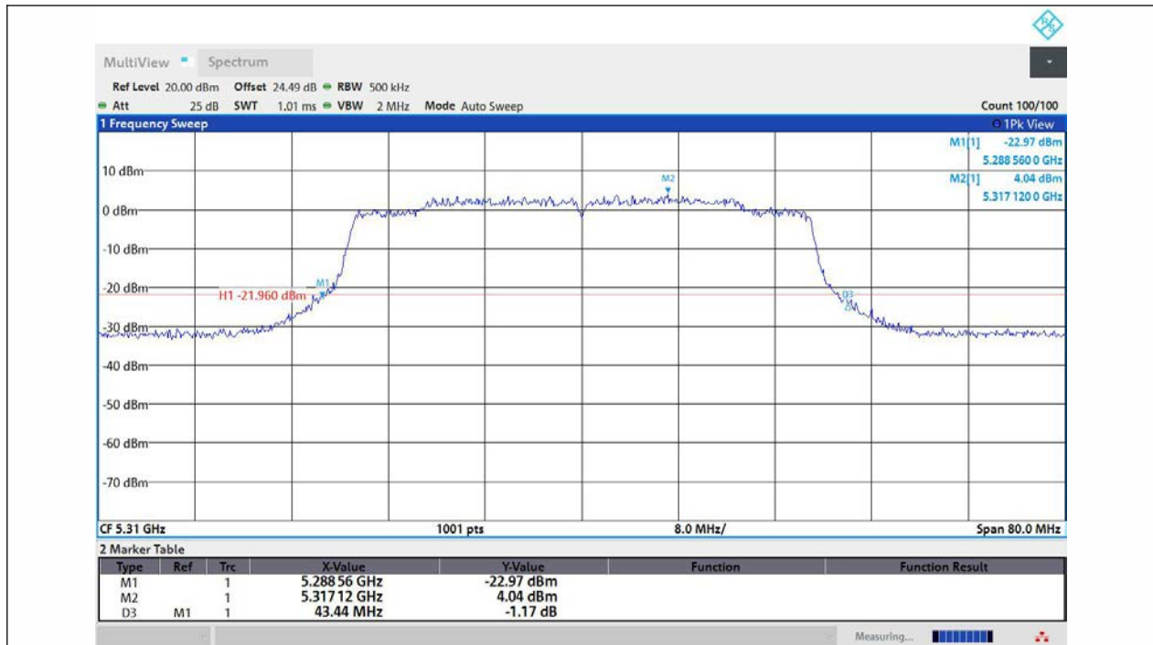
11AX40MIMO-Ant1-5310
