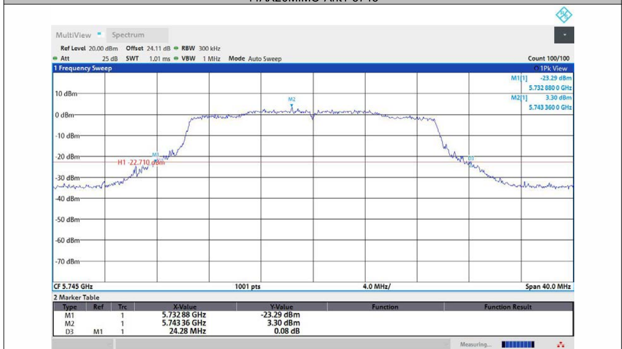
11AX20MIMO-Ant2-5745
