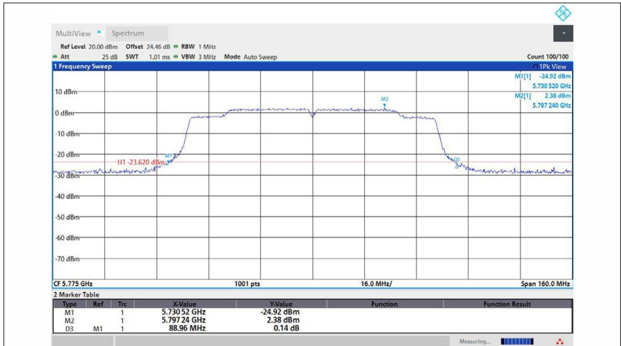
11AC80MIMO-Ant1-5775
