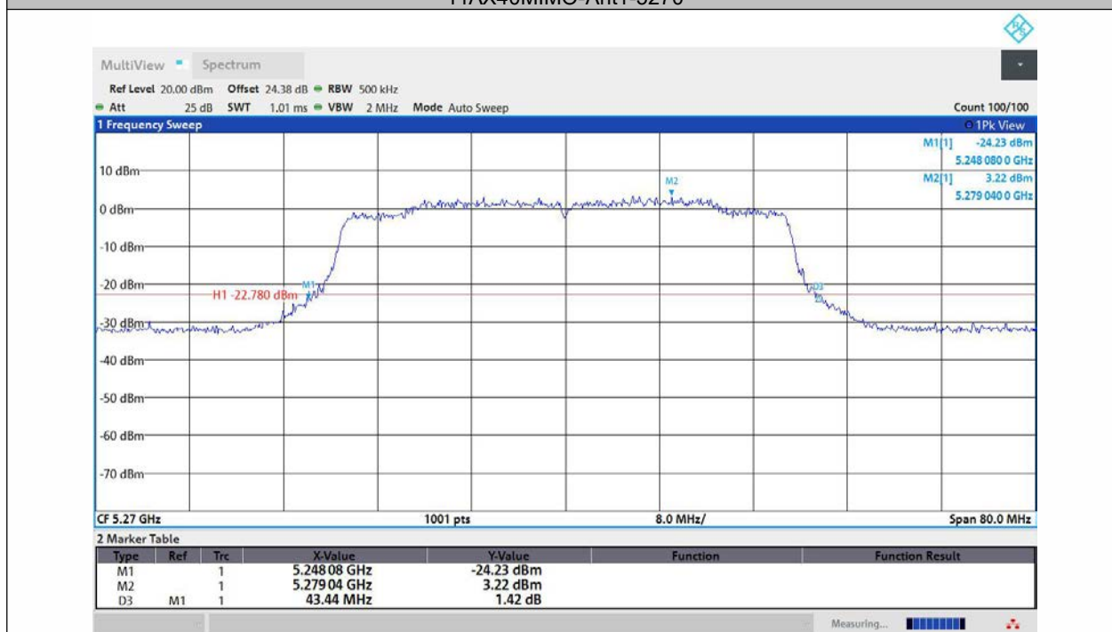
11AX40MIMO-Ant2-5270
