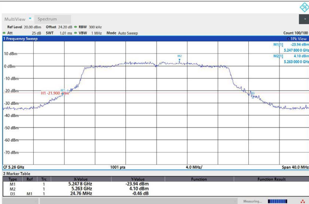
11AX20MIMO-Ant1-5260
