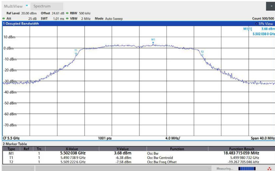
11N20MIMO-Ant2-5500
