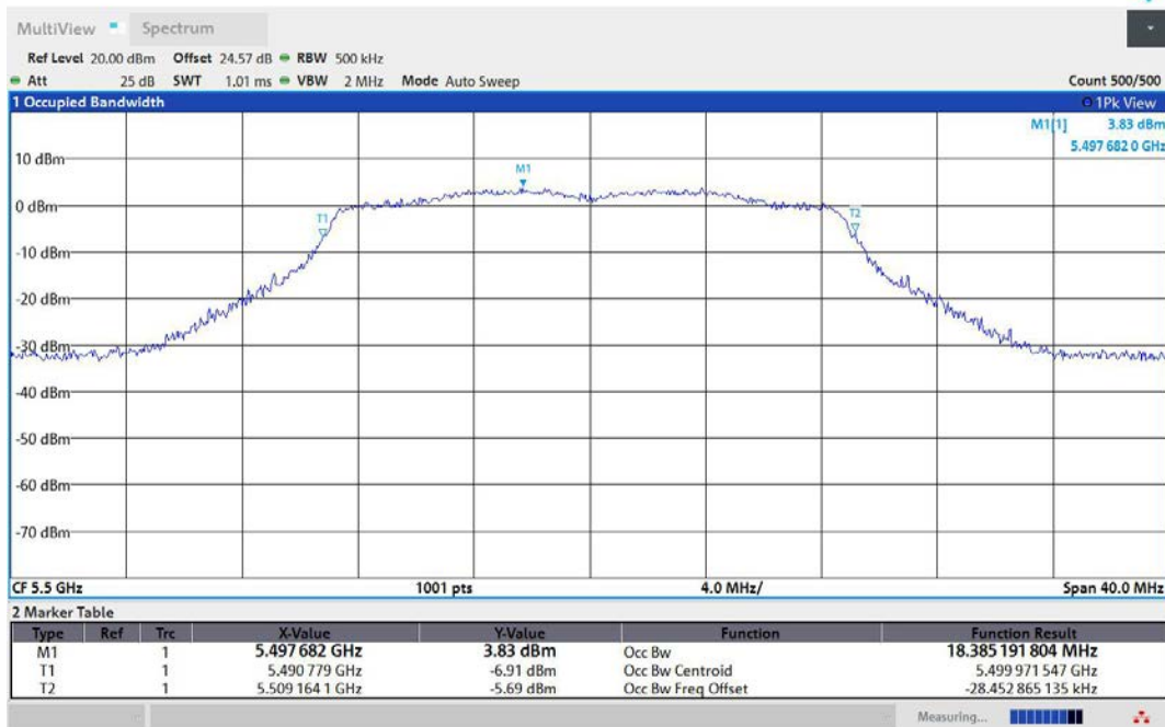
11N20MIMO-Ant1-5500
