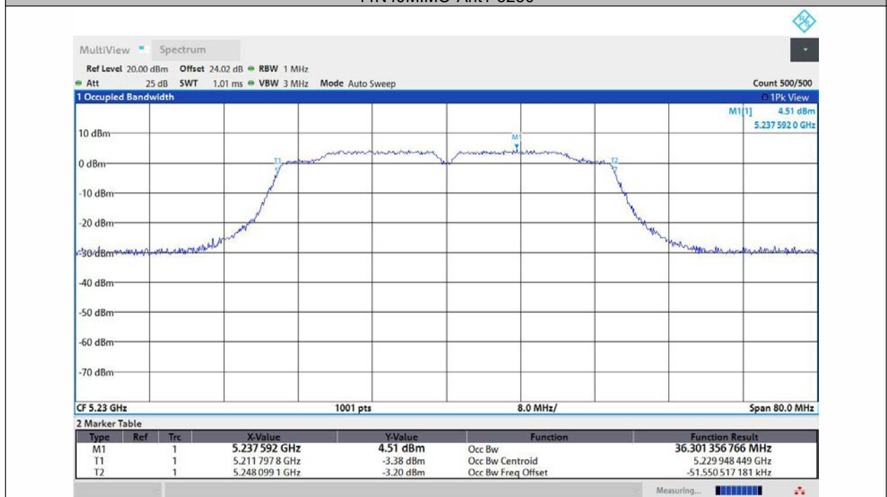
11N40MIMO-Ant2-5230
