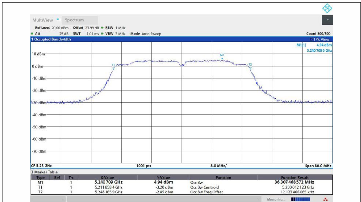
11N40MIMO-Ant1-5230
