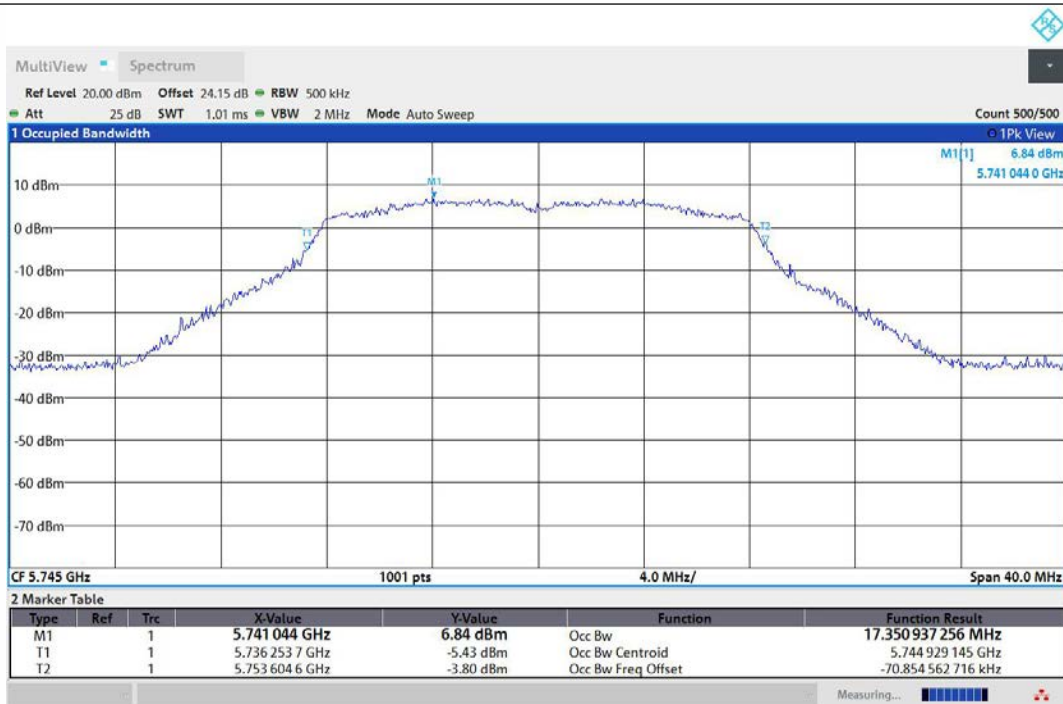
11A-Ant1-5745
