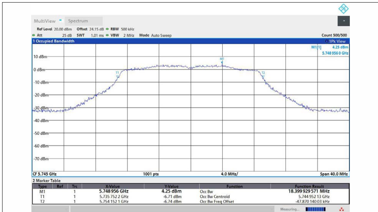
11N20MIMO-Ant1-5745
