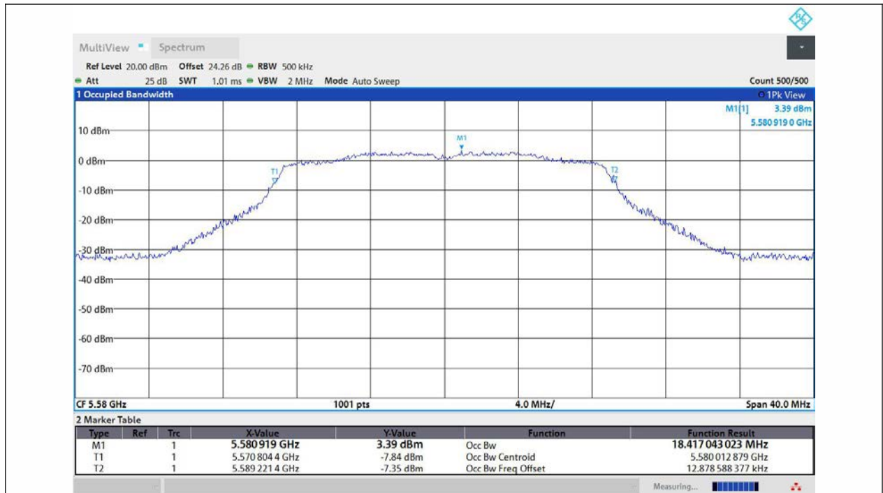
11N20MIMO-Ant1-5580
