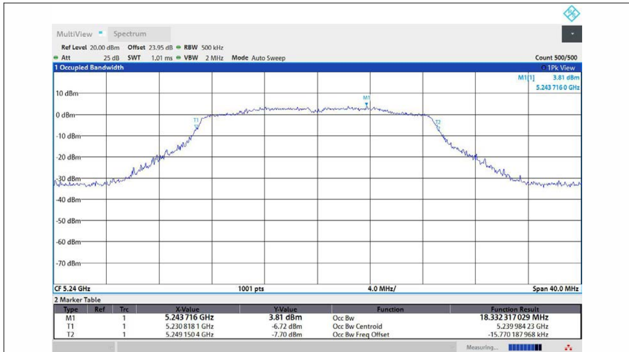
11N20MIMO-Ant1-5240
