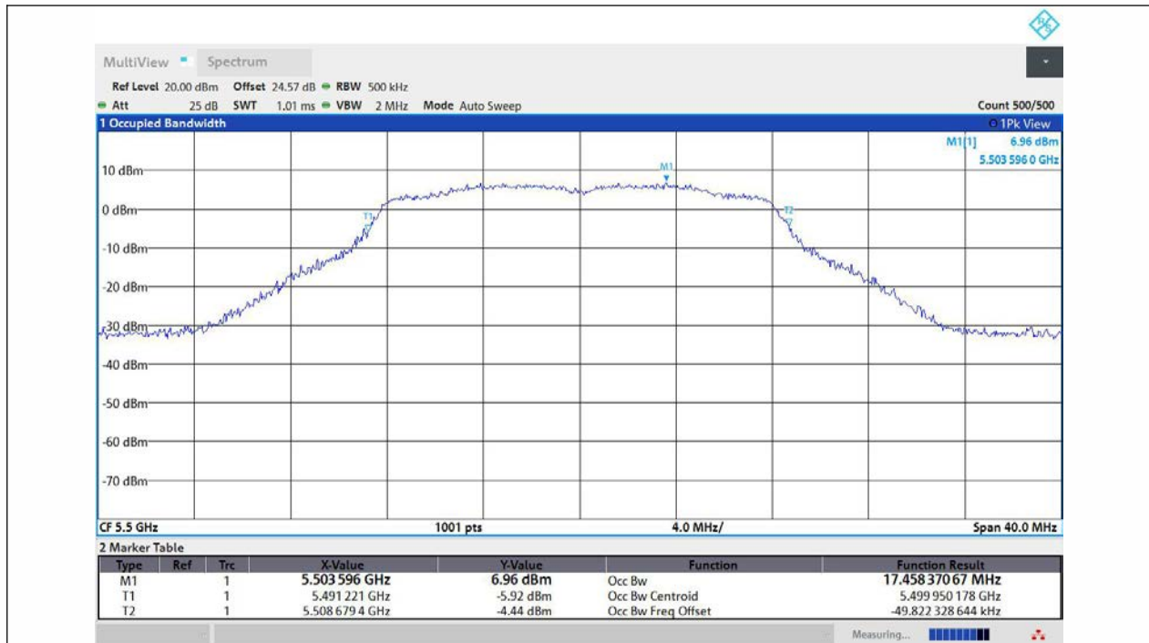
11A-Ant1-5500
