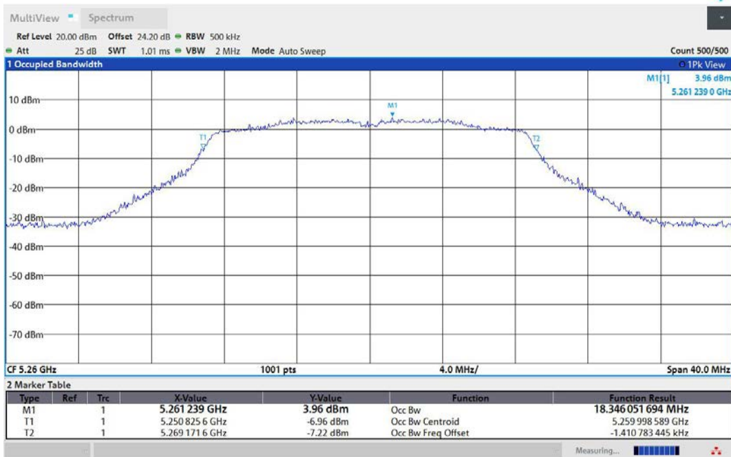
11AC20MIMO-Ant1-5260
