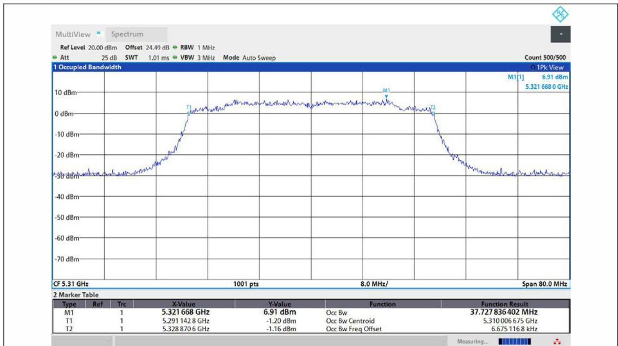
11AX40MIMO-Ant1-5310
