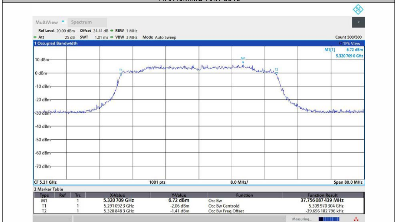
11AX40MIMO-Ant2-5310
