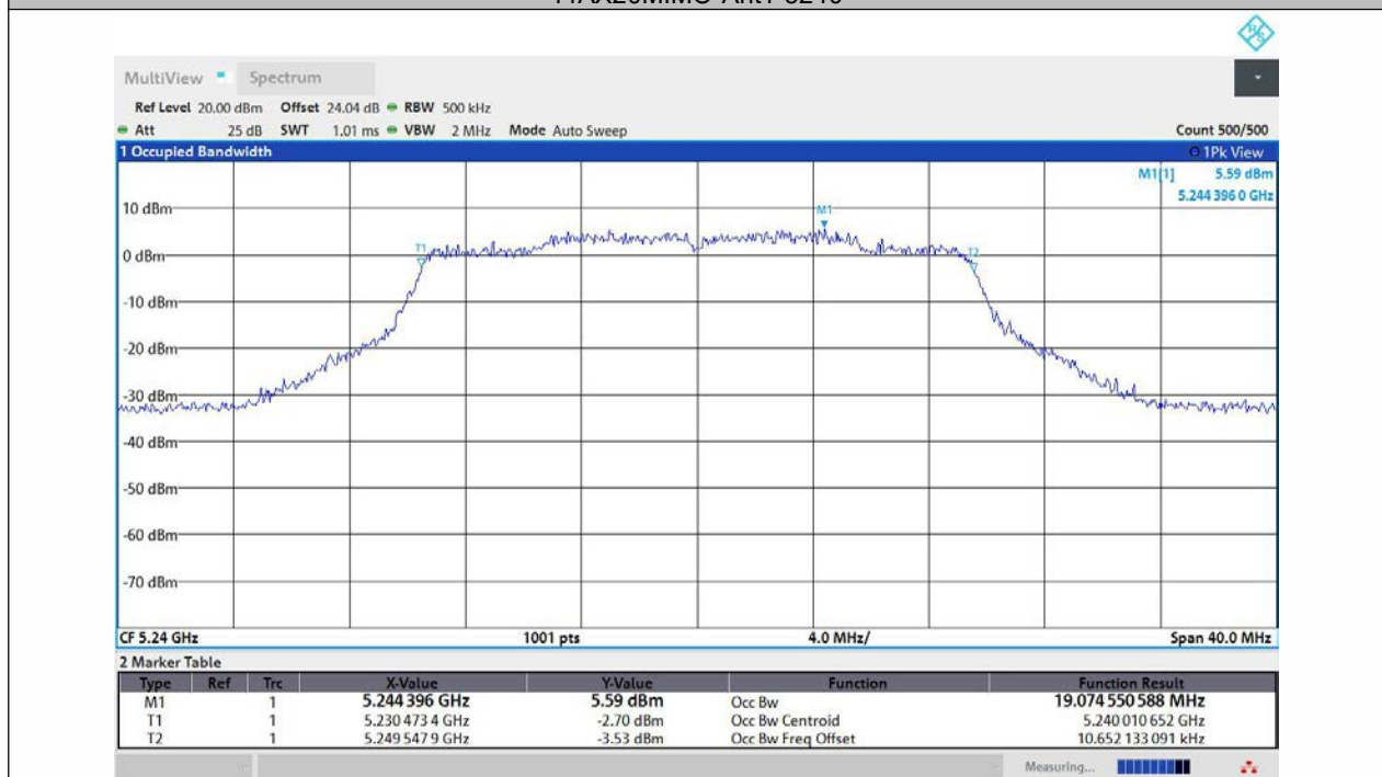
11AX20MIMO-Ant2-5240
