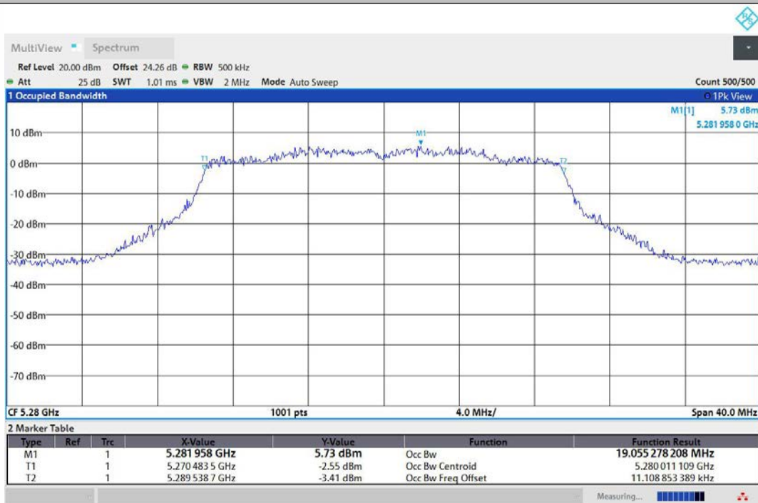
11AX20MIMO-Ant2-5280
