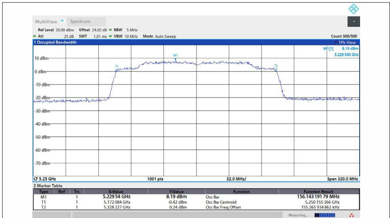
11AX160MIMO-Ant1-5250
