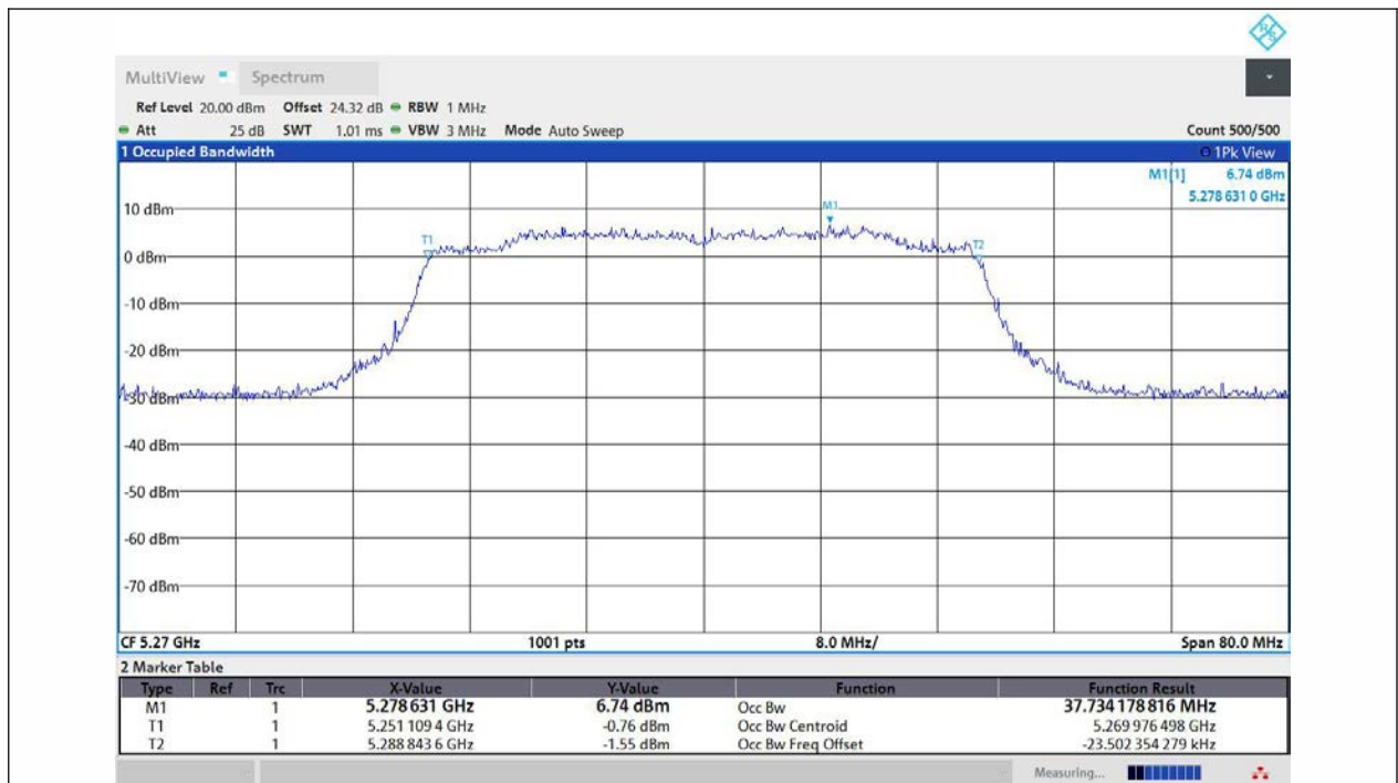
11AX40MIMO-Ant1-5270
