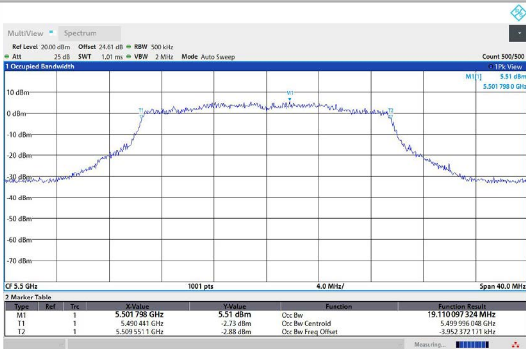
11AX20MIMO-Ant2-5500
