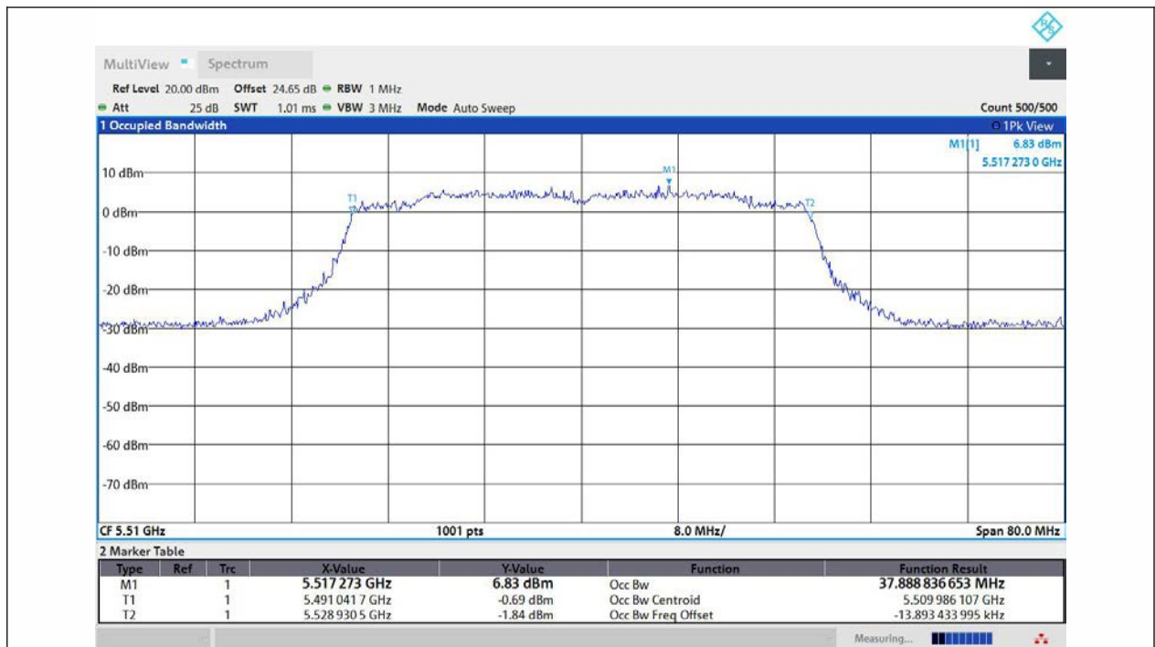
11AX40MIMO-Ant1-5510
