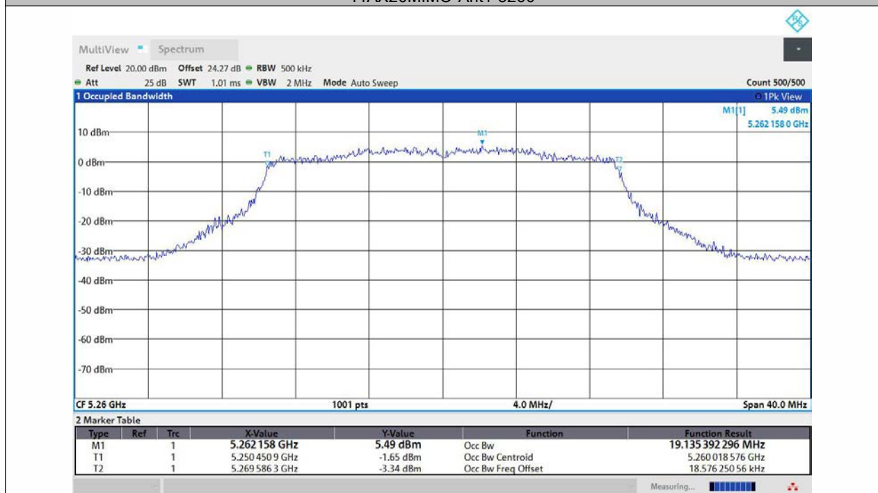
11AX20MIMO-Ant2-5260
