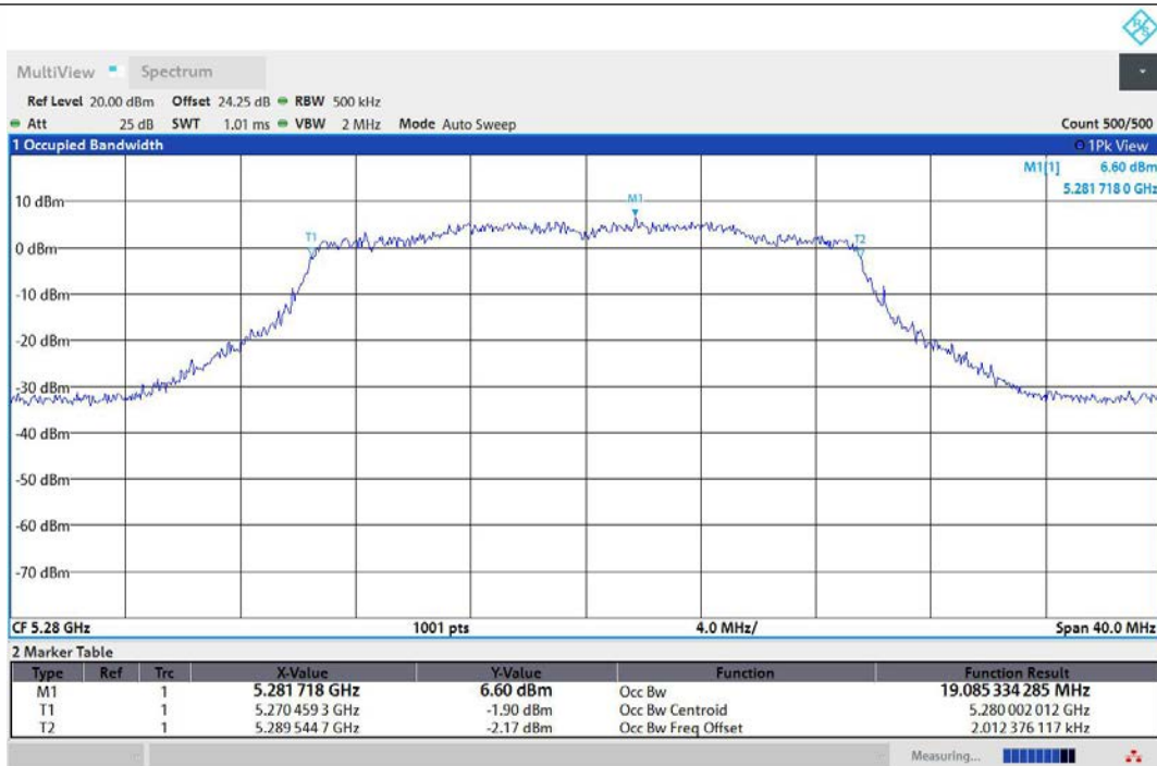
11AX20MIMO-Ant1-5280
