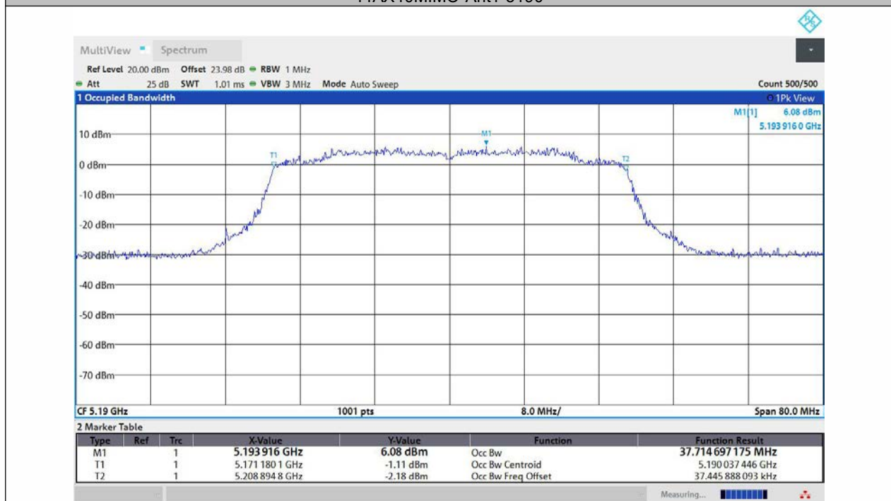
11AX40MIMO-Ant2-5190
