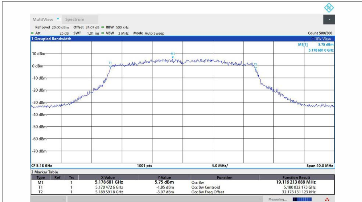
11AX20MIMO-Ant1-5180
