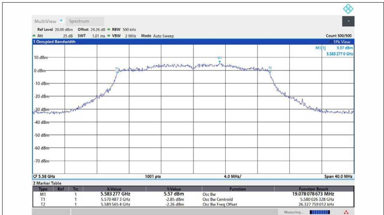
11AX20MIMO-Ant1-5580
