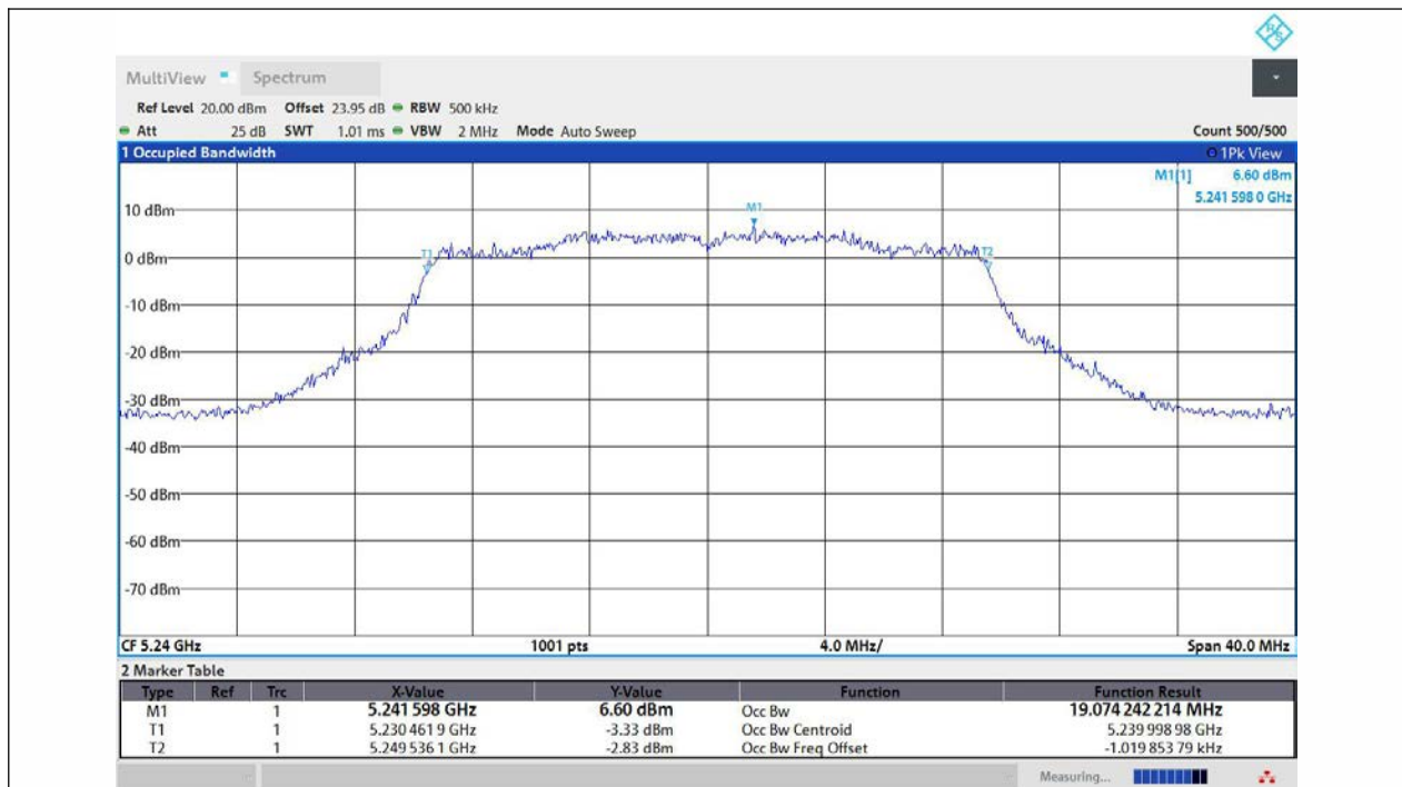
11AX20MIMO-Ant1-5240
