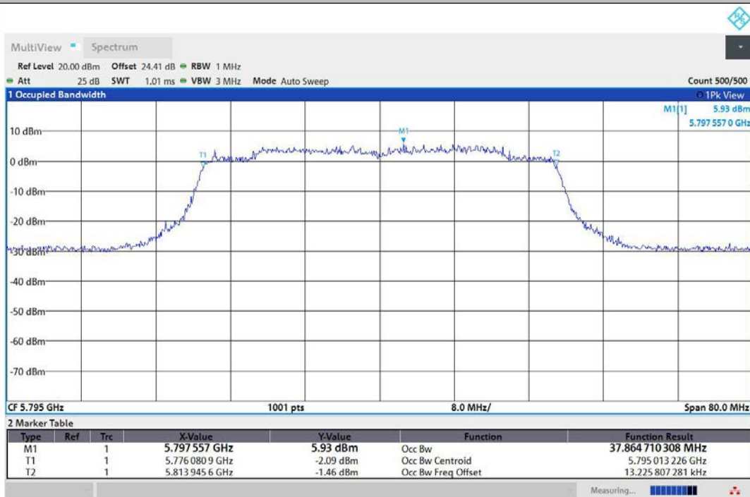
11AX40MIMO-Ant2-5795
