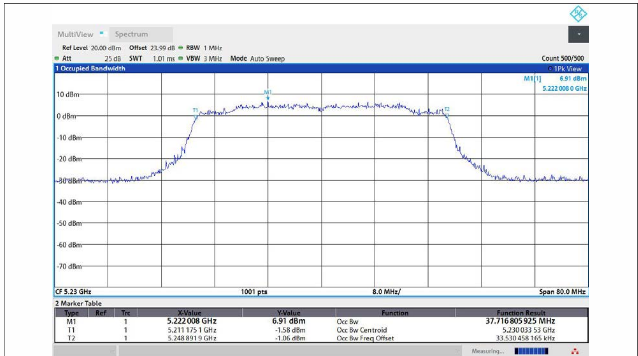
11AX40MIMO-Ant1-5230
