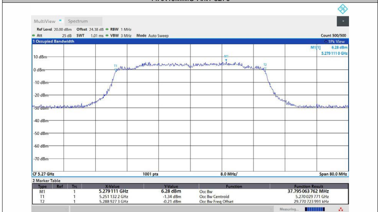
11AX40MIMO-Ant2-5270
