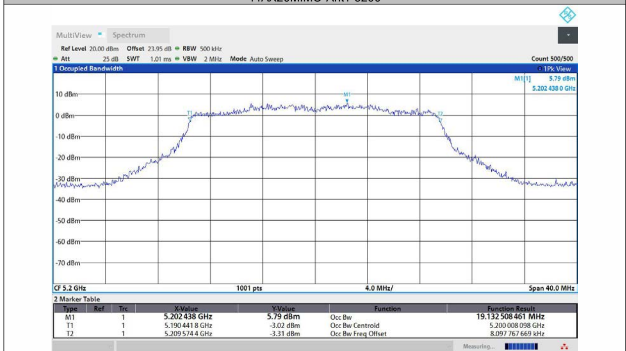
11AX20MIMO-Ant2-5200
