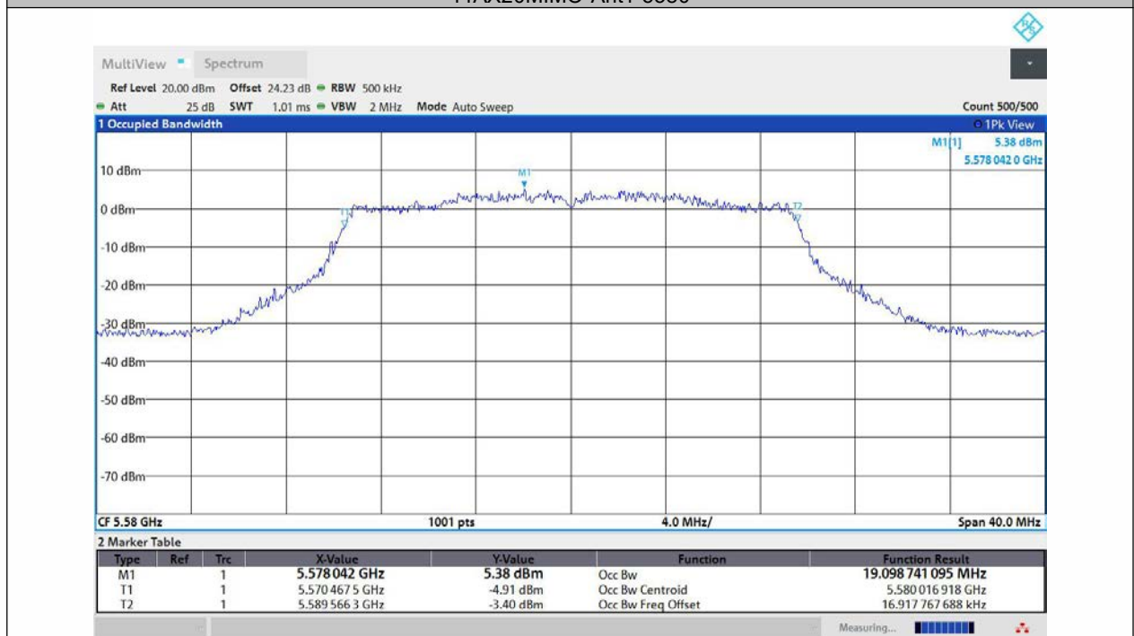
11AX20MIMO-Ant2-5580
