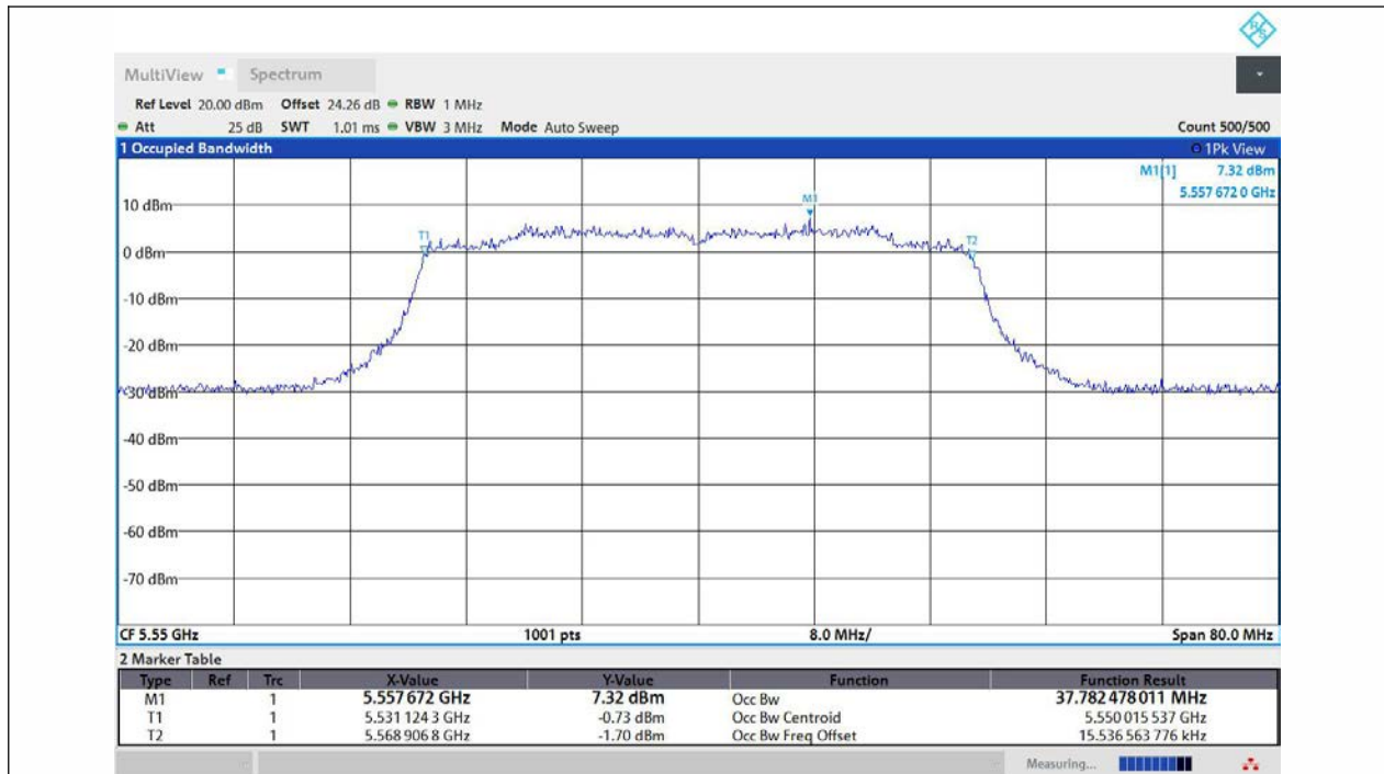
11AX40MIMO-Ant1-5550
