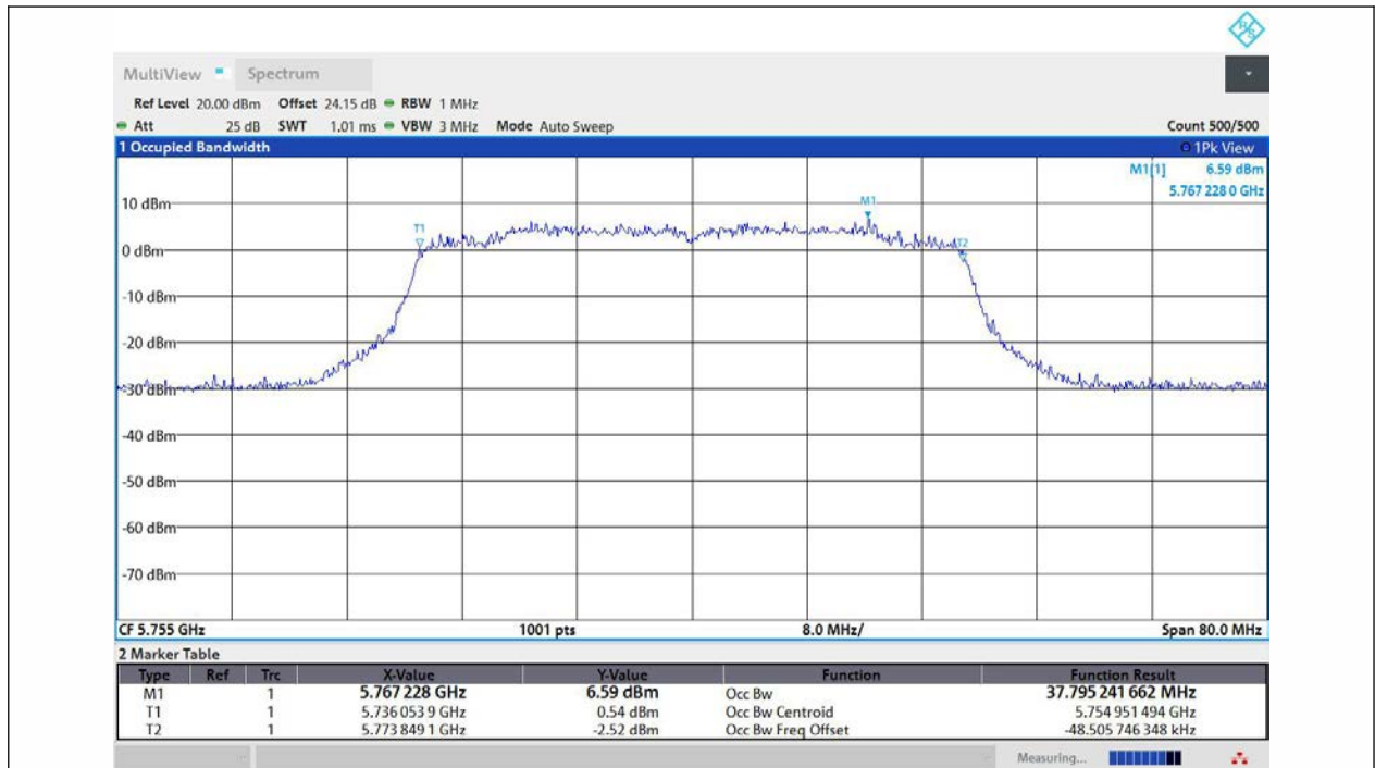
11AX40MIMO-Ant1-5755
