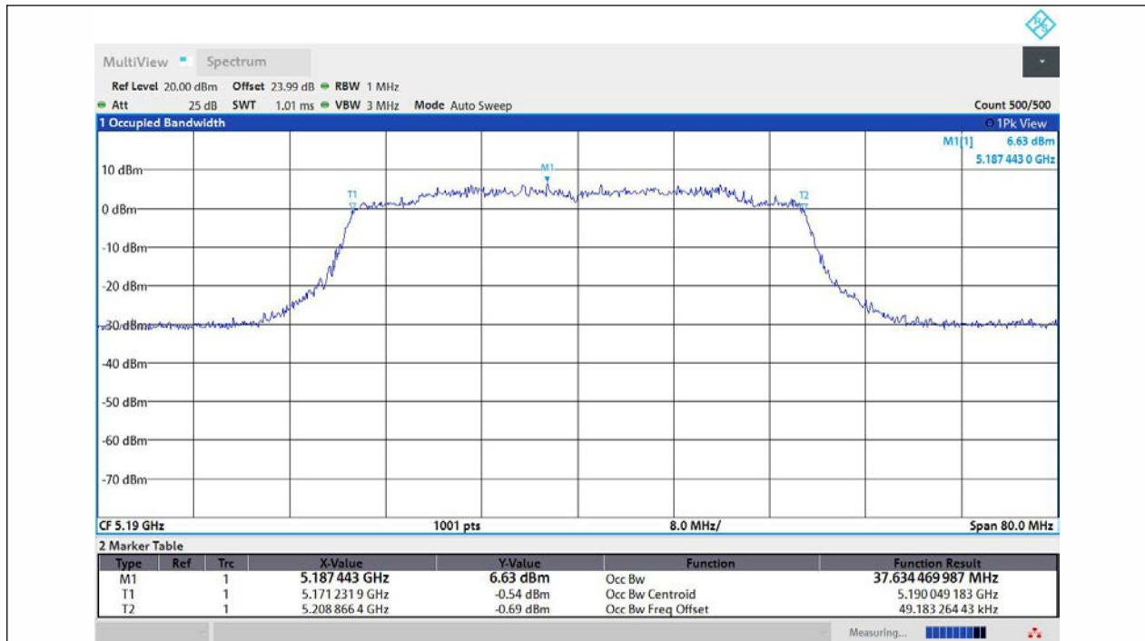
11AX40MIMO-Ant1-5190
