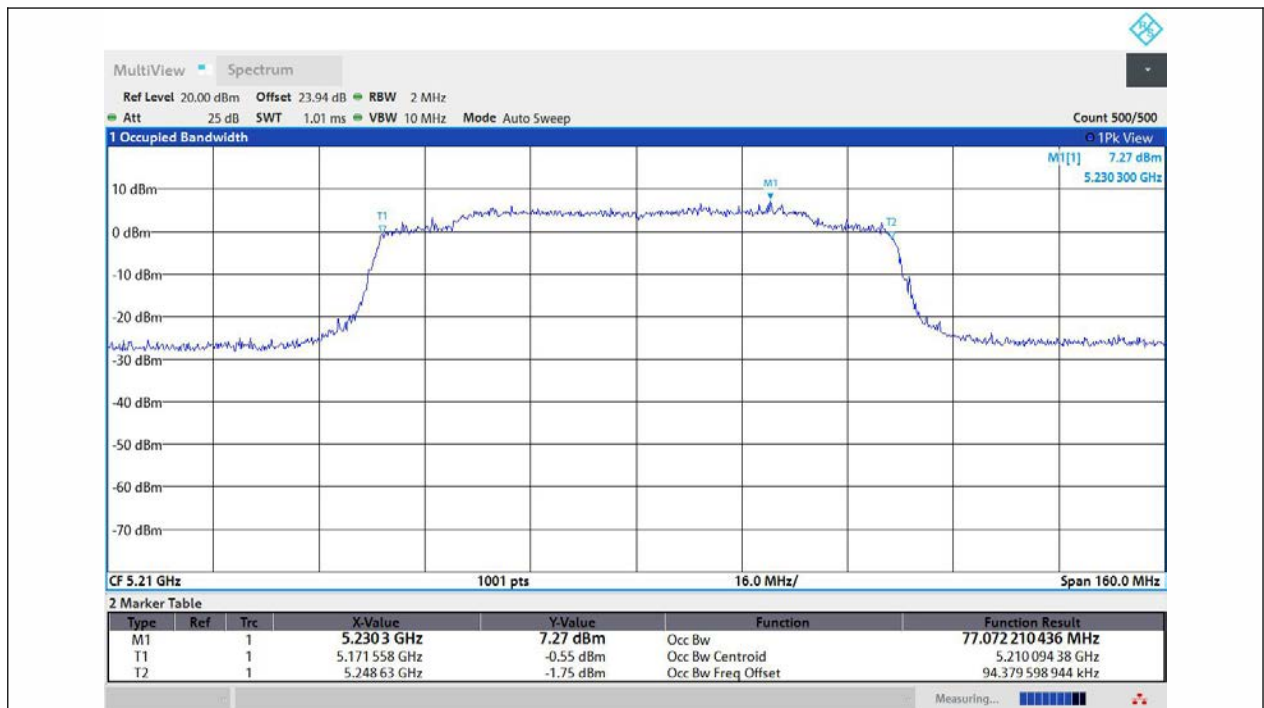
11AX80MIMO-Ant1-5210
