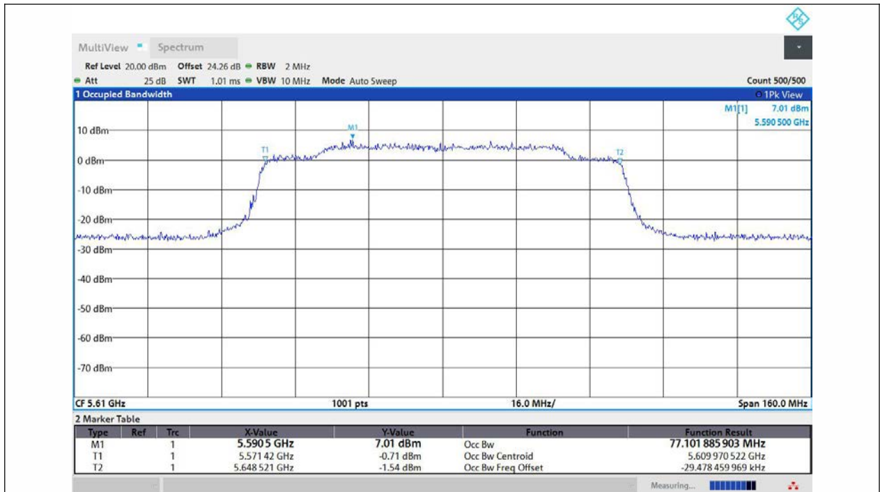
11AX80MIMO-Ant1-5610
