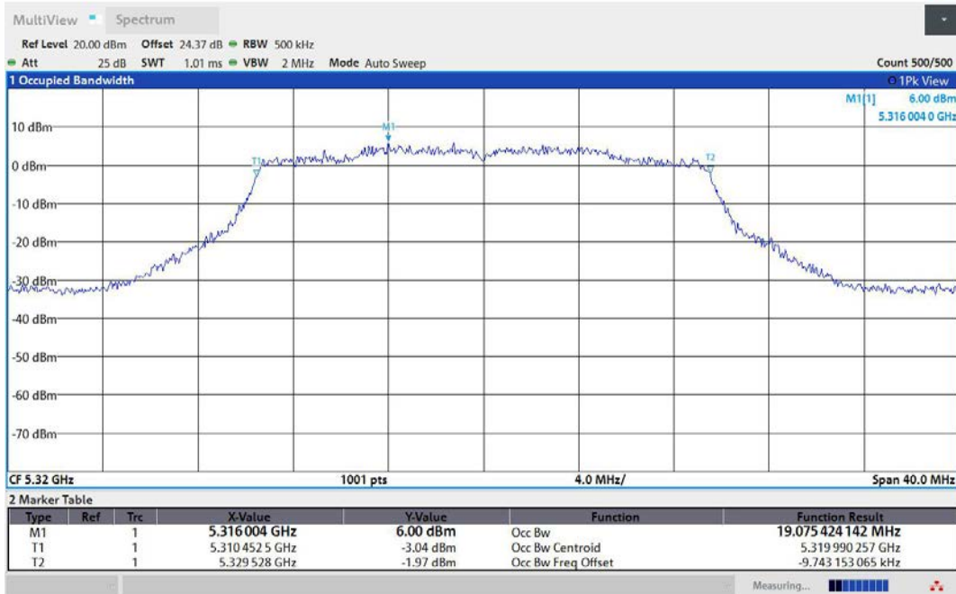
11AX20MIMO-Ant2-5320
