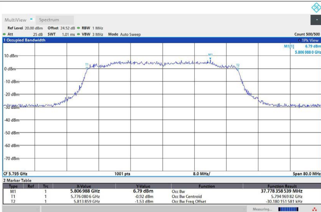
11AX40MIMO-Ant1-5795
