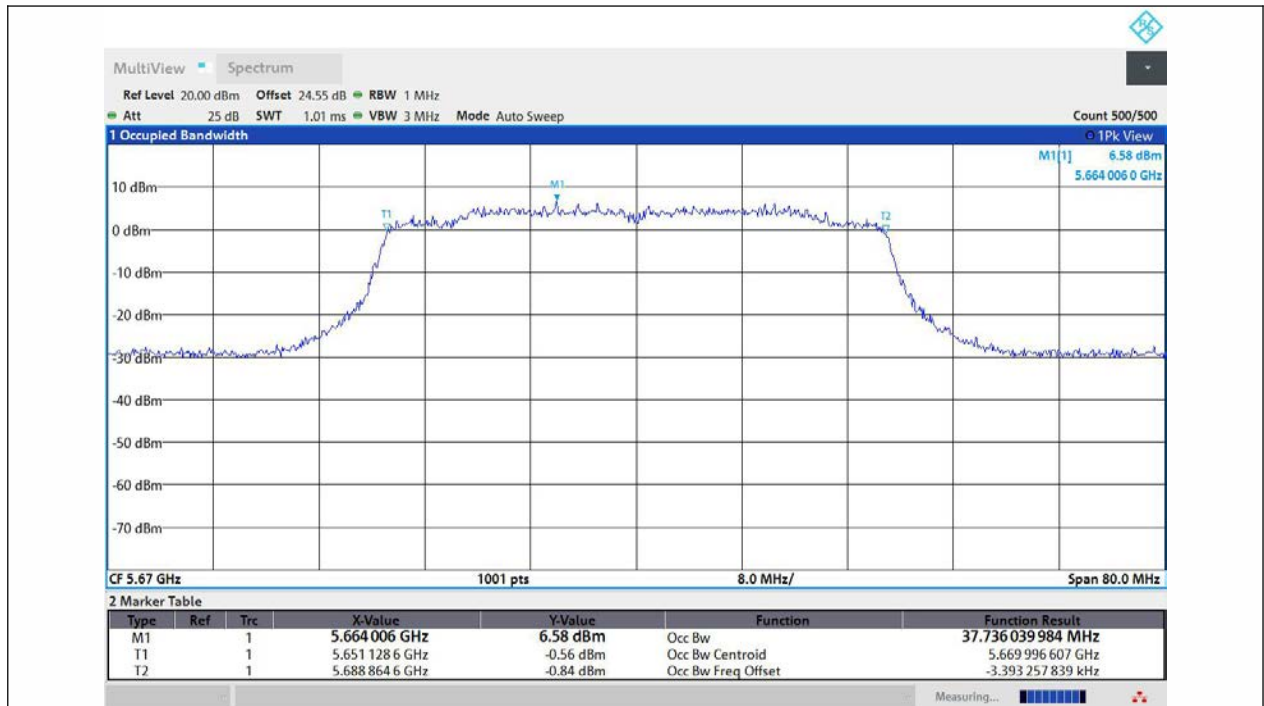
11AX40MIMO-Ant1-5670
