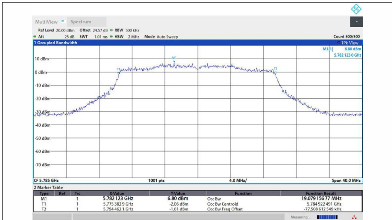
11AX20MIMO-Ant1-5785
