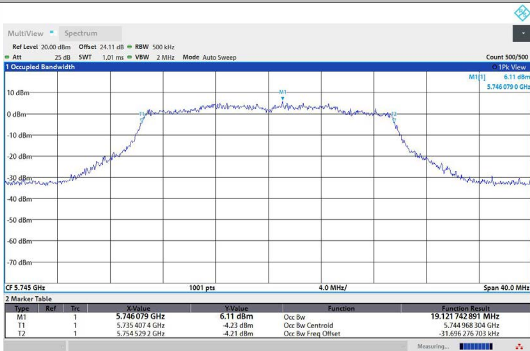
11AX20MIMO-Ant2-5745
