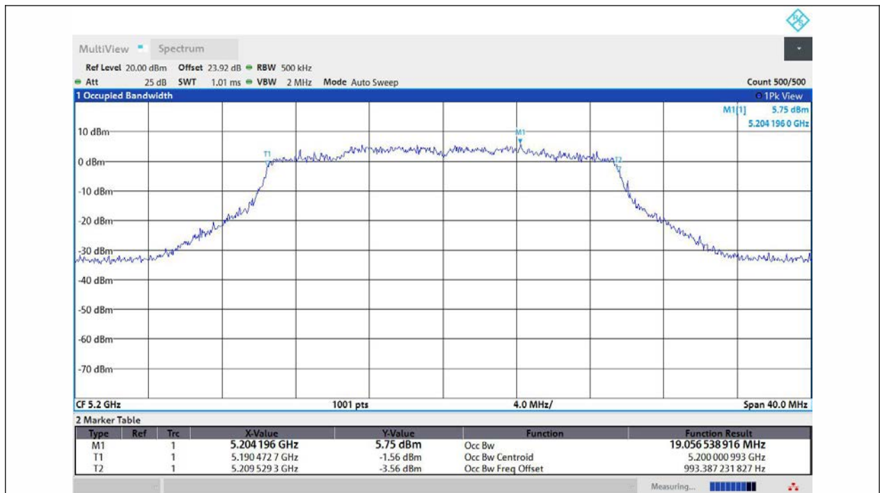
11AX20MIMO-Ant1-5200
