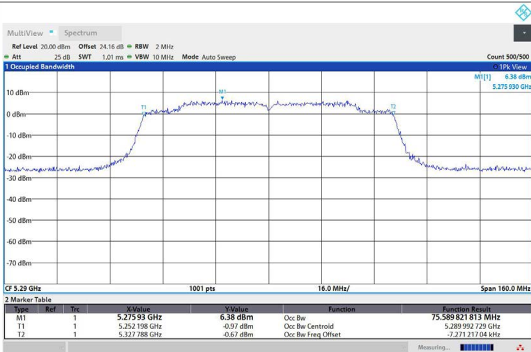
11AC80MIMO-Ant1-5290
