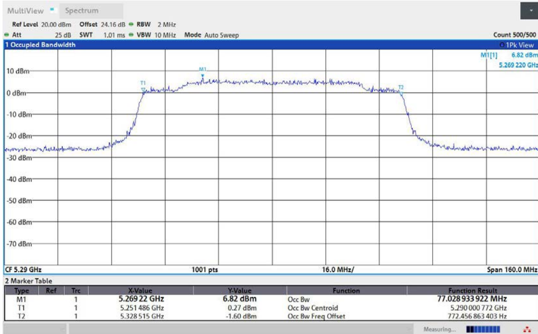
11AX80MIMO-Ant1-5290
