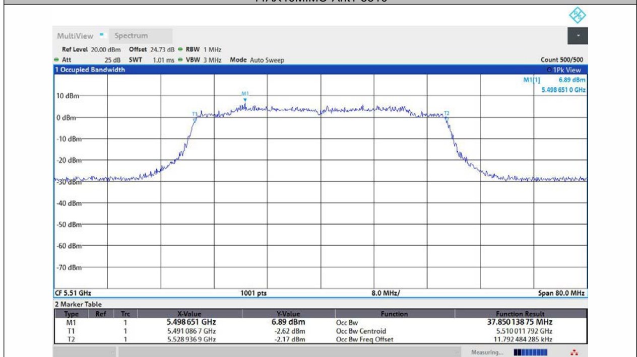
11AX40MIMO-Ant2-5510
