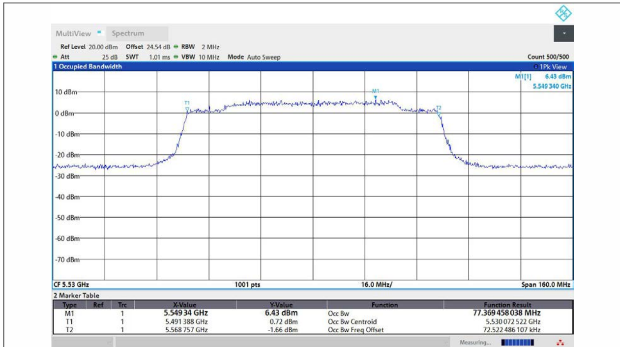
11AX80MIMO-Ant1-5530
