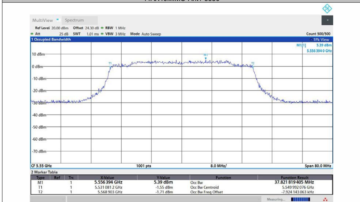
11AX40MIMO-Ant2-5550
