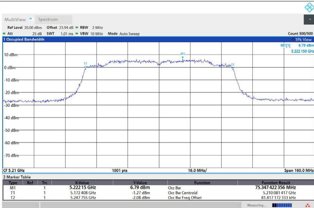
11AC80MIMO-Ant1-5210
