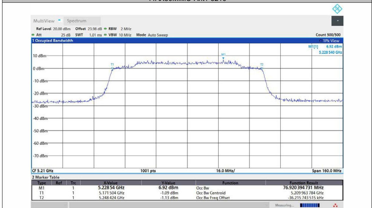
11AX80MIMO-Ant2-5210
