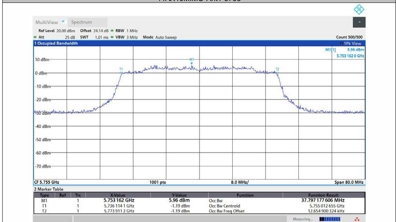
11AX40MIMO-Ant2-5755
