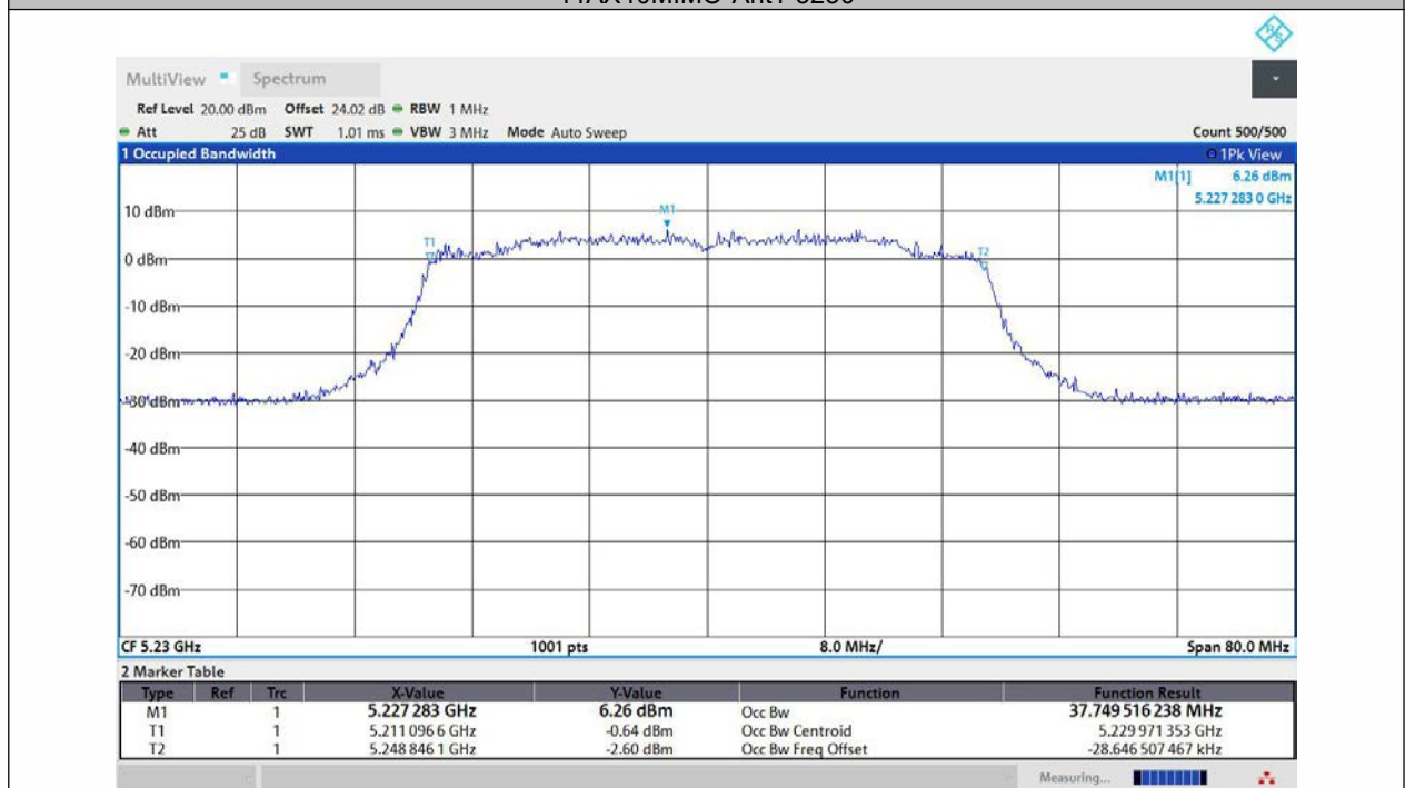
11AX40MIMO-Ant2-5230
