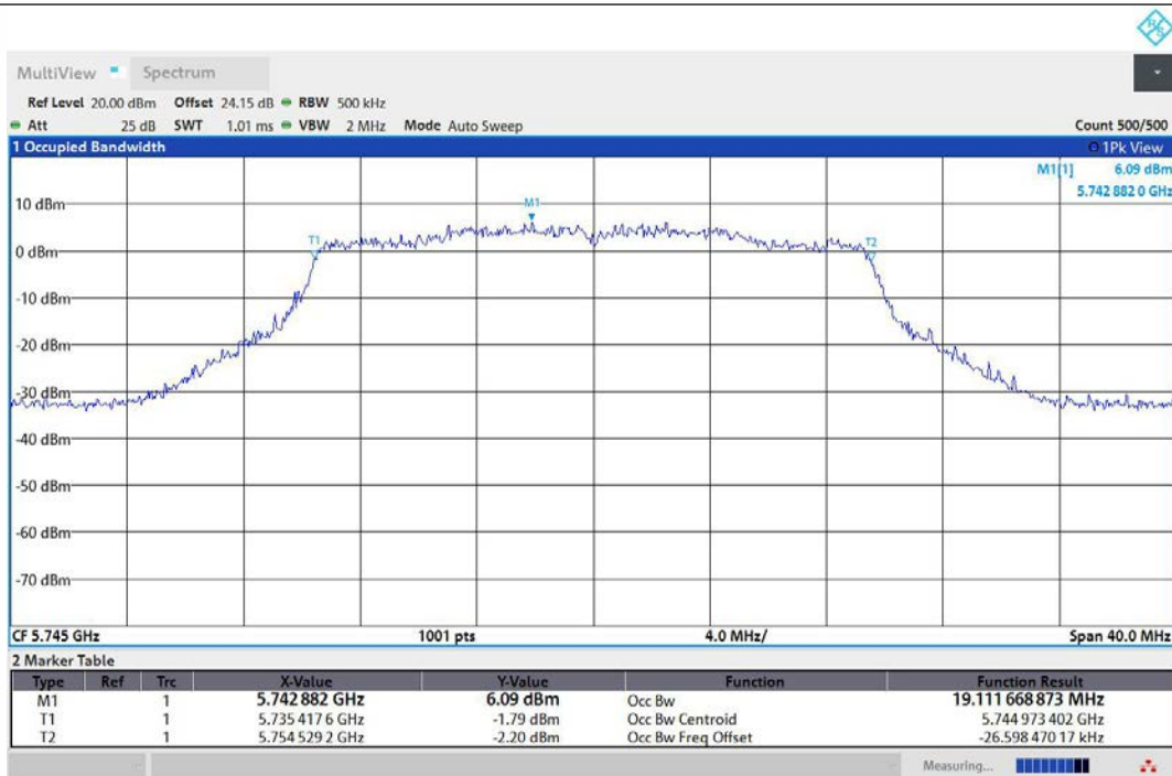
11AX20MIMO-Ant1-5745
