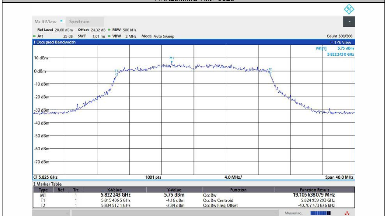
11AX20MIMO-Ant2-5825
