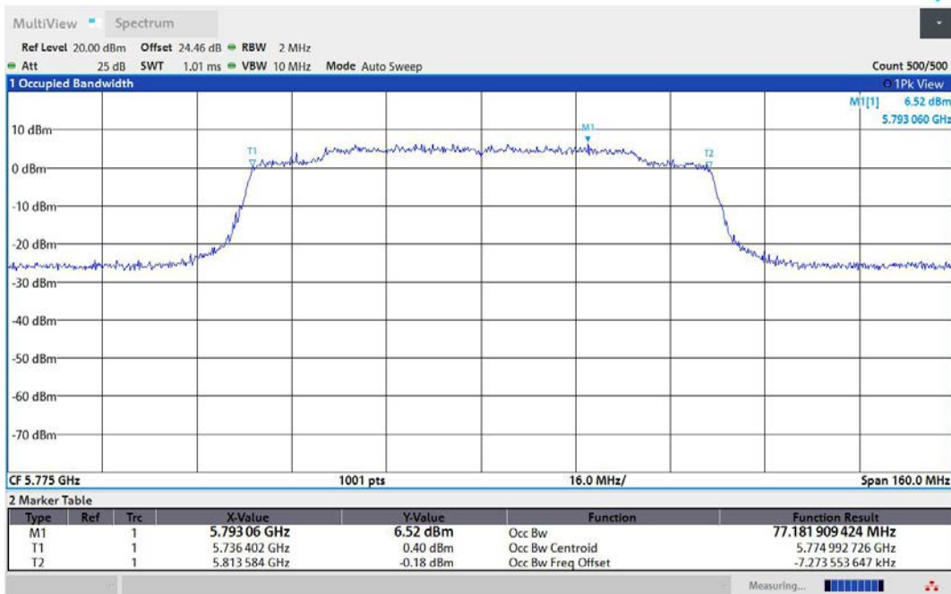
11AX80MIMO-Ant1-5775
