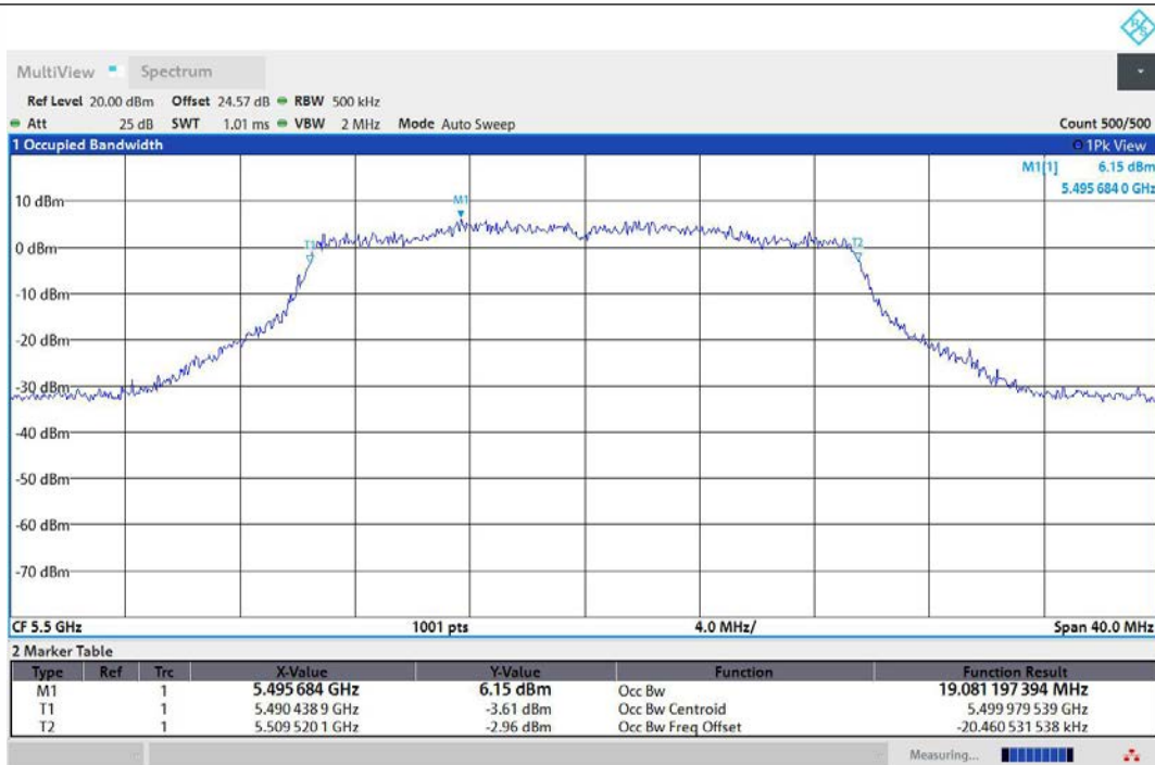
11AX20MIMO-Ant1-5500
