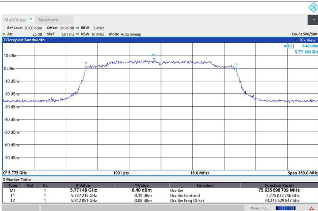
11AC80MIMO-Ant1-5775
