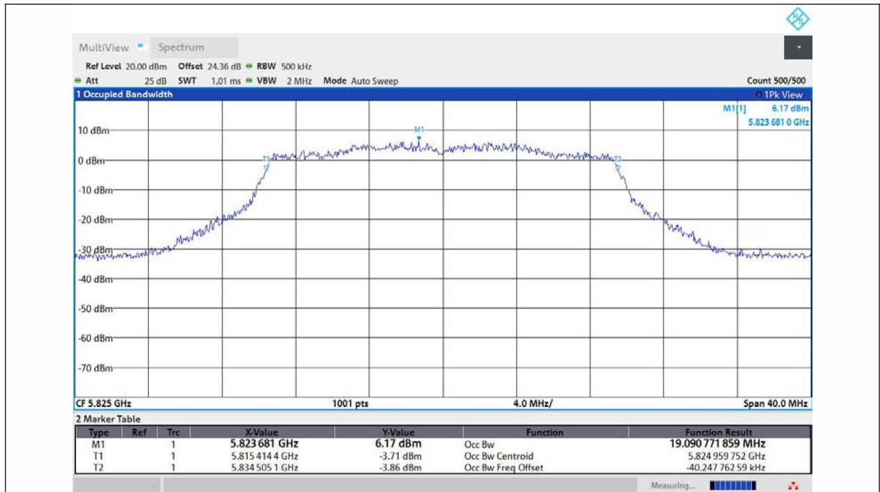
11AX20MIMO-Ant1-5825
