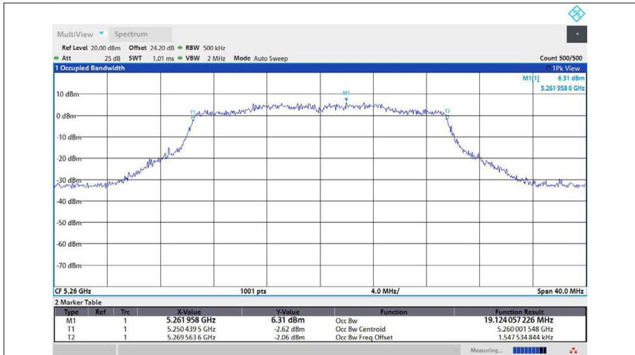
11AX20MIMO-Ant1-5260
