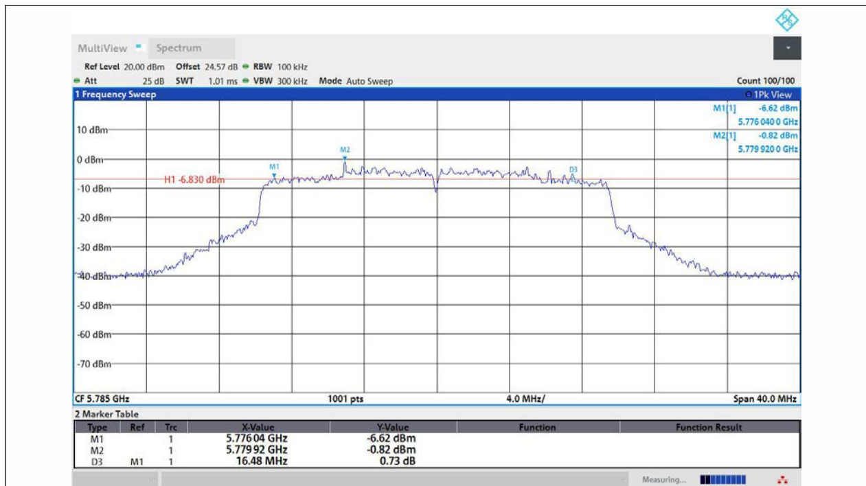
11AX20MIMO-Ant1-5785-PASS
