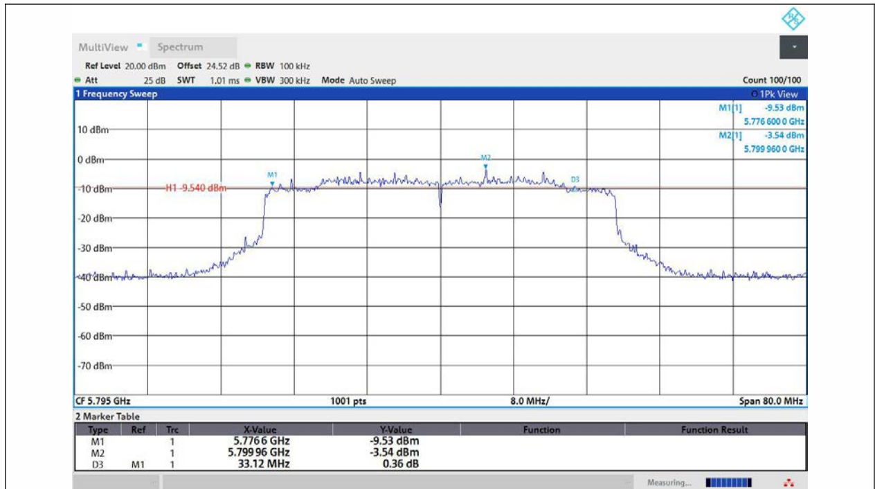
11AX40MIMO-Ant1-5795-PASS
