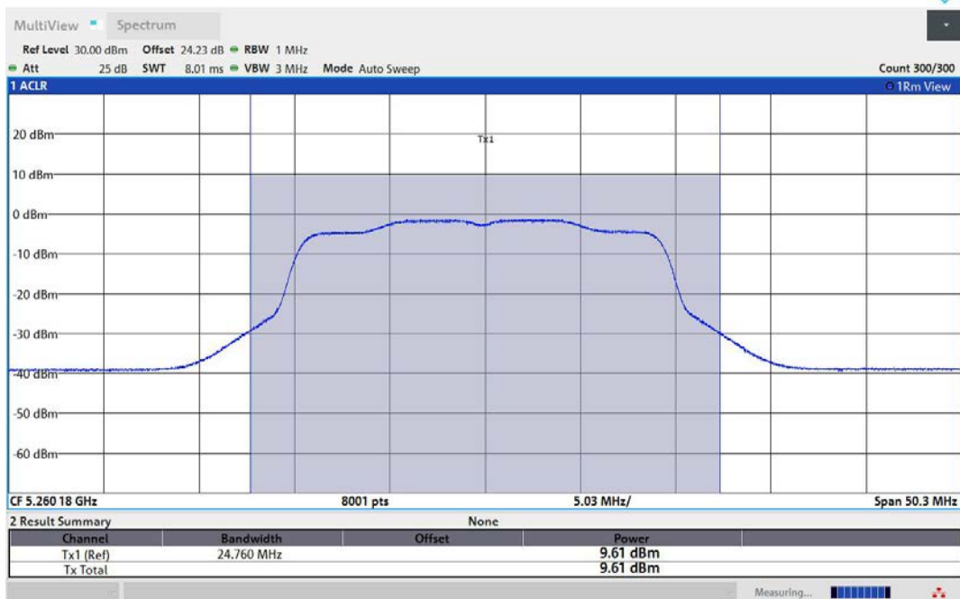
11AX20MIMO-Ant1-5260-PASS
