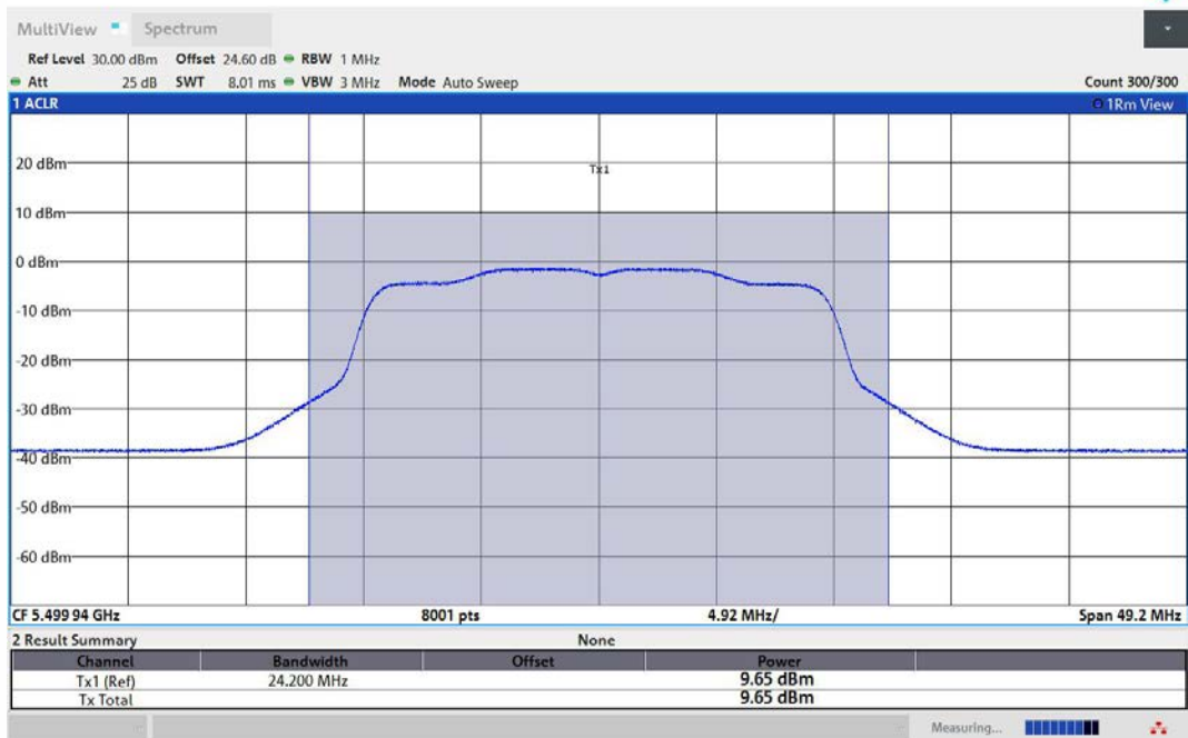
11AX20MIMO-Ant1-5500-PASS
