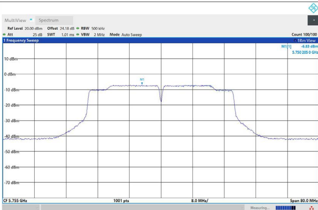
11N40MIMO-Ant1-5755-PASS
