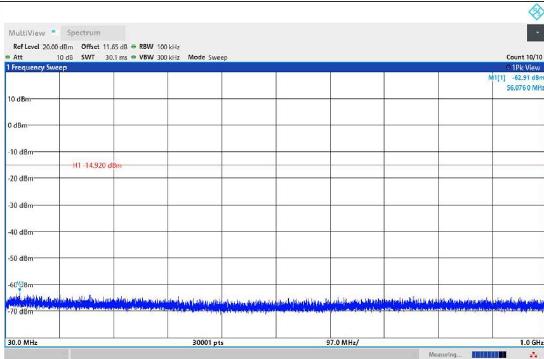
BLE_2M-Ant1-2480-30~1000-PASS
