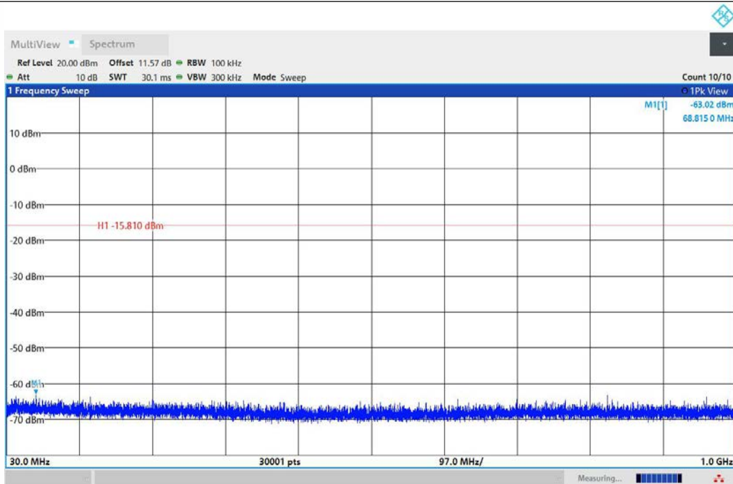
BLE_2M-Ant1-2440-30~1000-PASS
