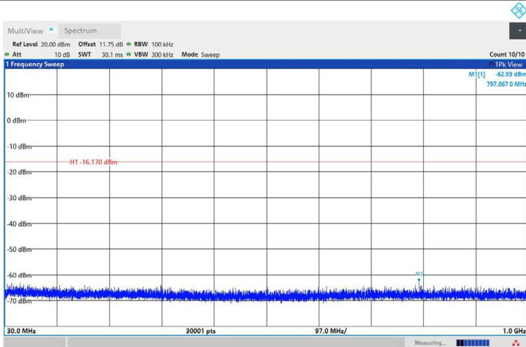
BLE_2M-Ant1-2402-30~1000-PASS
