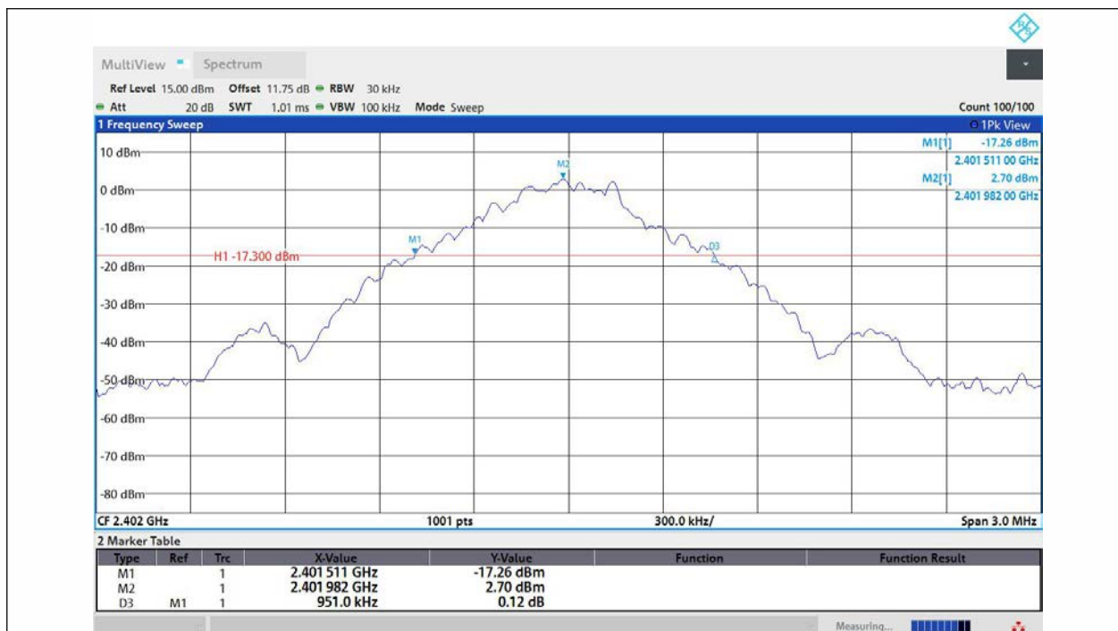
DH5-Ant1-2402
