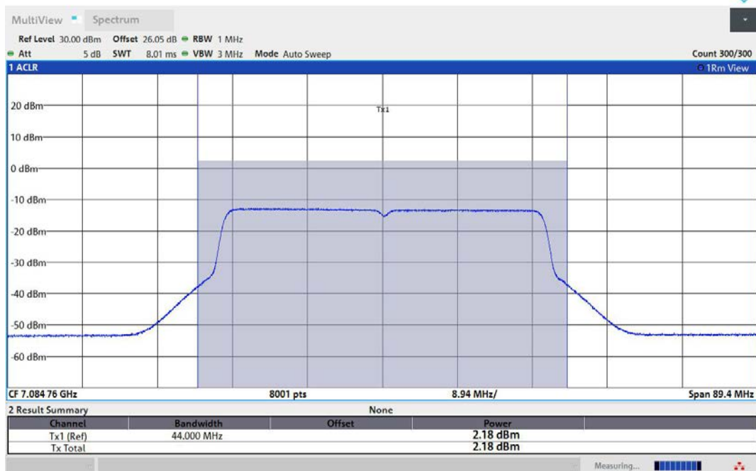
11AX40MIMO-Ant1-7085-PASS
