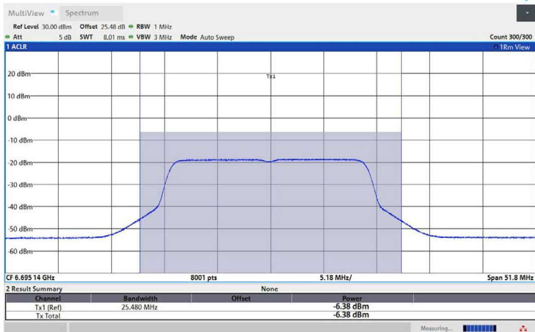
11AX20MIMO-Ant1-6695-PASS
