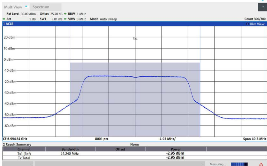
11AX20MIMO-Ant1-6995-PASS
