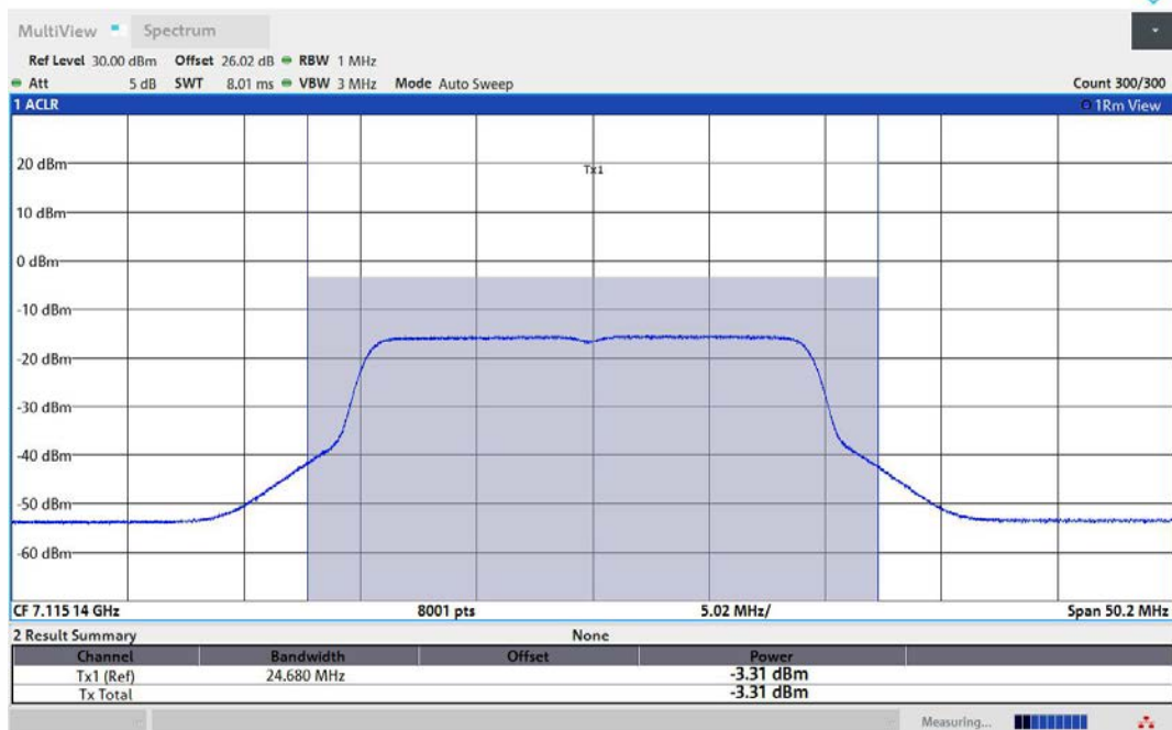
11AX20MIMO-Ant1-7115-PASS
