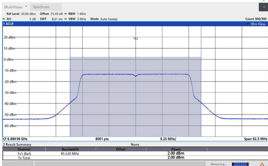
11AX40MIMO-Ant1-6685-PASS
