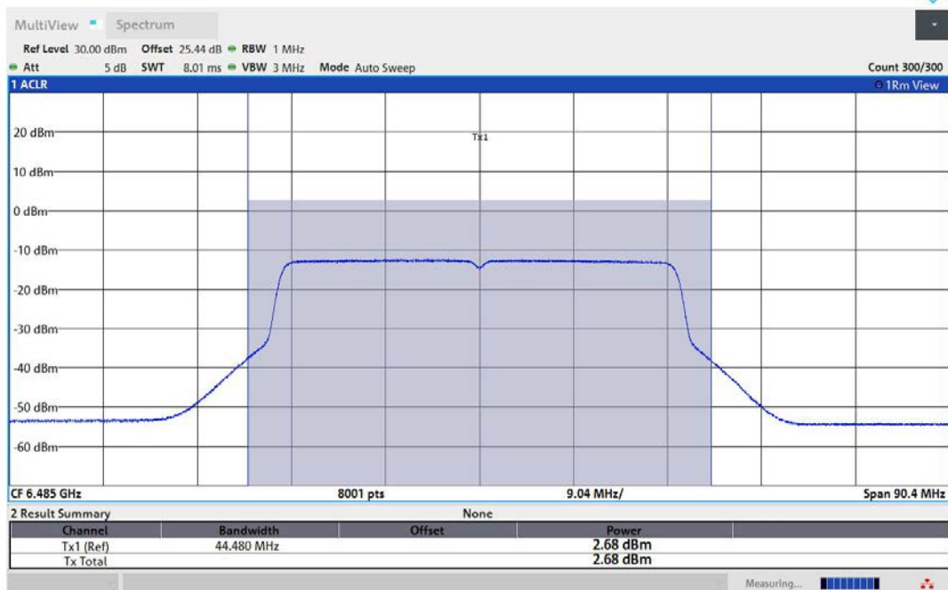
11AX40MIMO-Ant1-6485-PASS
