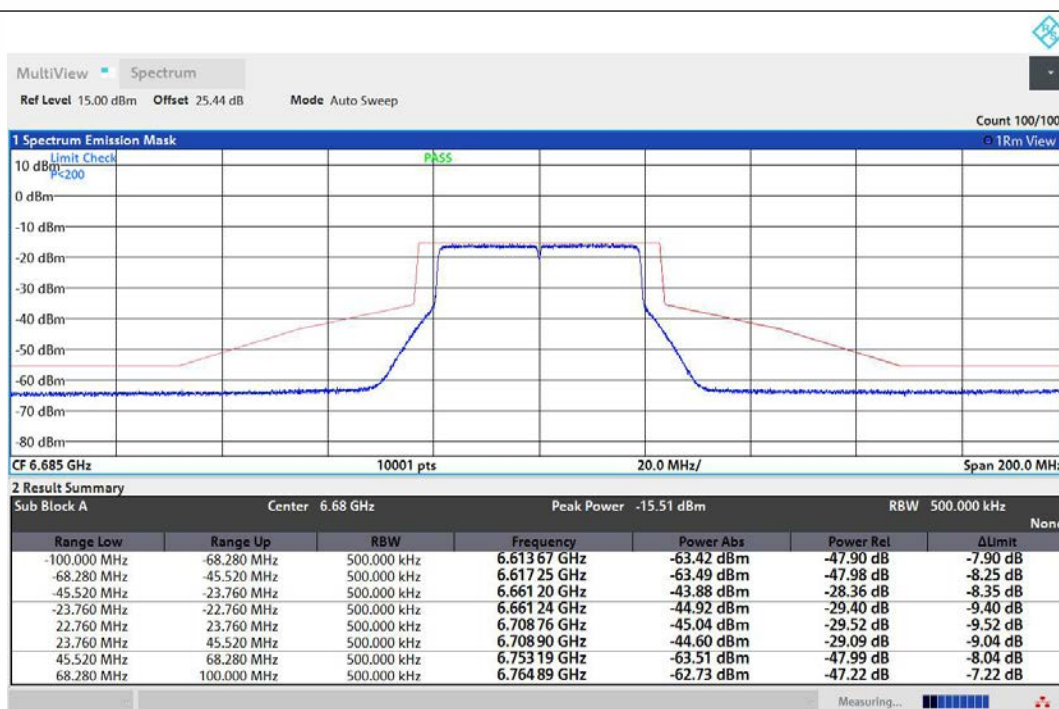
NTNV-11AX40MIMO-Ant1-6685-PASS
