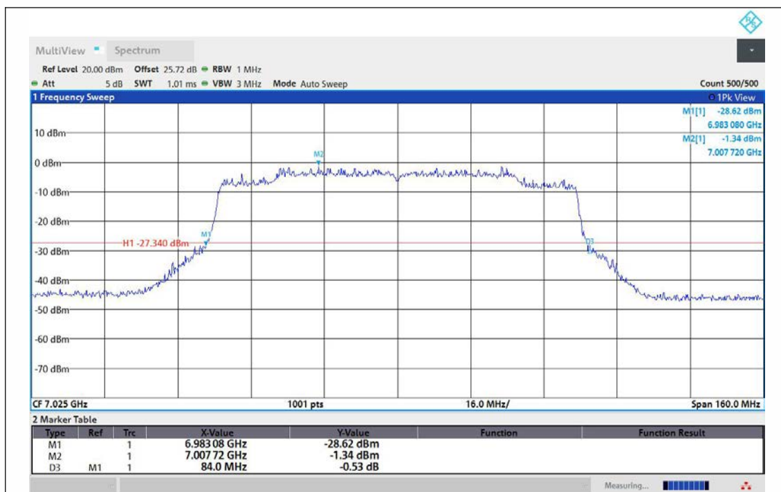
11AX80MIMO-Ant1-7025
