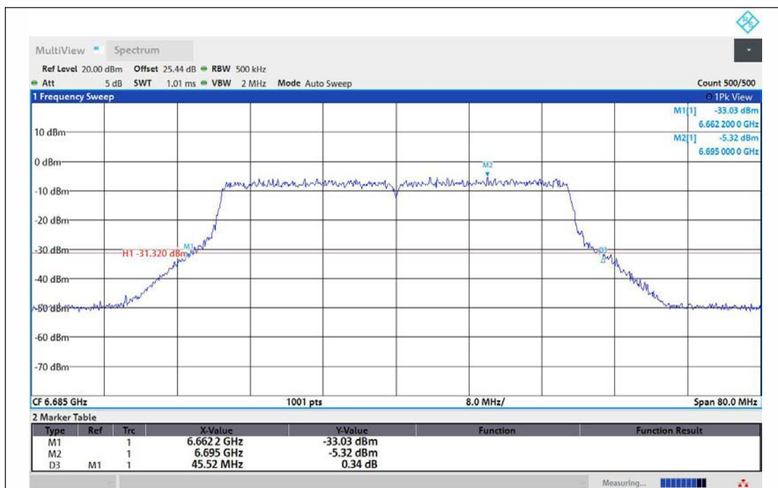
11AX40MIMO-Ant1-6685
