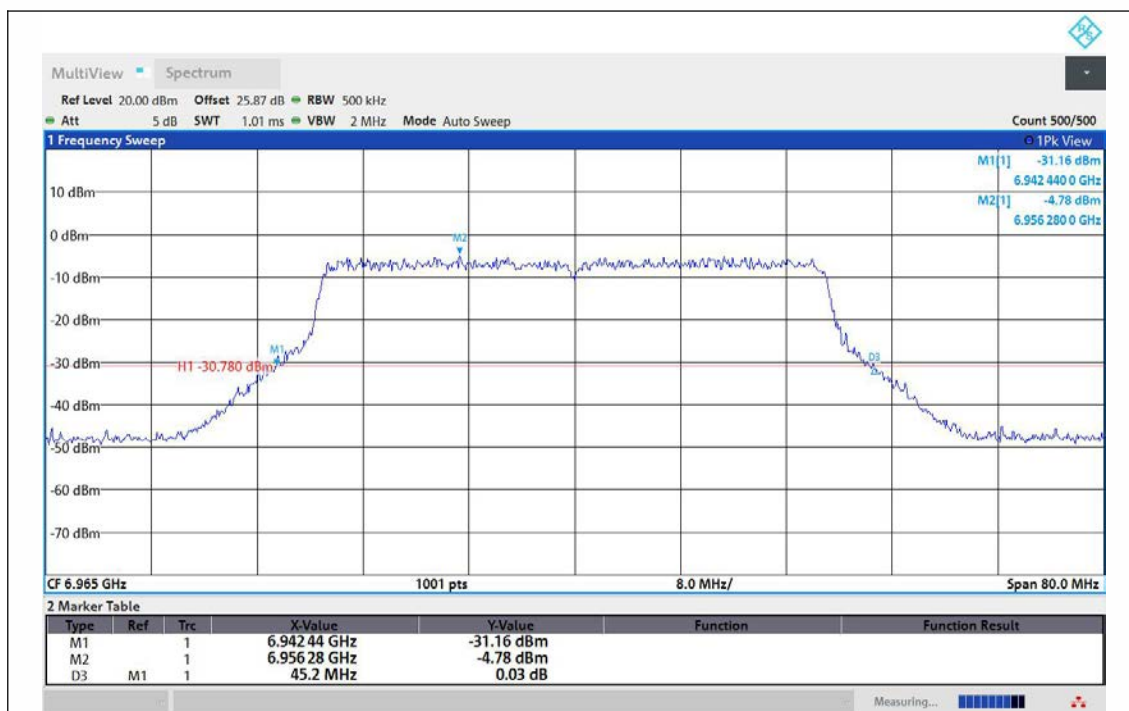
11AX40MIMO-Ant1-6965
