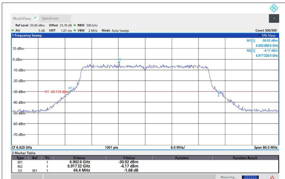
11AX40MIMO-Ant1-6925
