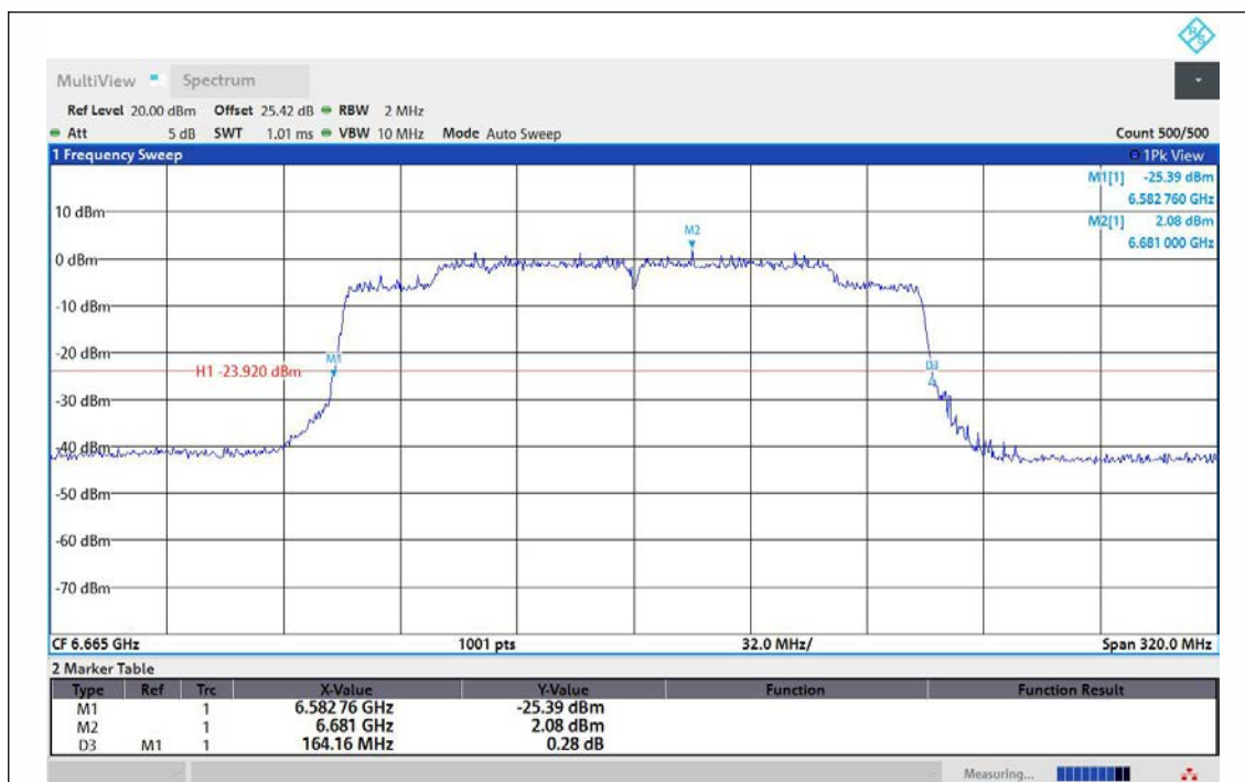
11AX160MIMO-Ant1-6665
