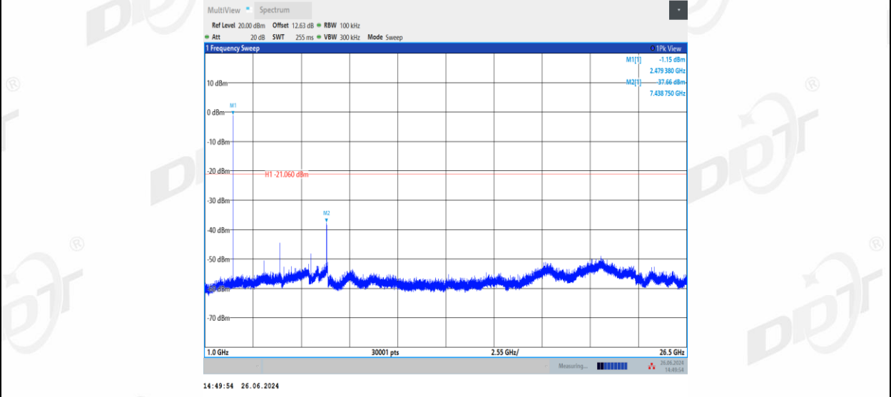
BLE_1M_Left side_2480_1000~26500
