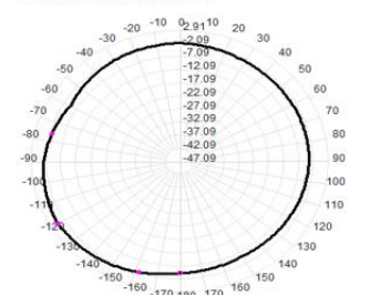
2470.0MHz Total(H), Max= 0.74dBi
