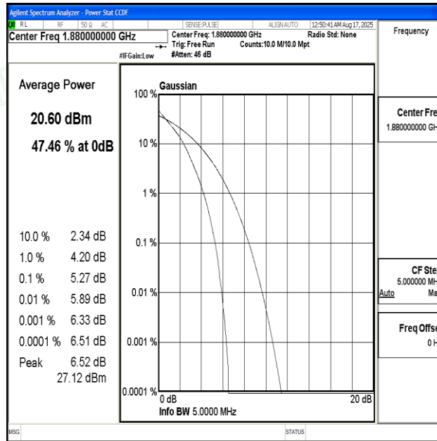
Band2-5MHz-QPSK-18900-25RB#0-PASS
