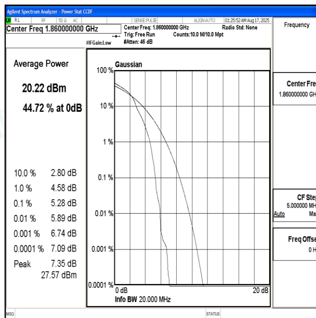
Band2-20MHz-16QAM-18700-1RB#0-PASS
