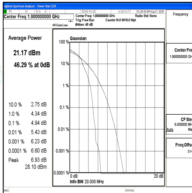
Band2-20MHz-16QAM-19100-1RB#0-PASS
