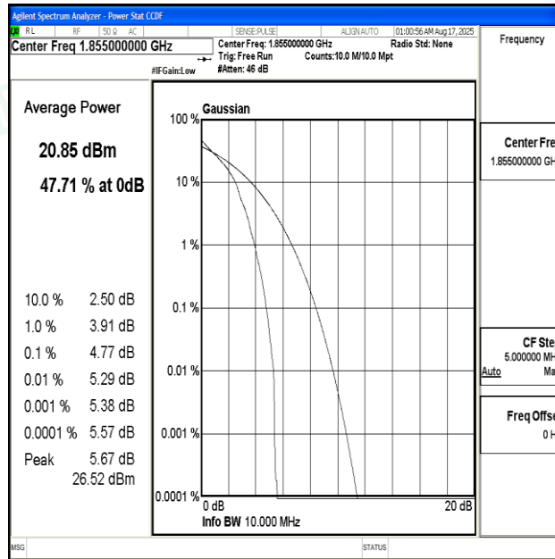
Band2-10MHz-QPSK-18650-1RB#0-PASS
