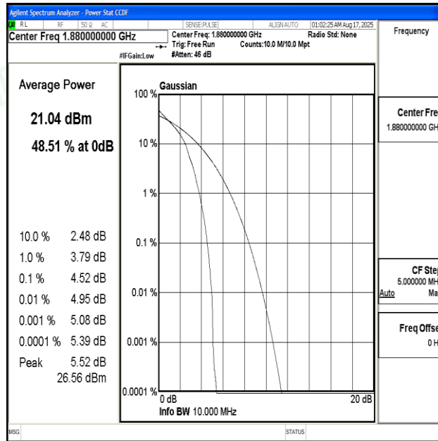
Band2-10MHz-QPSK-18900-1RB#0-PASS
