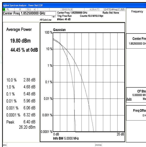
Band2-5MHz-16QAM-18625-1RB#0-PASS
