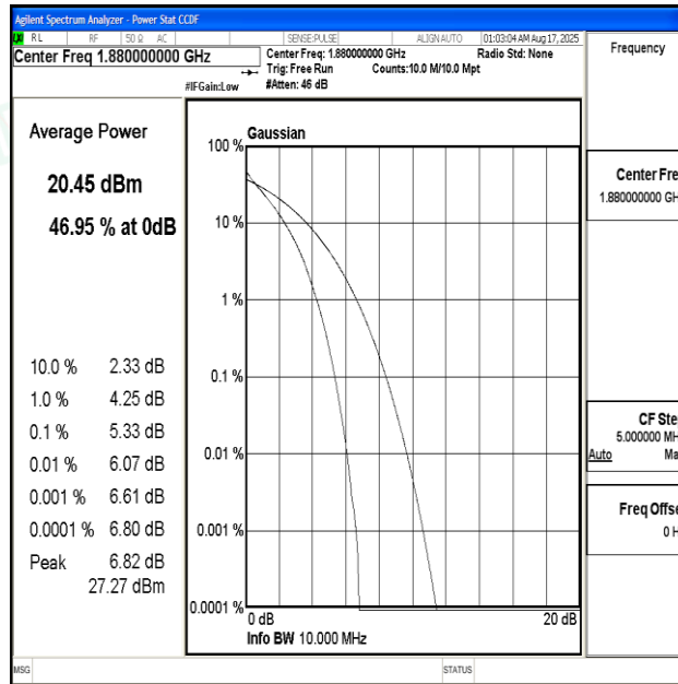
Band2-10MHz-QPSK-18900-50RB#0-PASS
