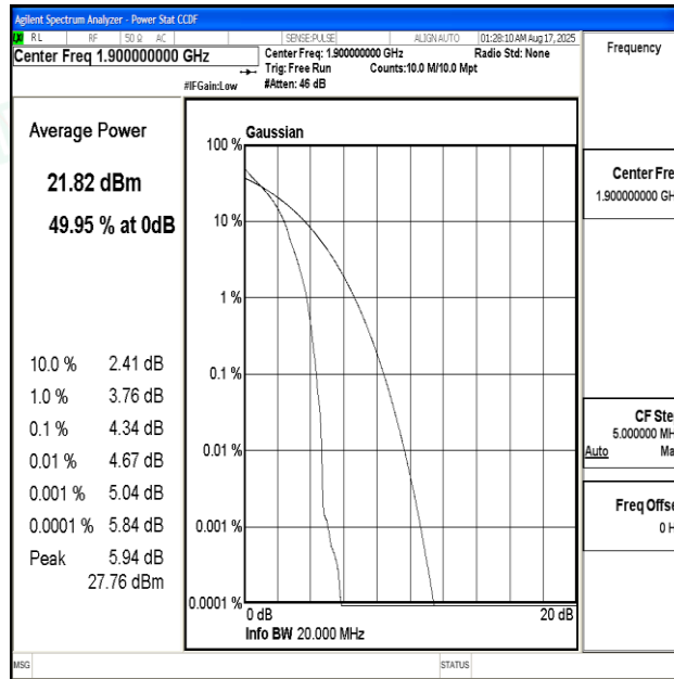
Band2-20MHz-QPSK-19100-1RB#0-PASS
