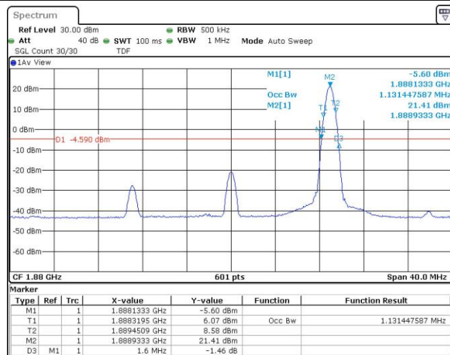
Band2-20MHz-16QAM-18900-1RB#99
