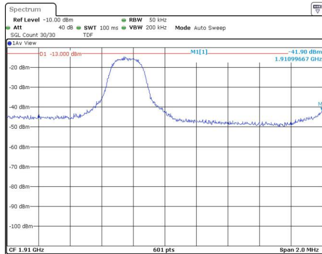
Band2-3MHz-QPSK-19185-1RB#14
