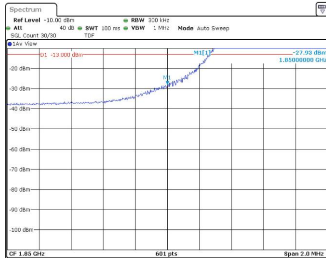
Band2-15MHz-QPSK-18675-1RB#74
