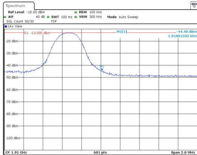
Band2-5MHz-QPSK-19175-1RB#24
