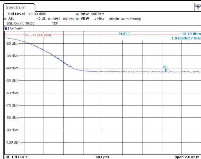
Band2-20MHz-QPSK-19100-1RB#99
