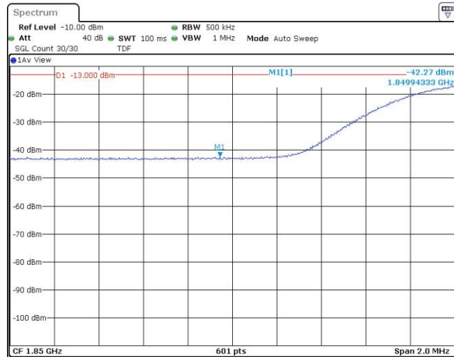
Band2-20MHz-QPSK-18700-100RB#0
