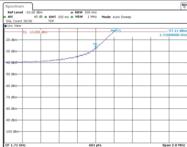
Band4-20MHz-QPSK-20050-1RB#99
