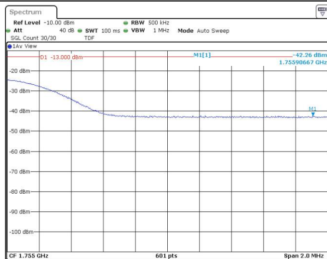
Band4-20MHz-QPSK-20300-1RB#99
