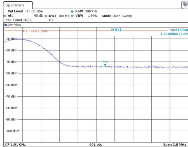
Band2-15MHz-16QAM-19125-1RB#74
