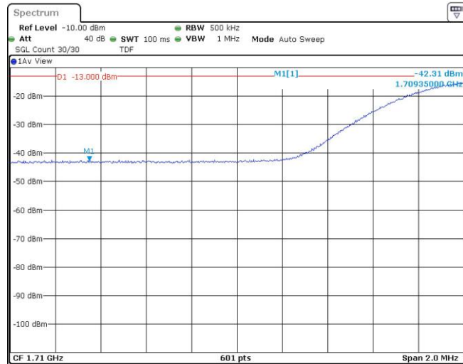
Band4-20MHz-QPSK-20050-100RB#0
