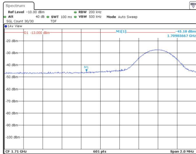
Band4-10MHz-QPSK-20000-50RB#0
