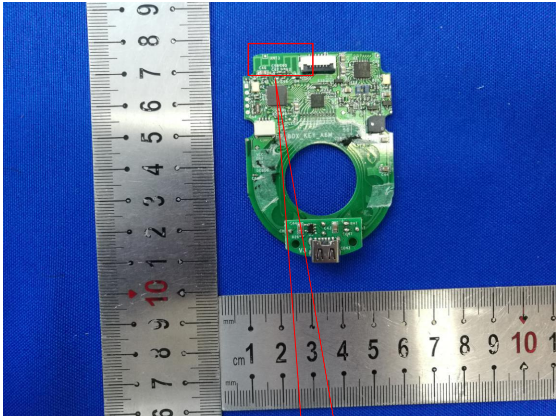
BLE Antenna
