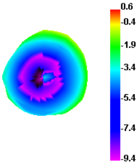
2400.000MHz E1
