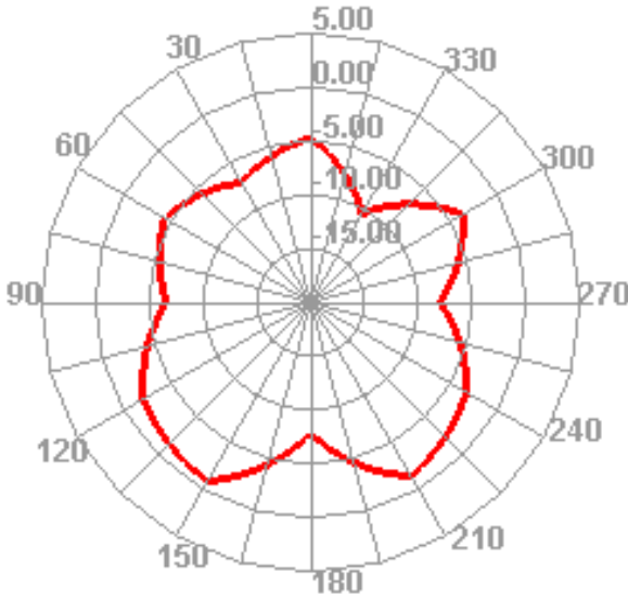
2400.000MHz E1
