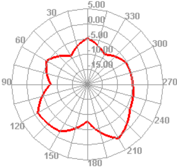
2400.000MHz E2
