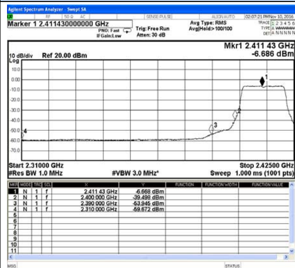
802.11n(HT20)-Low channel(Average)
