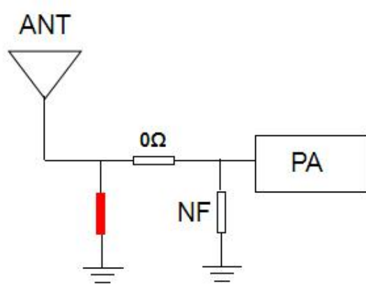
原始匹配电路未更改
