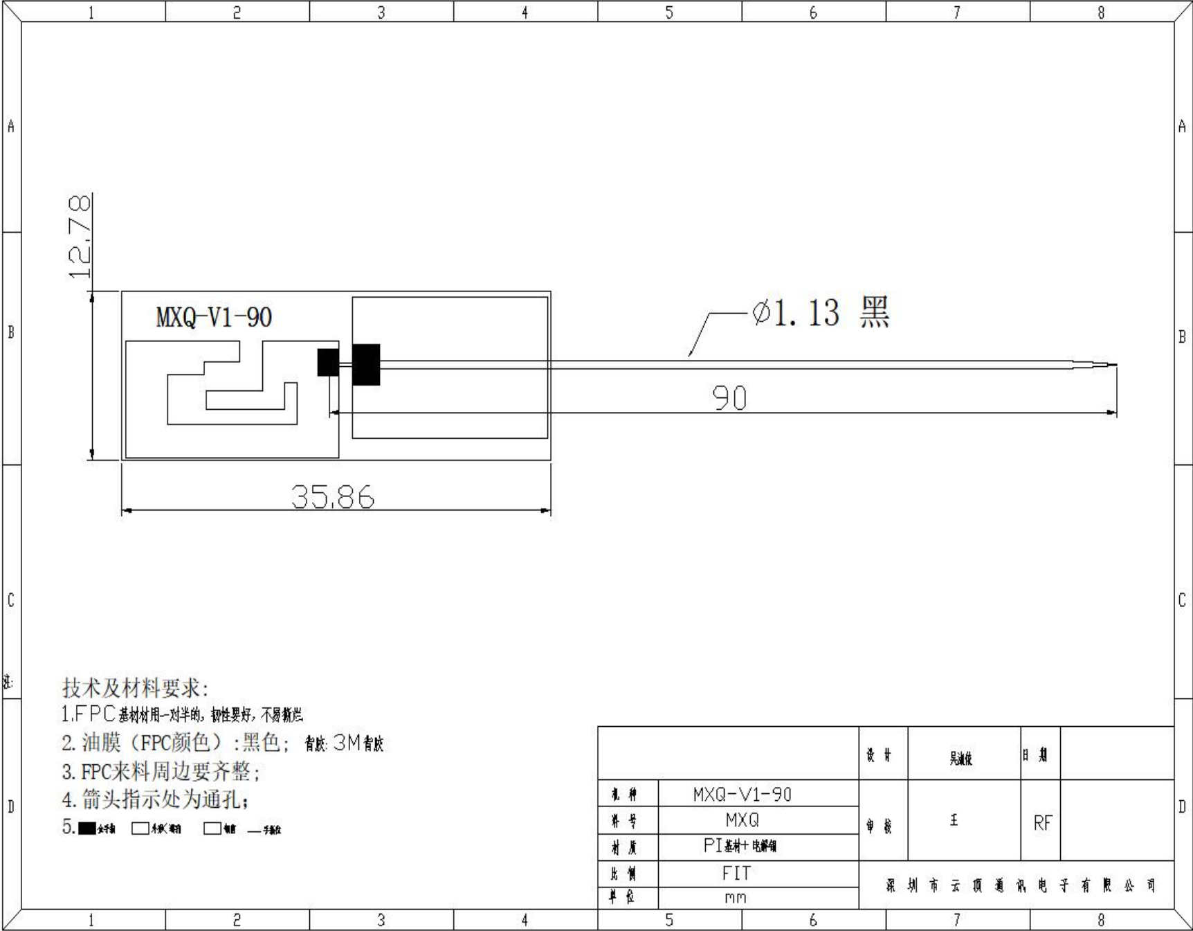
4.天线结构图
