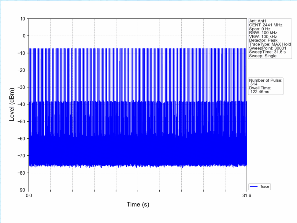
Pi/4DQPSK_2DH1_HOPP_Ant1_NTNV
