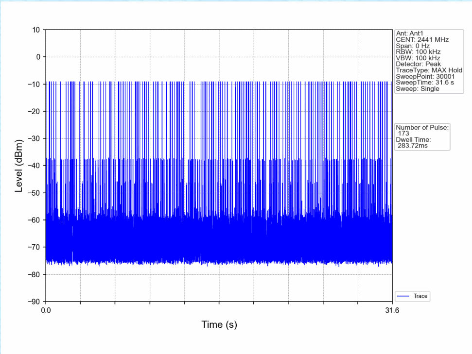
8DPSK_3DH3_HOPP_Ant1_NTNV
