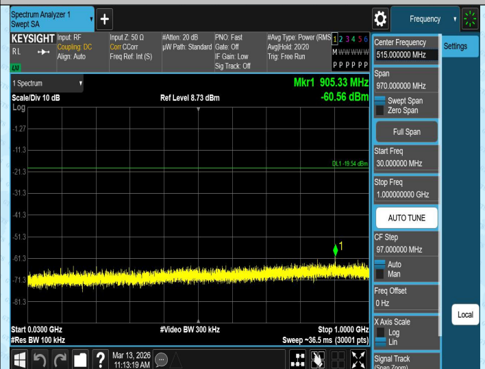
BLE_2M-Ant1-2440-30~1000-PASS
