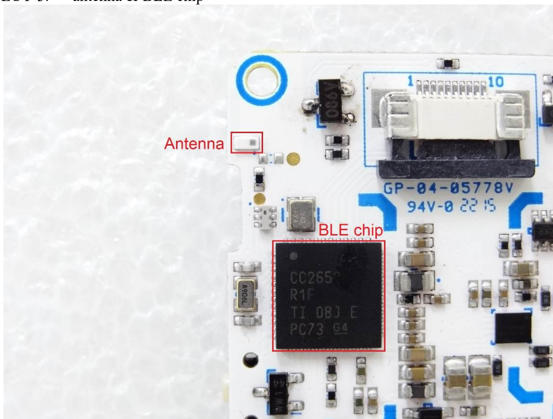
EUT-5. antenna & BLE chip
