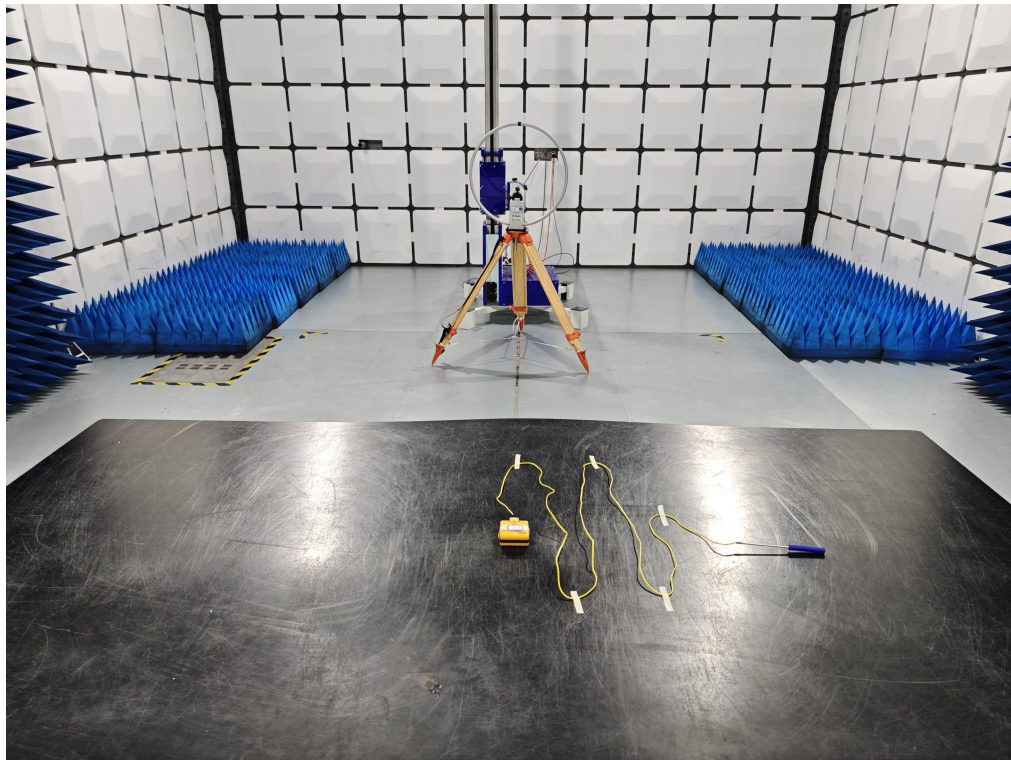
9kHz – 30MHz
