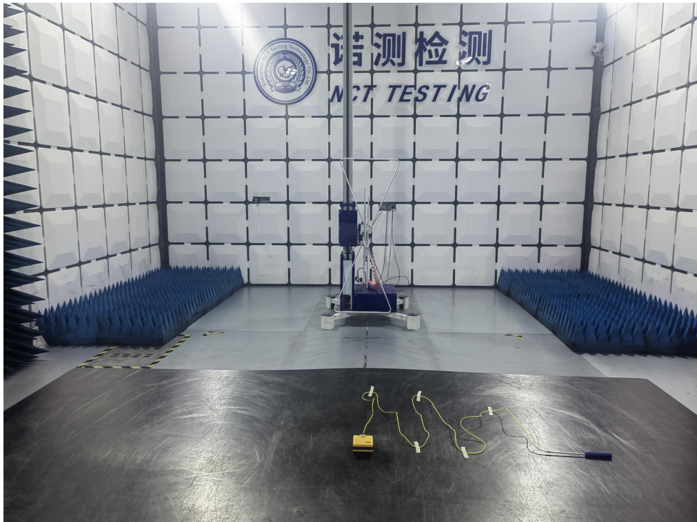
30MHz-1000MHz
