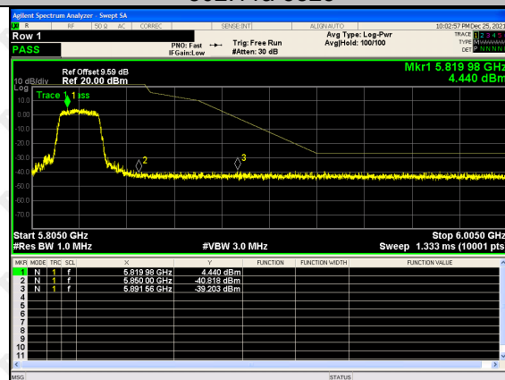
802.11(n20)-5825
