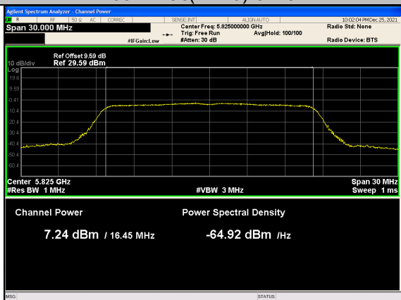
802.11ac(VH20)-5825
