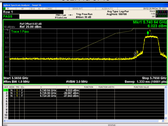
802.11(n20)-5745
