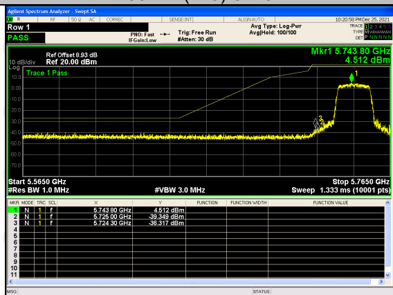
802.11(n40)-5755
