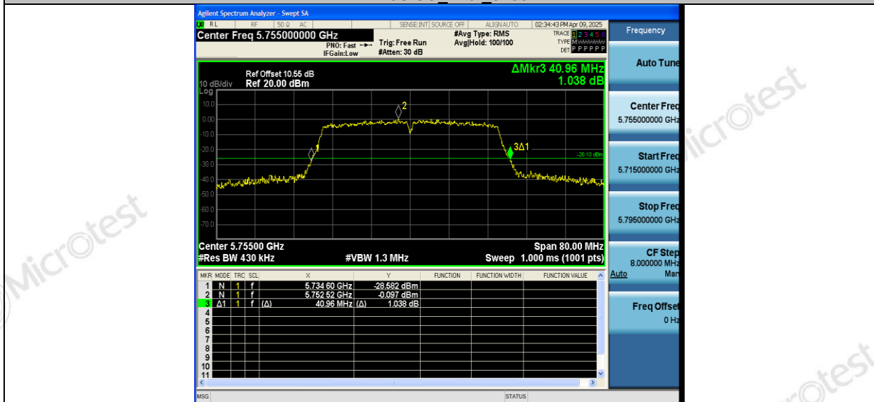
11N40SISO_Ant2_5755
