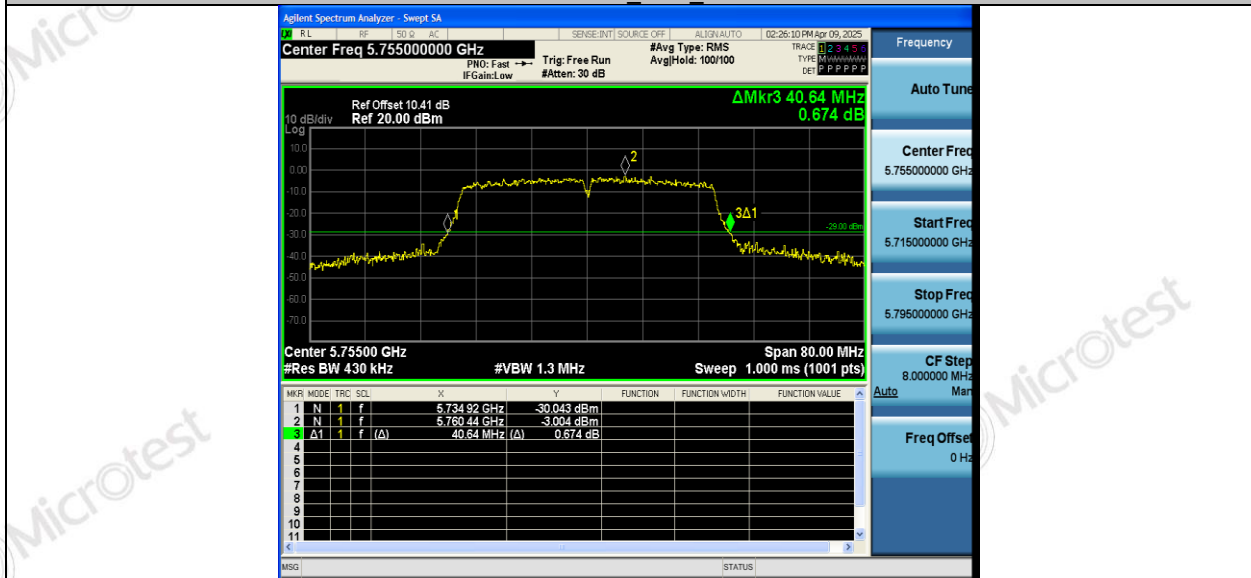
11N40SISO_Ant2_5755
