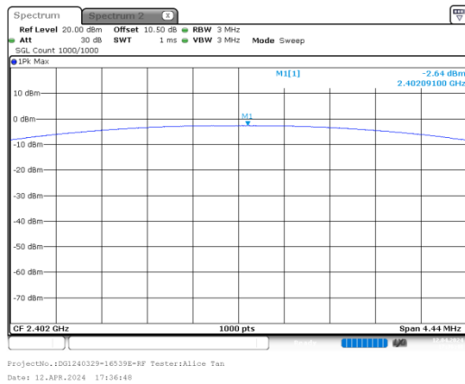
GFSK_Low_DH1
