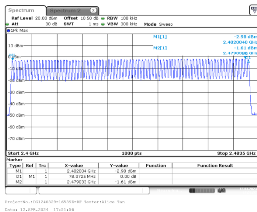
GFSK_Hopping_DH1
