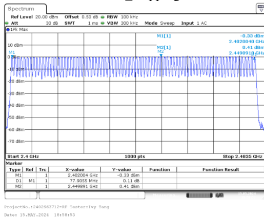
GFSK_Hopping
