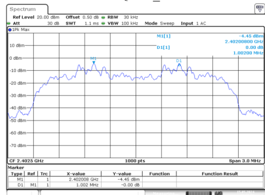
\pi/4 -DQPSK_Low
