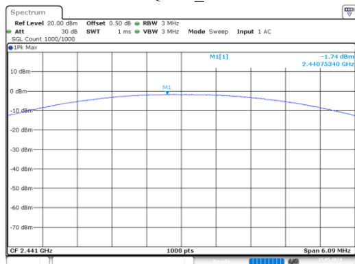
\pi/4 -DQPSK_Middle
