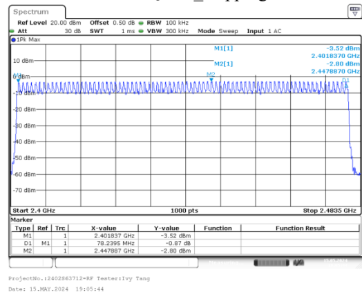
\pi/4 -DQPSK_Hopping
