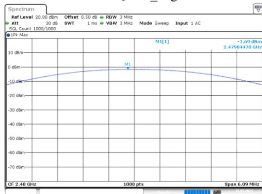
\pi/4 -DQPSK_High
