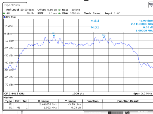
\pi/4 -DQPSK_Middle
