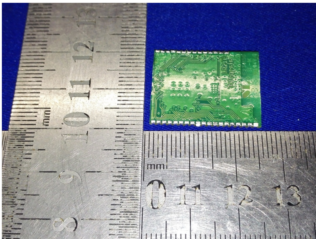
Zigbee Module
