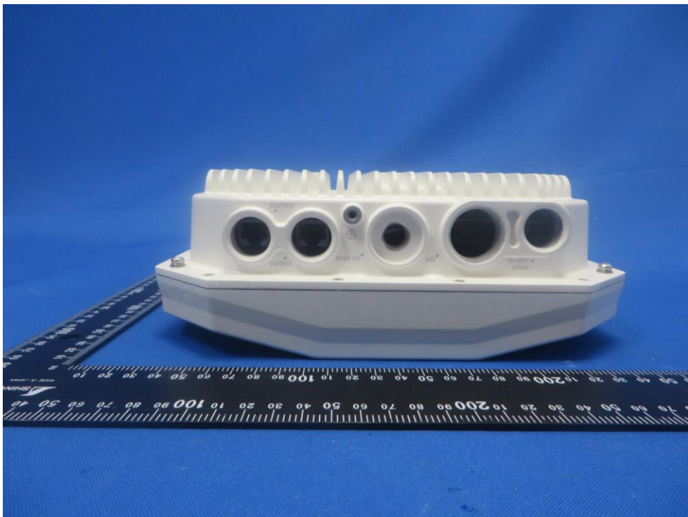
(4) EUT Photo - OAW-AP1361
