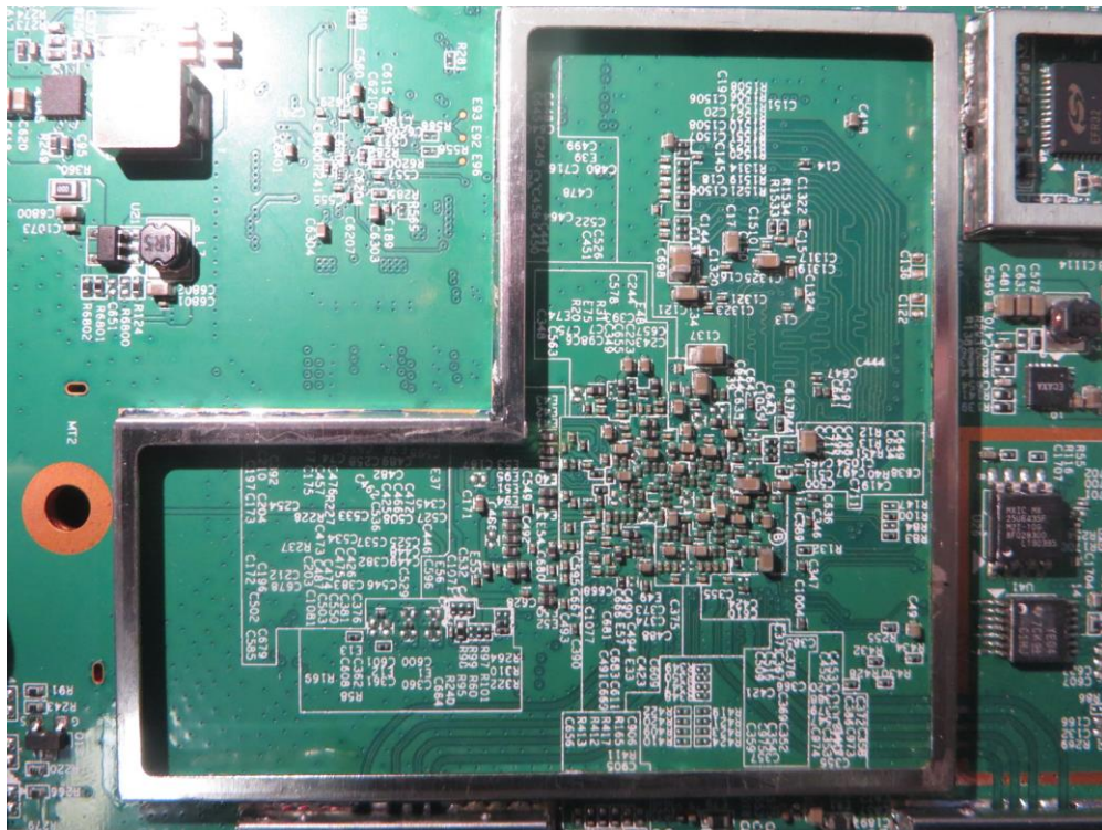
(33) EUT Photo
