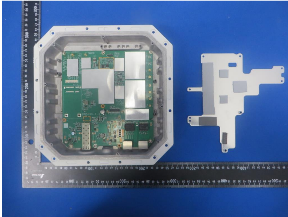
(9) EUT Photo - OAW-AP1362
