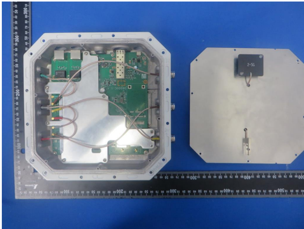
(7) EUT Photo - OAW-AP1362
