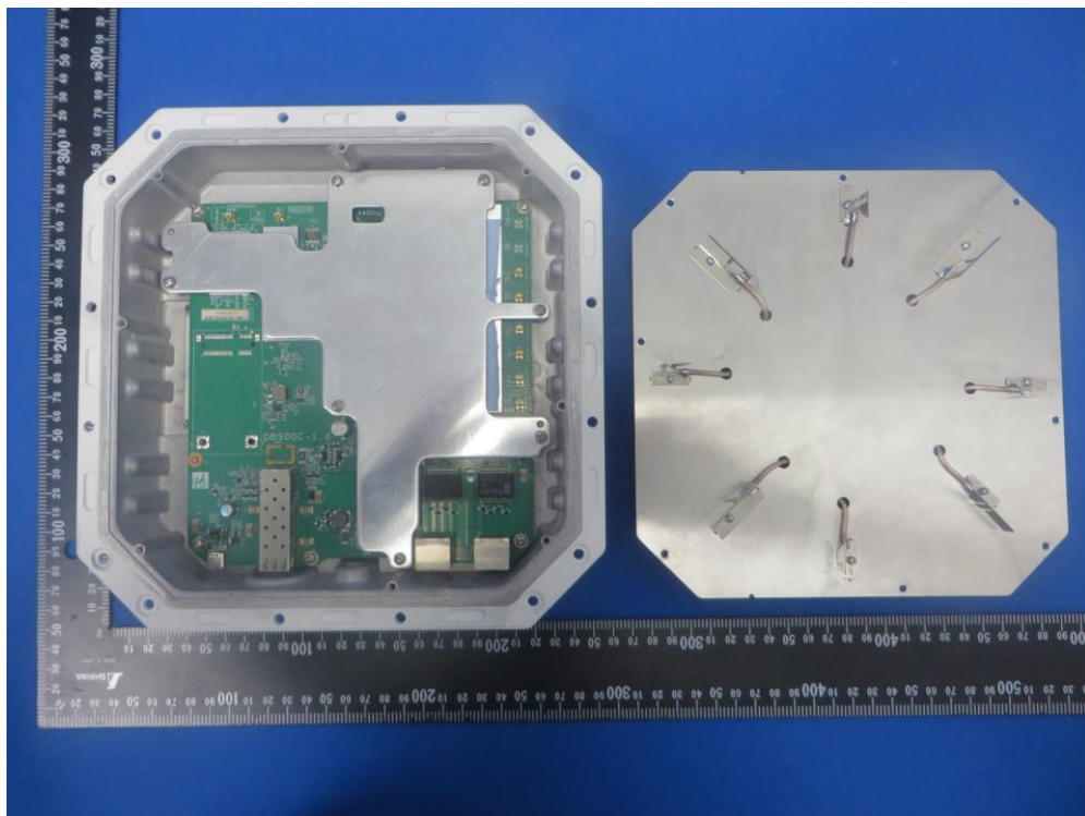
(2) EUT Photo - OAW-AP1361
