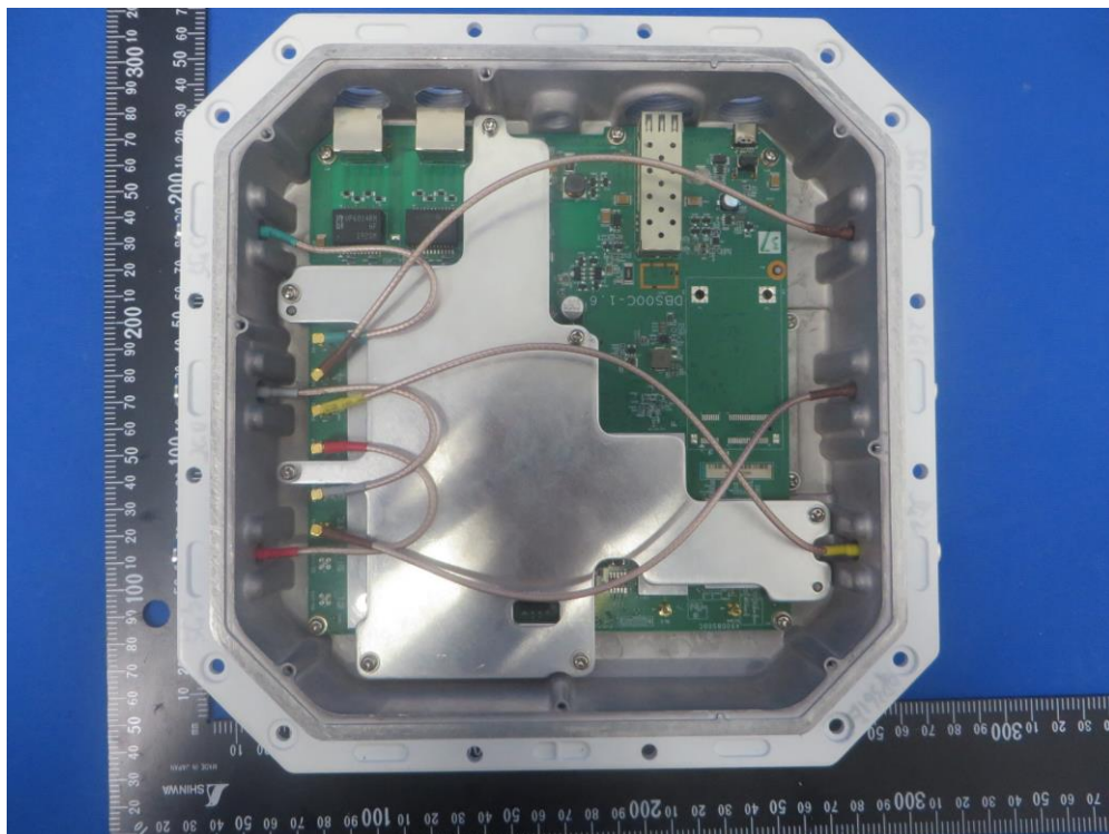
(8) EUT Photo - OAW-AP1362
