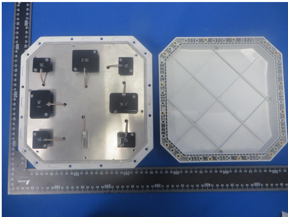
(4) EUT Photo - OAW-AP1361D
