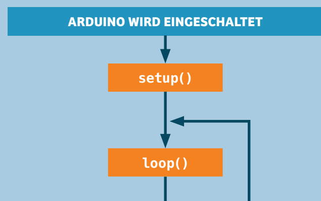
▲ Flussdiagramm
