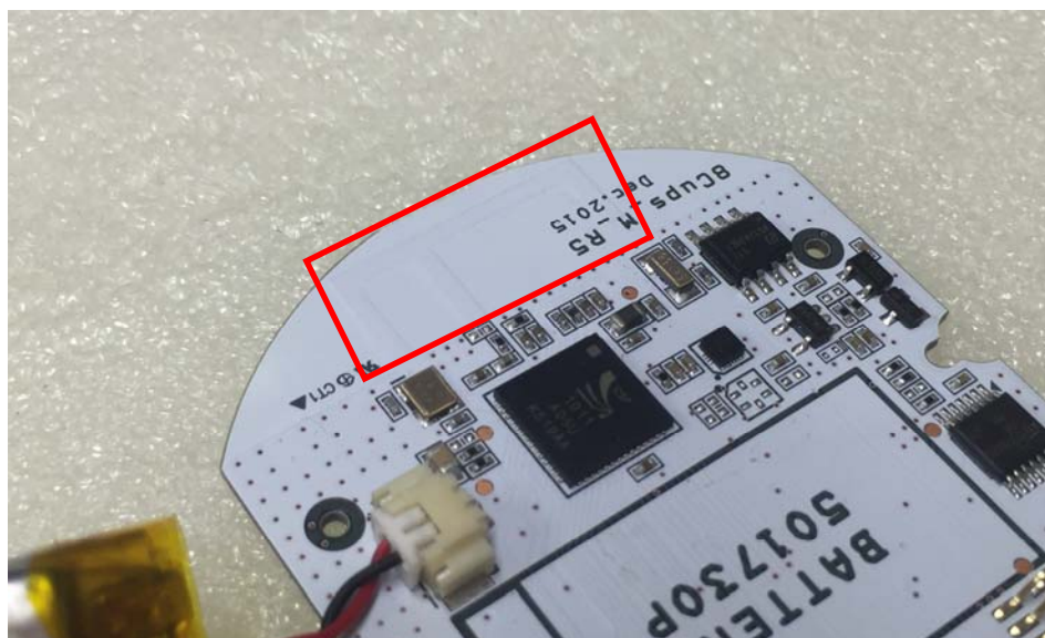
[BT Antenna]
