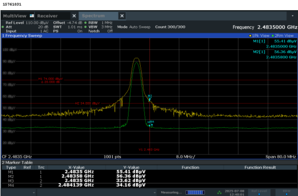
Upper Band Edge
