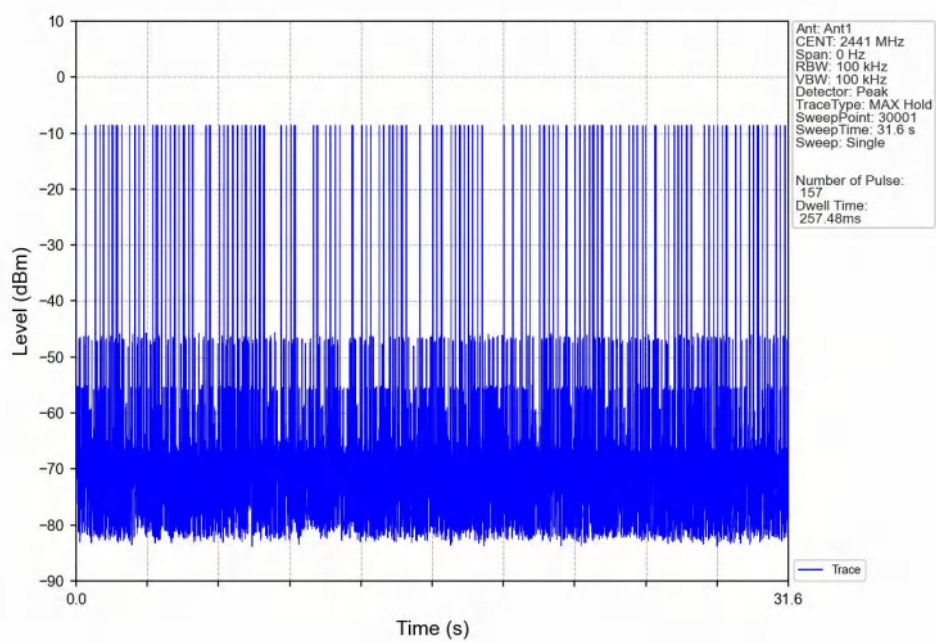
GFSK_DH3_HOPP_Ant1_NTNV
