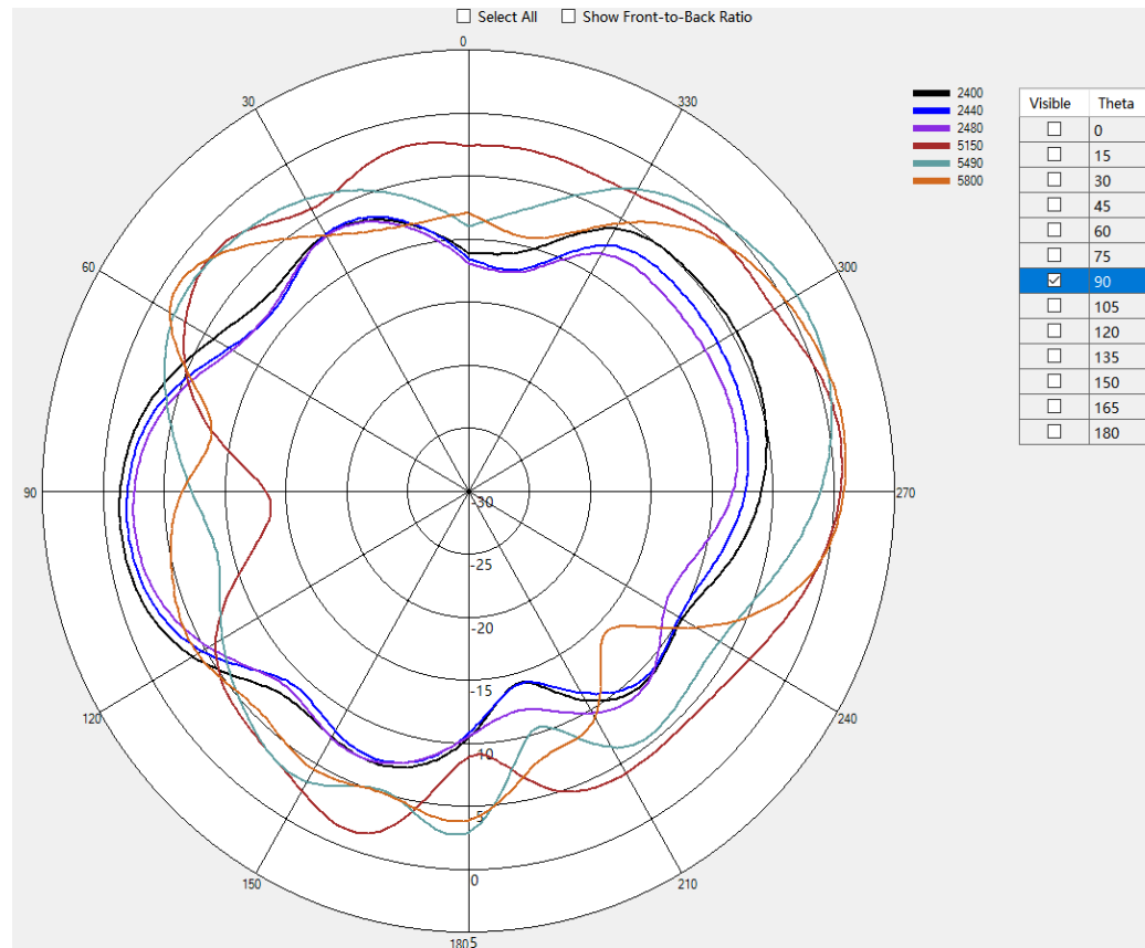
Ant2_2D_Theta90°
