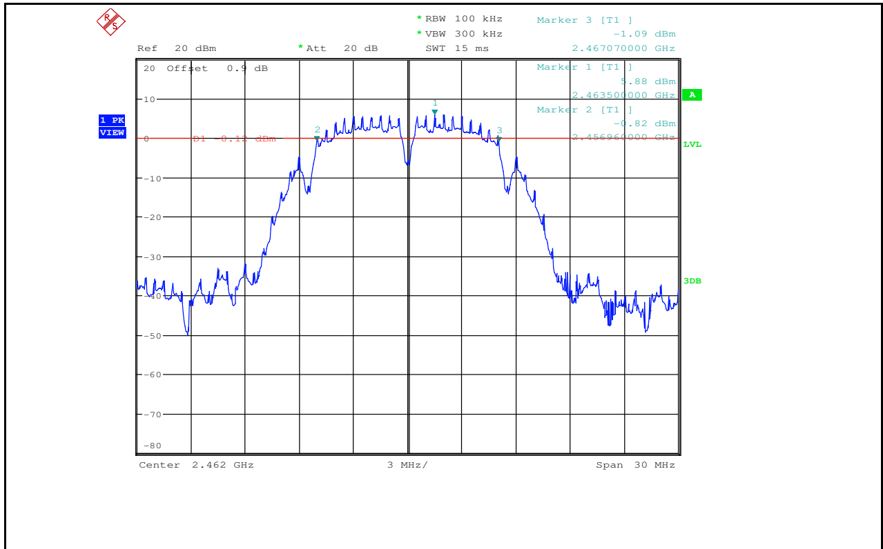
6dB Bandwidth_11B_2462_Ant2
