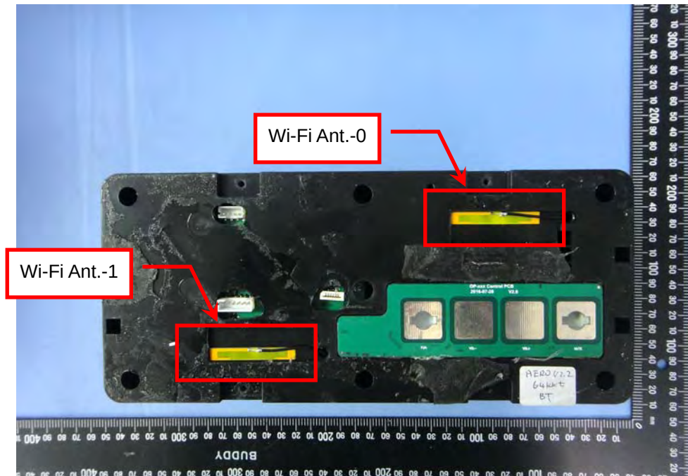
EUT Photo 3 )
