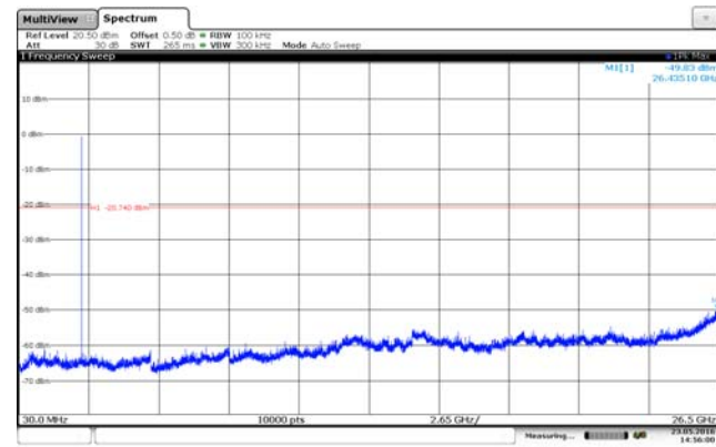
CH00
