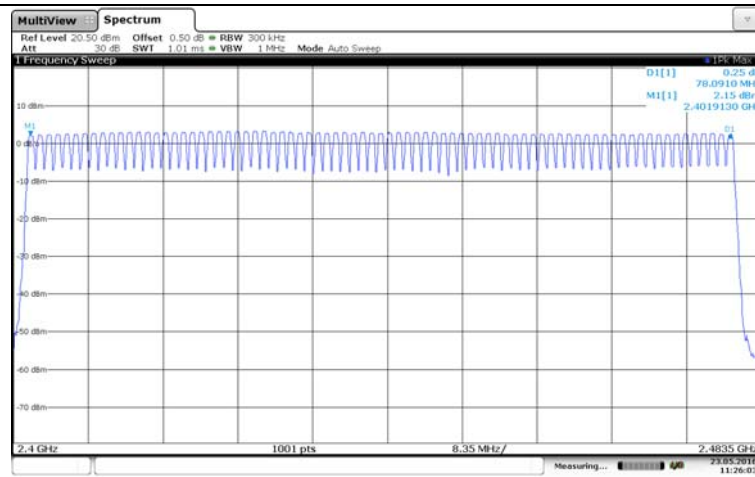
GFSK
