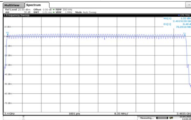
8DPSK
