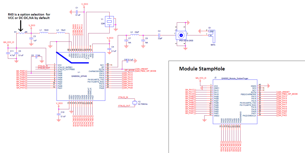
QN9080- QFN-Module
