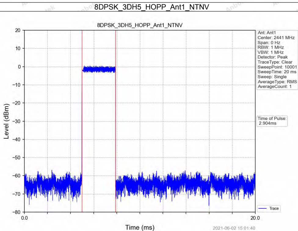
8DPSK_3DH5_HOPP_Ant1_NTNV
