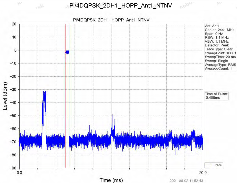
Pi/4DQPSK_2DH1_HOPP_Ant1_NTNV
