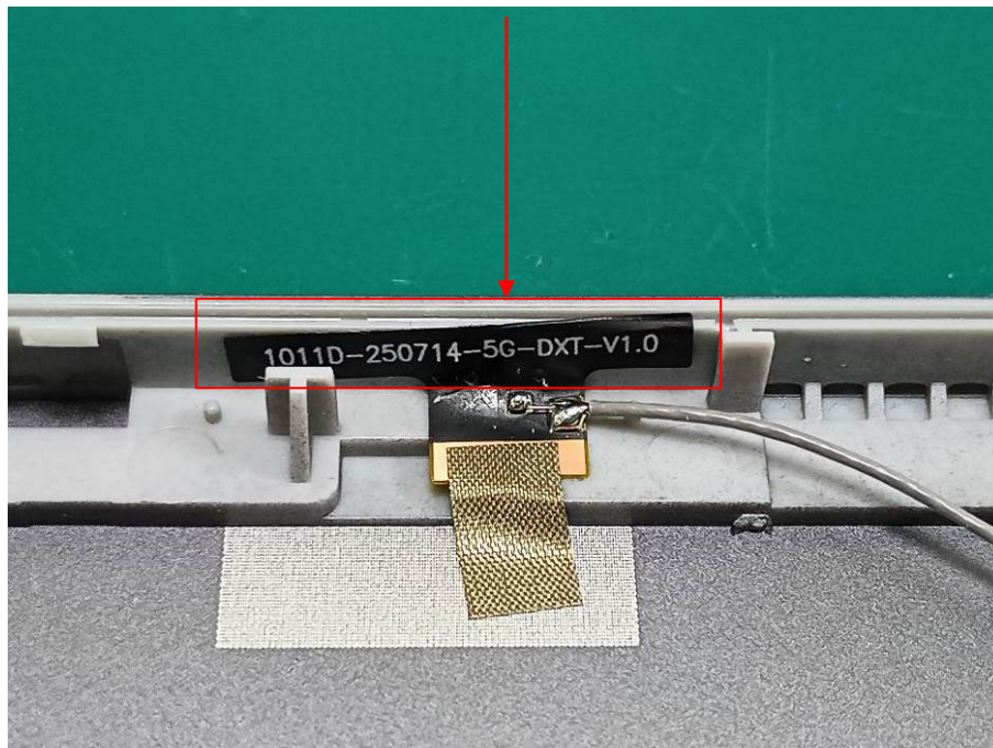
Wi-Fi ANT 1
